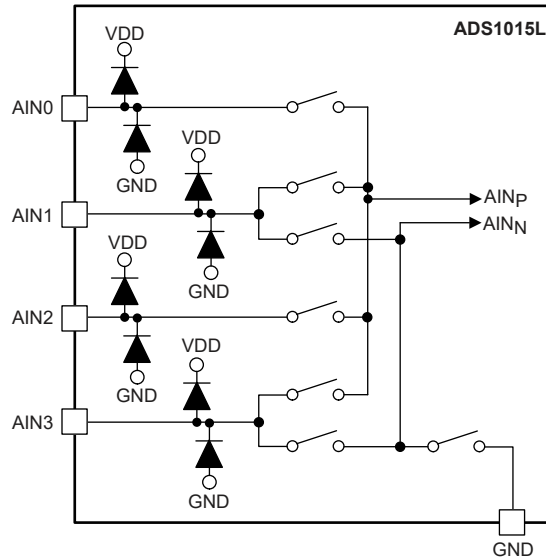
図 7-3. Input Multiplexer
