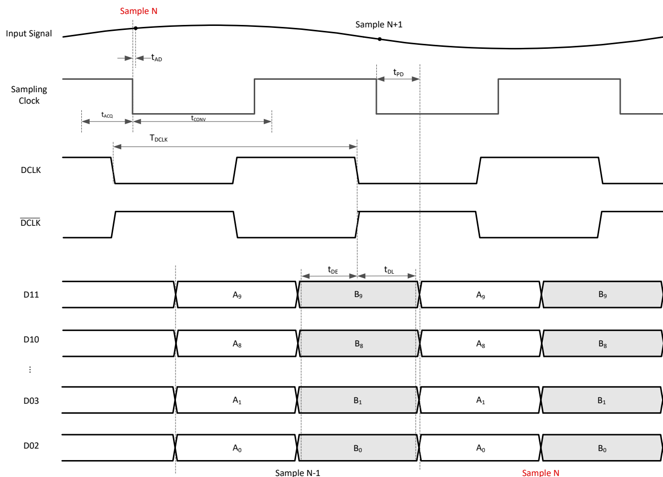
图 5-1. Timing Diagram: 10-Bit DDR (Default: 10 Lanes)
