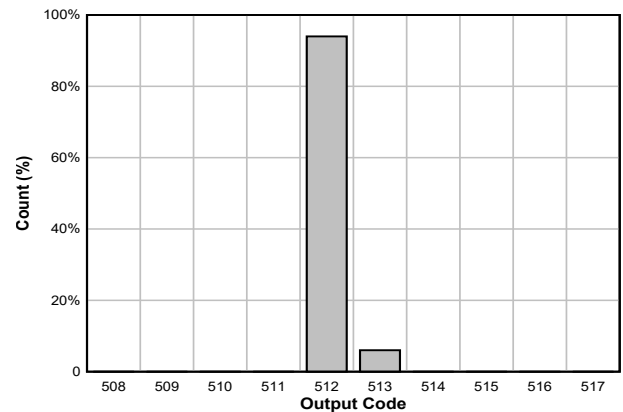
图 5-61. DC Offset Histogram
