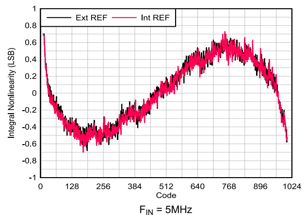
图 5-59. INL vs ADC Code
