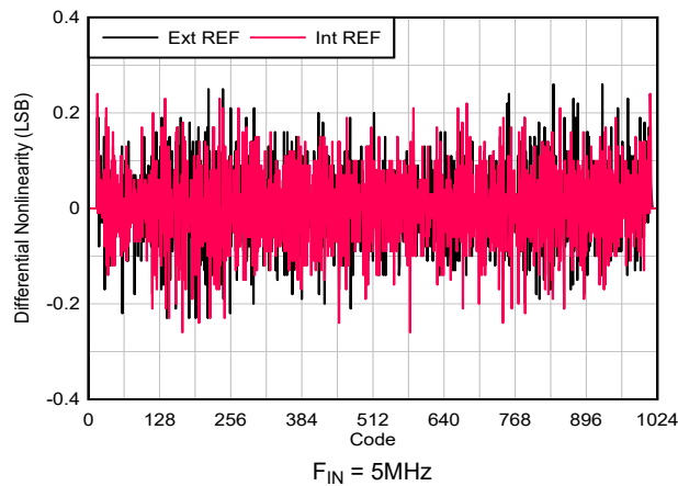
图 5-60. DNL vs ADC Code
