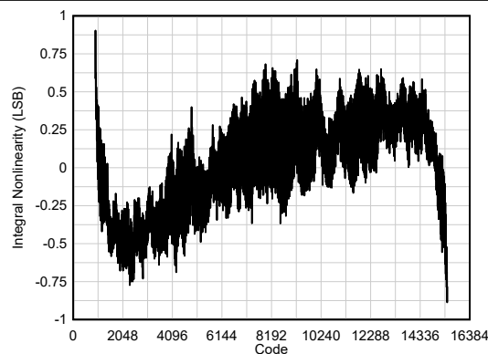
図 6-52. INL
