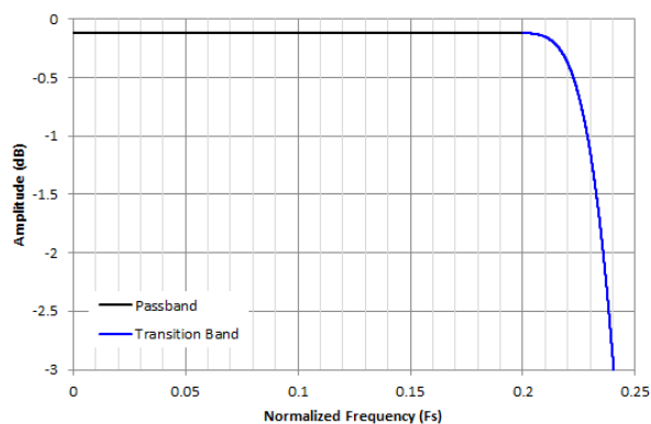
図 8-24. 1/2 デシメーションのパスバンド リップル 応答
