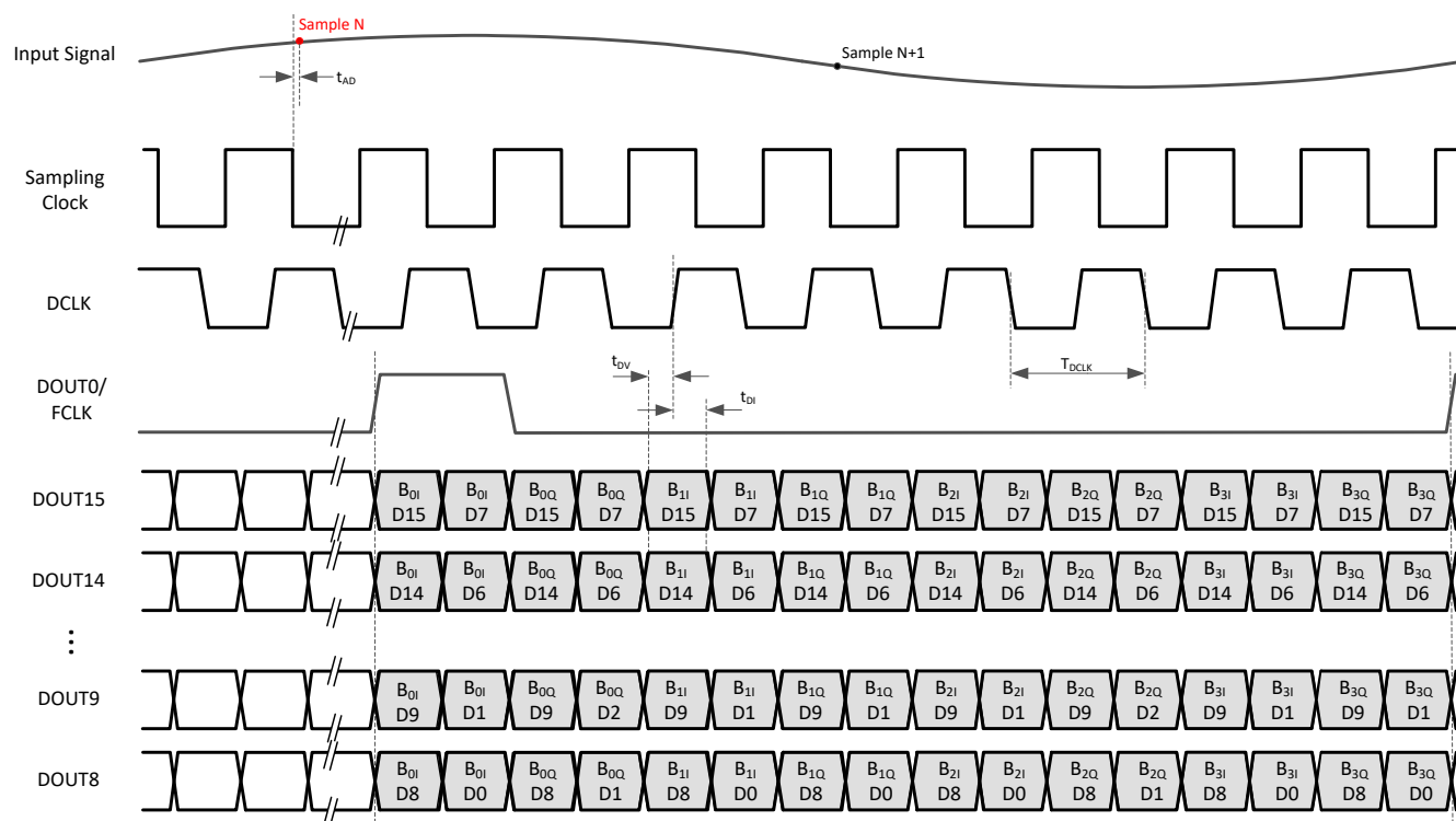
図 7-2. タイミング図 - シリアル LVDS (例: デュアルバンド、16 ビット、1/8 の複素デシメーション)
