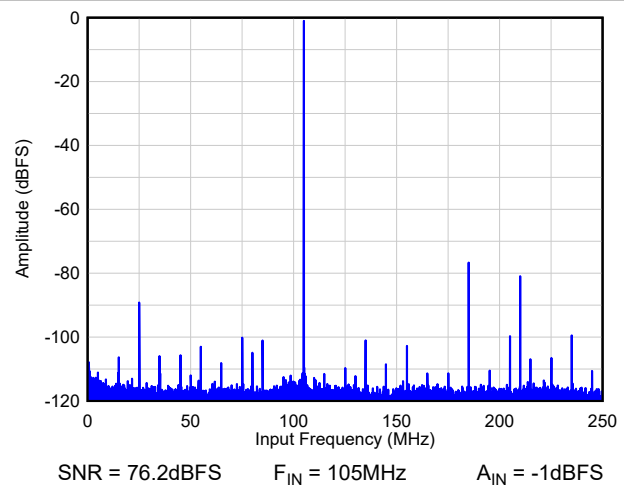
図 8-72. FFT - 2x AVG
