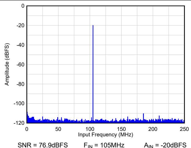
図 8-74. FFT - 2x AVG
