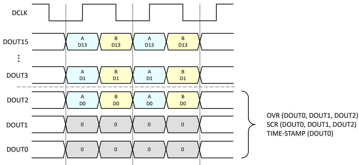
図 8-55. DDR LVDS モードでの出力データ フォーマット
