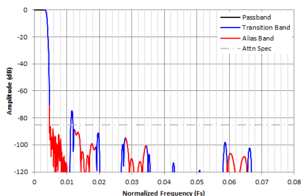
図 8-35. 1/128 複素デシメーションのフィルタ応答
