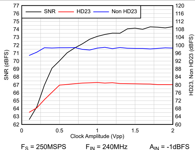
図 8-14. AC 振幅とクロック振幅との関係
