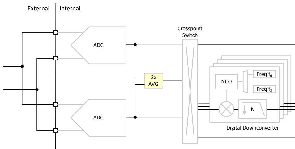
図 8-70. デジタル チャネル平均化の図
