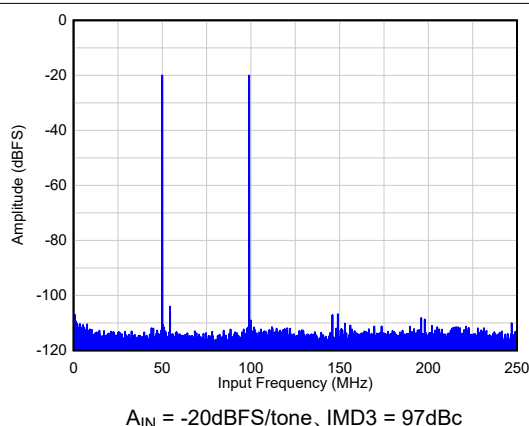
図 6-39. F_{IN} = 445/455\text{MHz} での 2 トーン FFT
