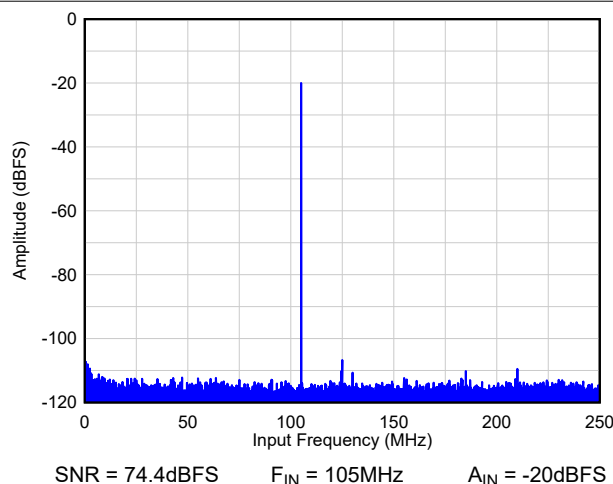
図 8-73. FFT - AVG なし
