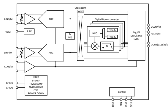
ブロック図
