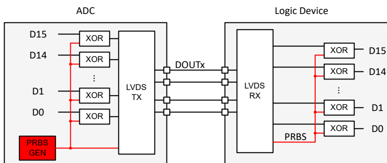
図 8-63. 出力スクランブラ
