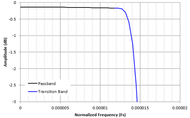
図 8-52. 1/32768 デシメーションのパスバンド リップル応答
