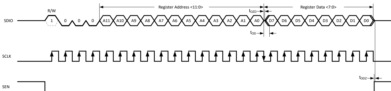
図 8-76. シリアル レジスタ読み出しタイミング図
