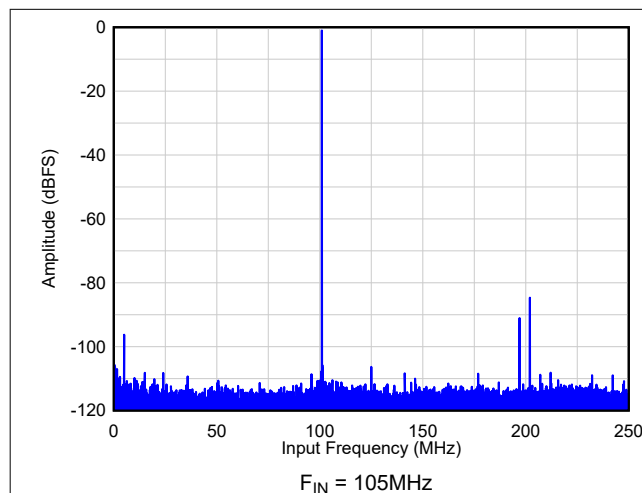
図 8-68. FFT : 通常モード
