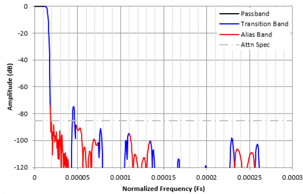
図 8-51. 1/32768 複素デシメーションのフィルタ応答
