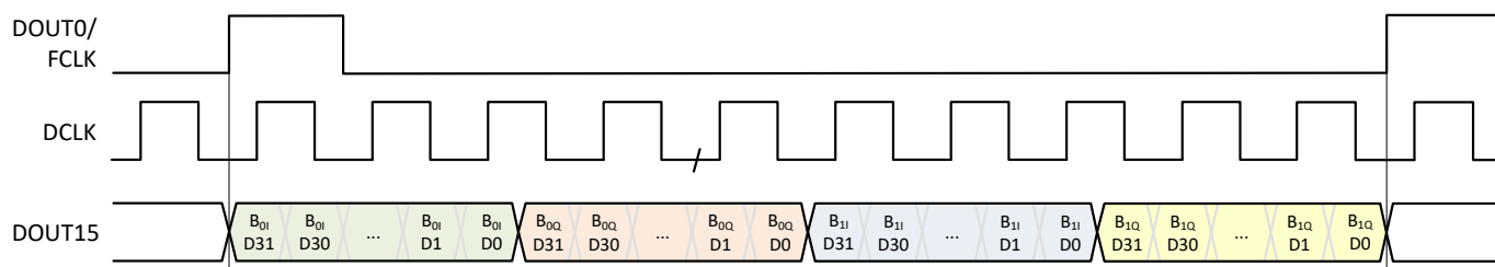
図 8-60. 例 5 の SLVDS フレームの組み立て
