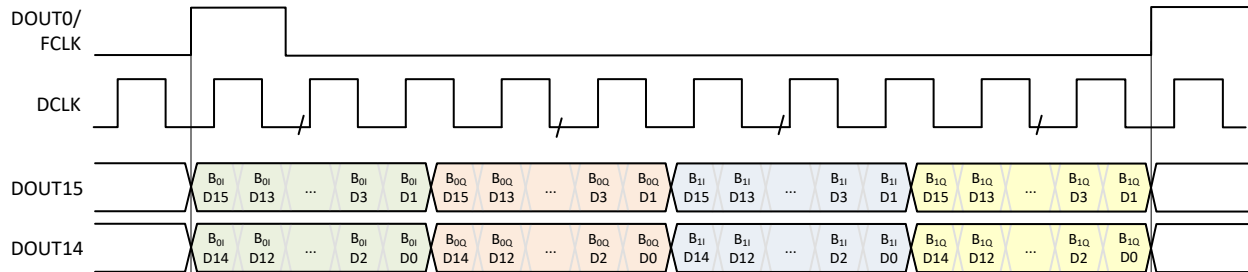
図 8-58. 例 3 の SLVDS フレームの組み立て
