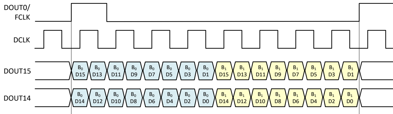
図 8-56. 例 1 の SLVDS フレームの組み立て
