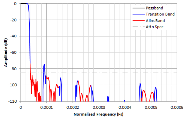
図 8-49. 1/16384 複素デシメーションのフィルタ応答
