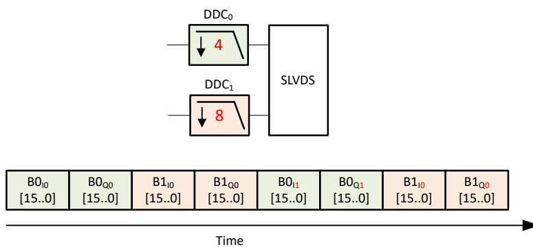
図 8-21. 異なるデシメーション係数
