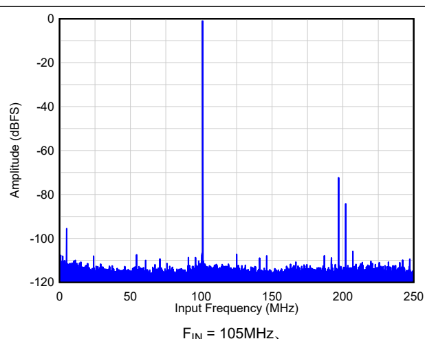
図 8-69. FFT : 低レイテンシ モード
