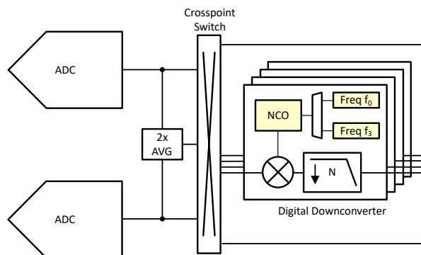
図 8-53. NCO のブロック図
