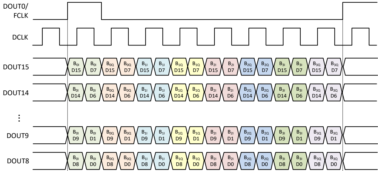
図 8-59. 例 4 の SLVDS フレームの組み立て
