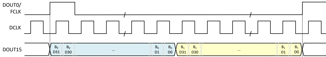
図 8-57. 例 2 の SLVDS フレームの組み立て
