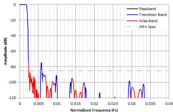
図 8-37. 1/256 複素デシメーションのフィルタ応答
