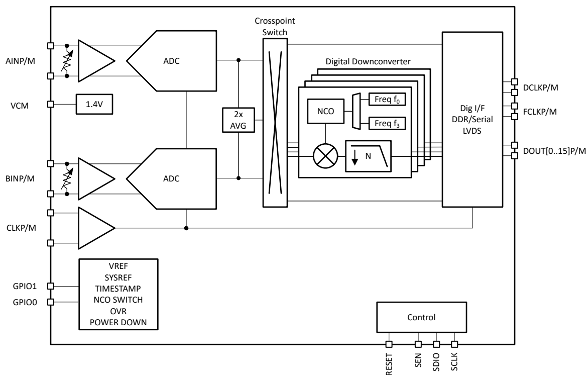
図 8-1. ブロック図
