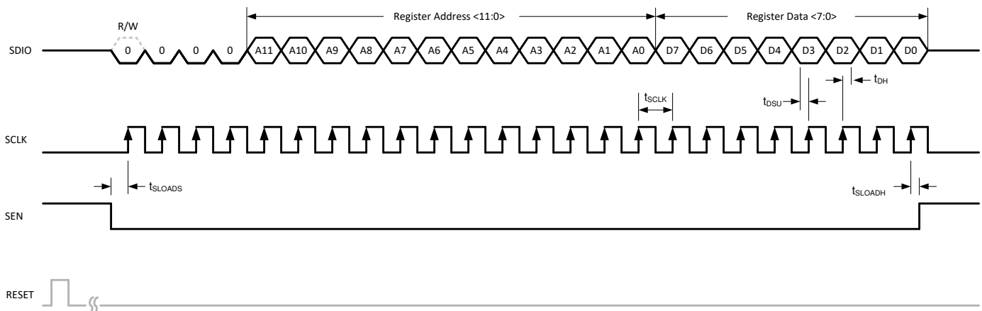
図 8-75. シリアル レジスタ書き込みタイミング図
