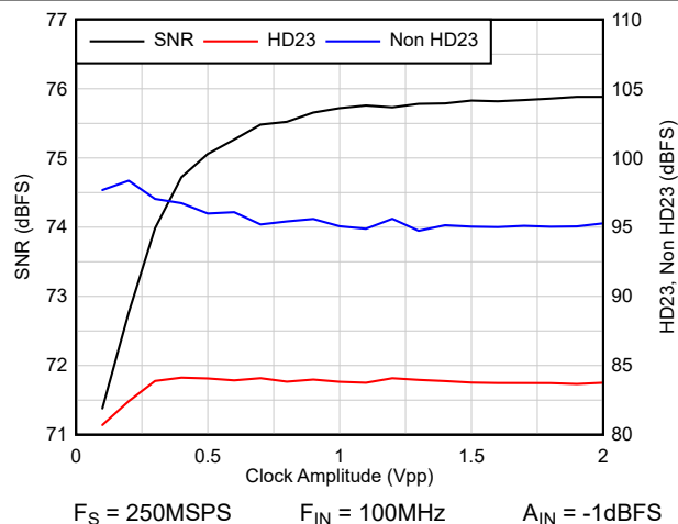
図 8-13. AC 振幅とクロック振幅との関係
