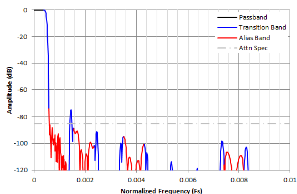
図 8-41. 1/1024 複素デシメーションのフィルタ応答
