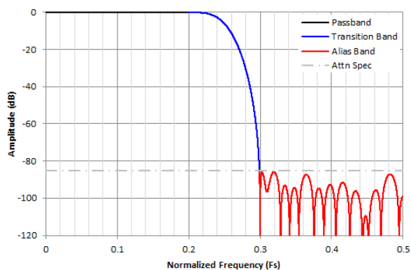
図 8-23. 1/2 複素デシメーションのフィルタ 応答
