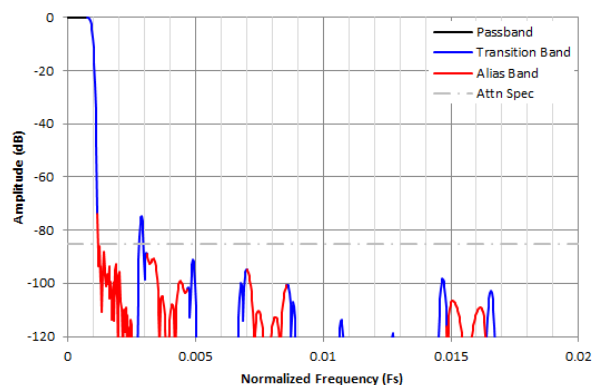
図 8-39. 1/512 複素デシメーションのフィルタ応答
