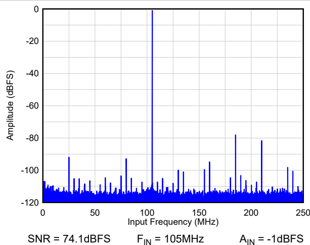
図 8-71. FFT - AVG なし
