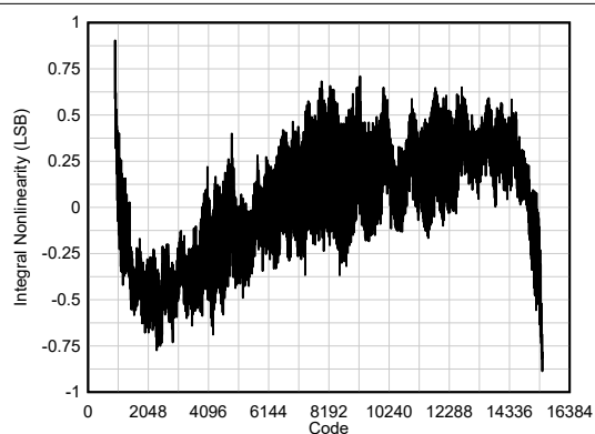
図 6-51. INL
