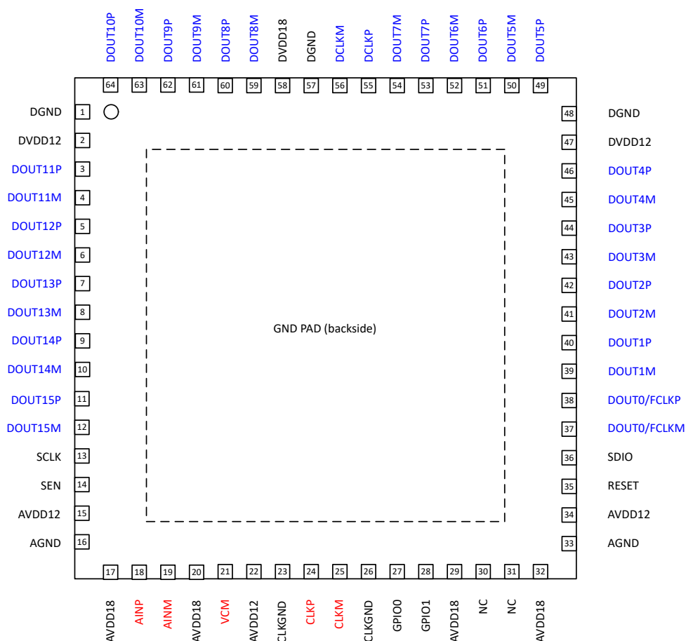
図 5-1. RTD パッケージ、64 ピン VQFN (上面図)
