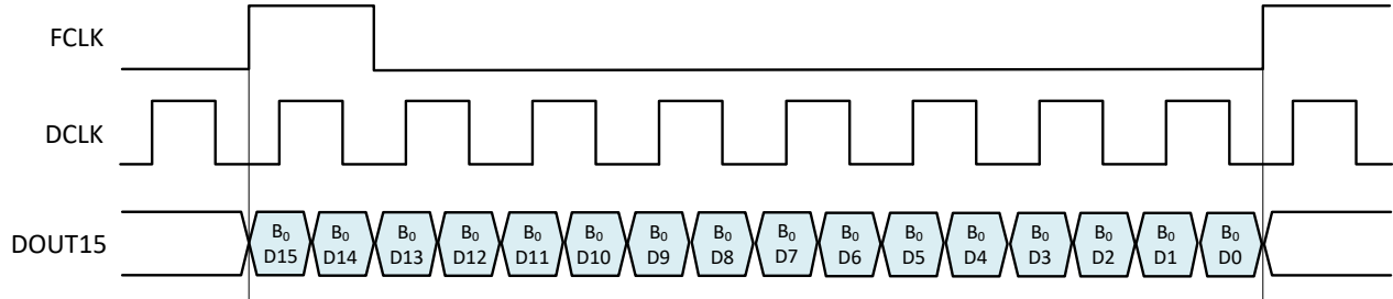
図 8-57. 例 1 の SLVDS フレームの組み立て
