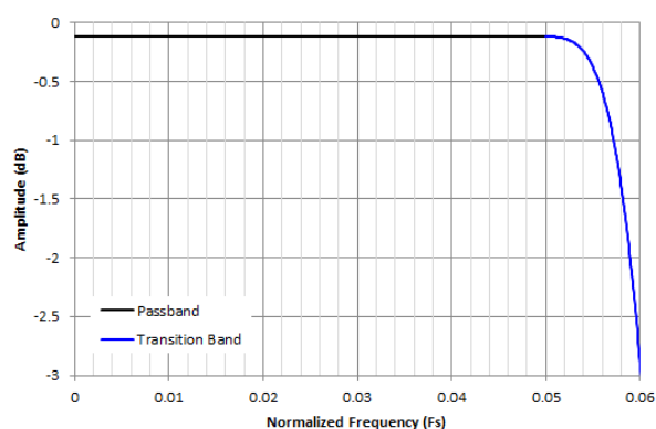
図 8-28. 1/8 デシメーションのパスバンド リップル応答
