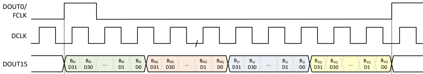
図 8-60. 例 4 の SLVDS フレームの組み立て
