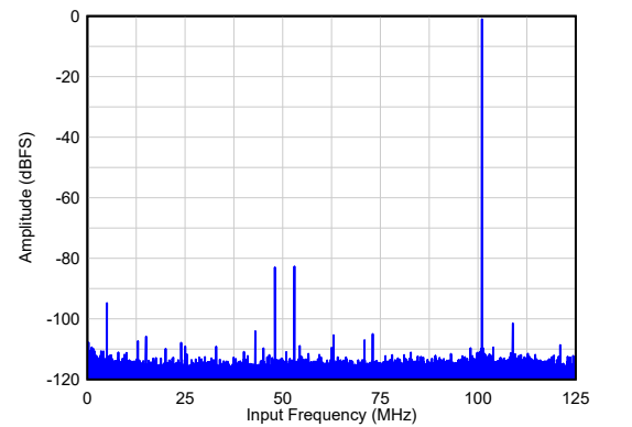
図 6-2. F_{IN} = 101\text{MHz} でのシングル トーン FFT
