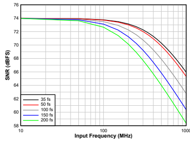
図 9-2. SNR と T_{\text{jitter}} と F_{\text{IN}} との関係
