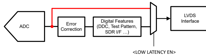
図 8-67. 低レイテンシ モード
