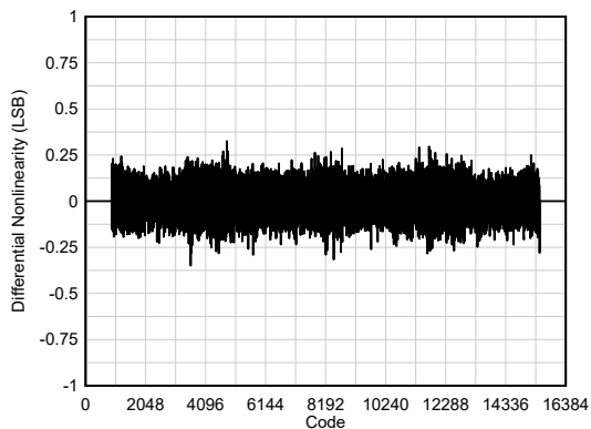
図 6-23. DNL
