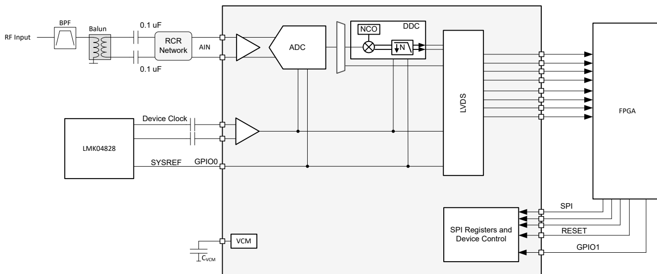
図 9-1. 広帯域スペクトラム アナライザの標準的な構成
