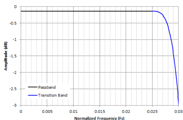
図 8-30. 1/16 デシメーションのパスバンド リップル応答
