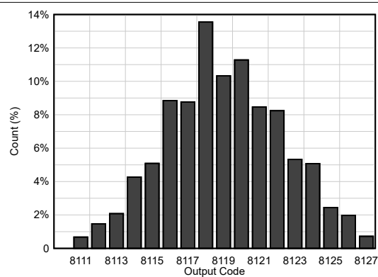
図 6-52. DC オフセット ヒストグラム
