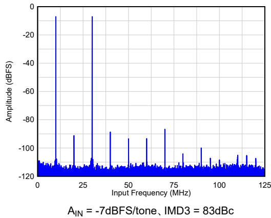
図 6-11. F_{IN} = 220/240\text{MHz} での 2 トーン FFT
