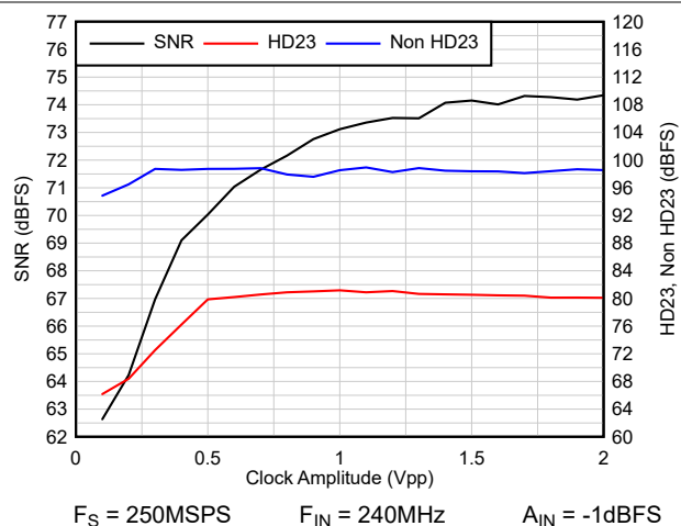
図 8-14. AC 振幅とクロック振幅との関係
