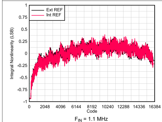
6-11. INL vs Code
