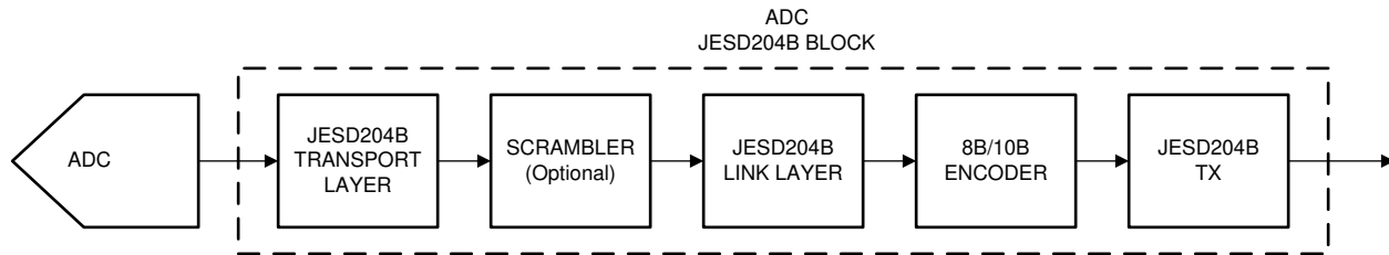
図 6-41. JESD204B Block Diagram
