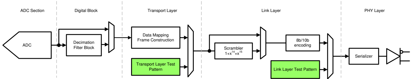
図 6-44. Test Pattern Options
