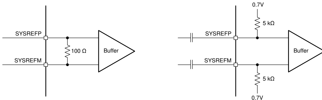
図 6-20. SYSREF Input Circuitry
