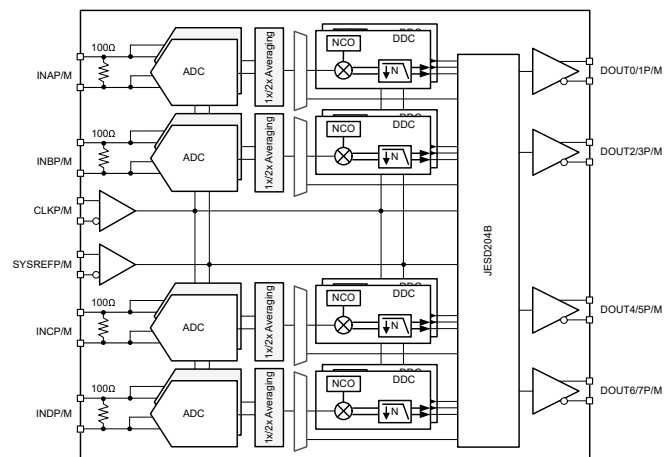
ブロック図
