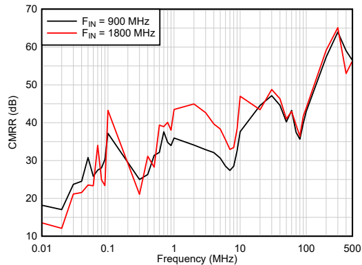
FIG 5-41. CMRR
