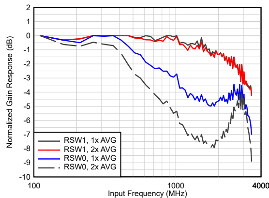
図 6-2. Input Bandwidth - Reset switch DIS
