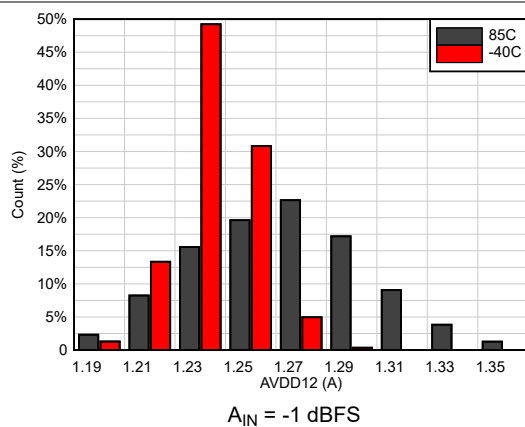
图 6-55. AVDD12 Distribution
