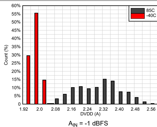
图 6-56. DVDD Distribution
