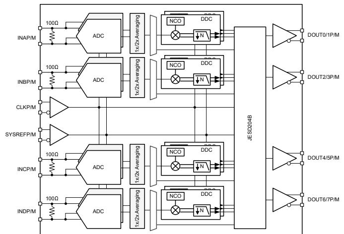
ブロック図
