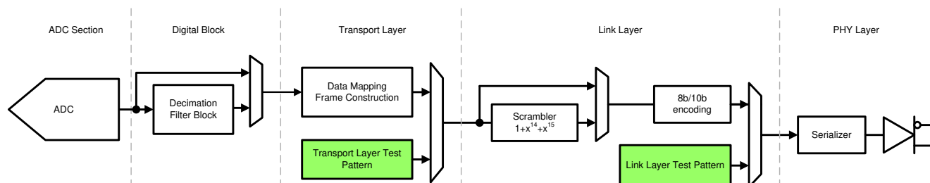
図 7-41. Test Pattern Options
