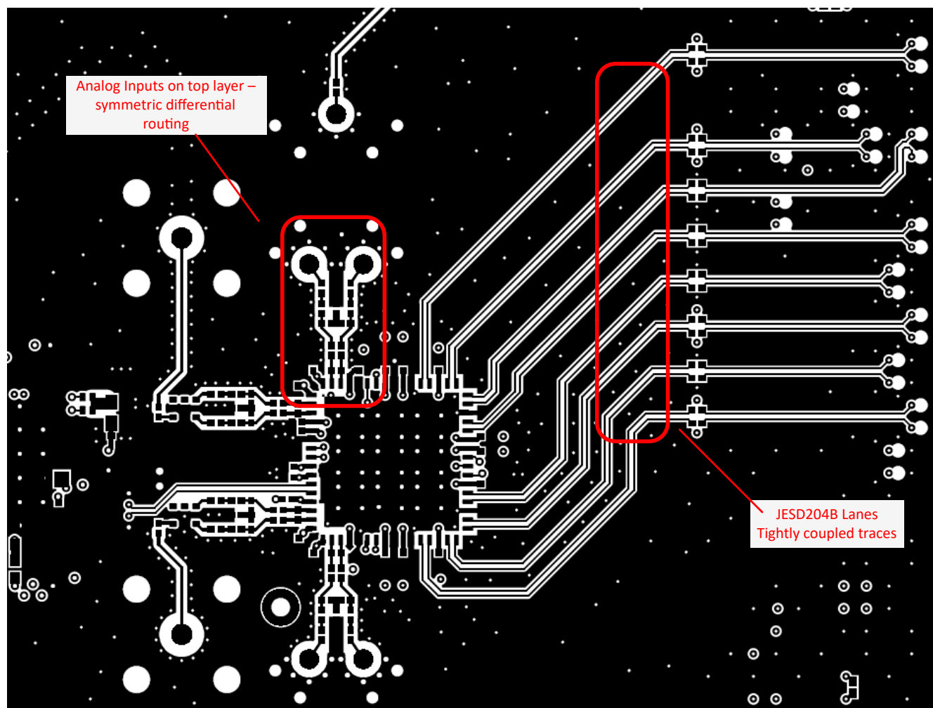
図 8-7. Layout example: top layer of ADC32RF5x EVM
