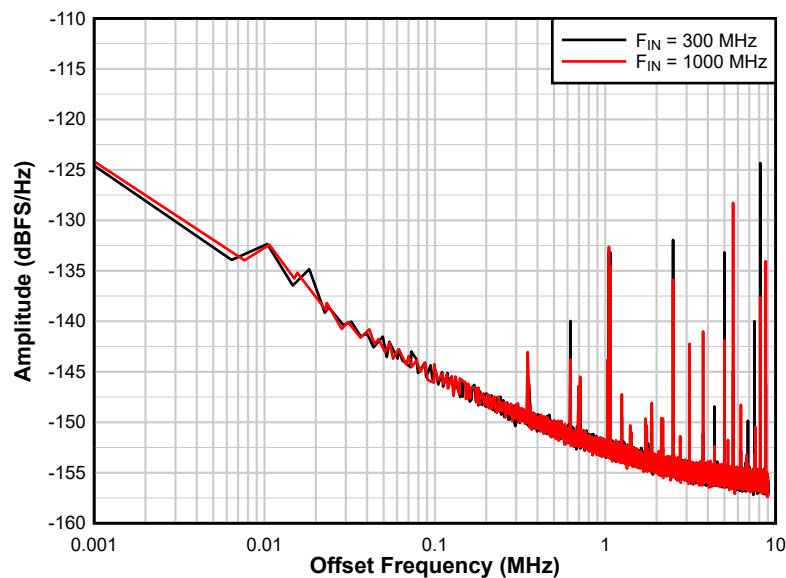
図 7-8. Amplitude Noise
