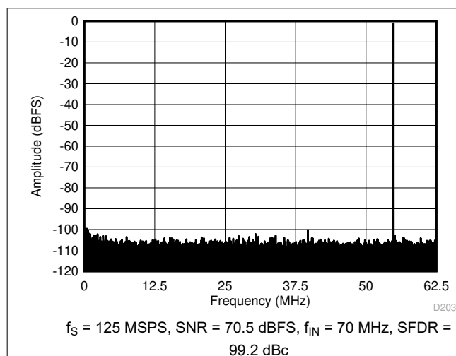
图 8-11. FFT with Dither On
