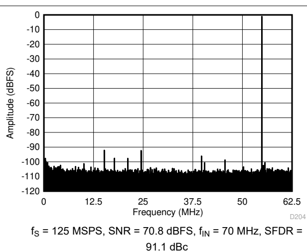
图 8-12. FFT Dither Off
