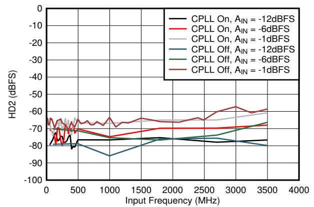
図 6-52. HD2 vs A_{IN} and C-PLL
