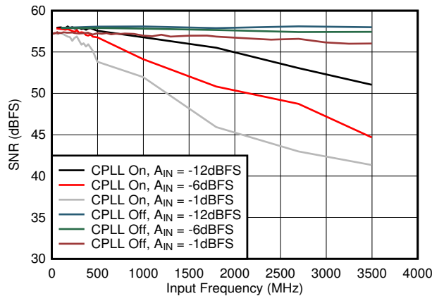
図 6-49. SNR vs A_{IN} and C-PLL
