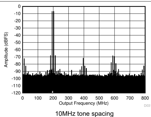
図 5-70. Two Tone FFT at 1798MHz
