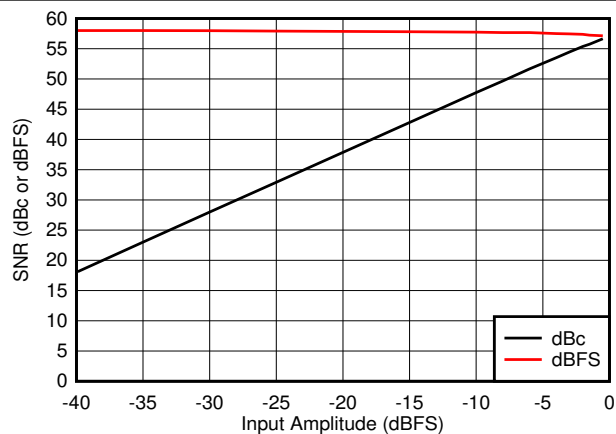
図 5-35. SNR vs A_{IN}
