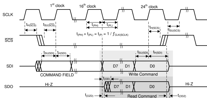
図 5-9. Serial Interface Timing
