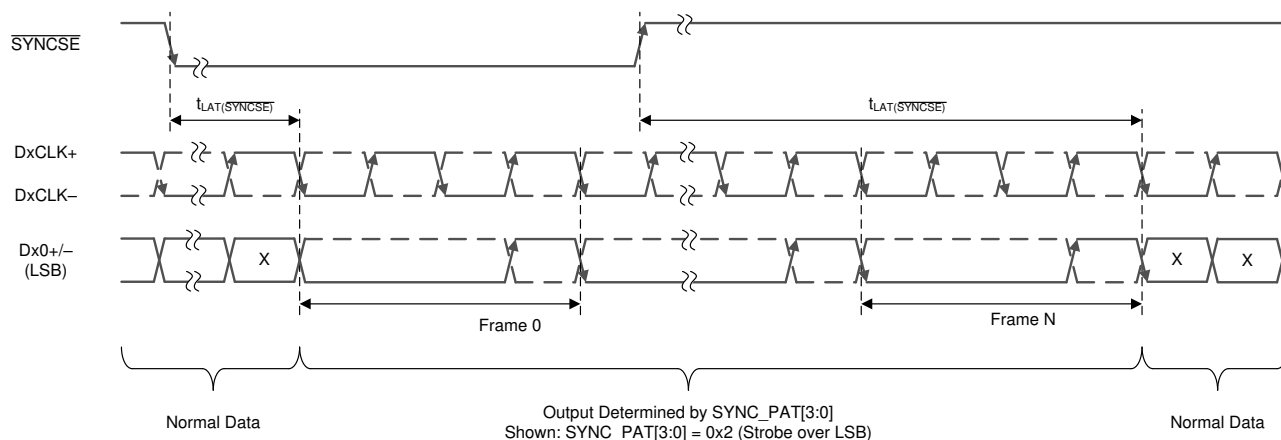
図 5-8. SYNCSE Timing Diagram
