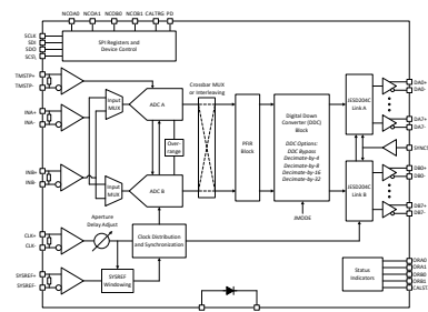
ADC12DJ5200RF ブロック図
