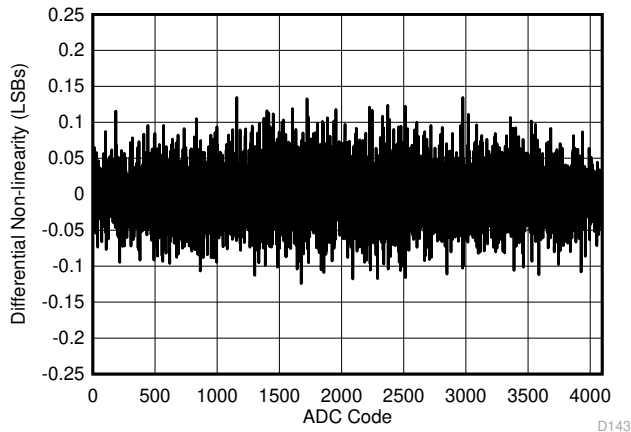
図 5-3. DNL vs ADC Code
