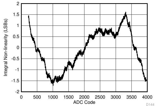
図 5-4. INL vs ADC Code
