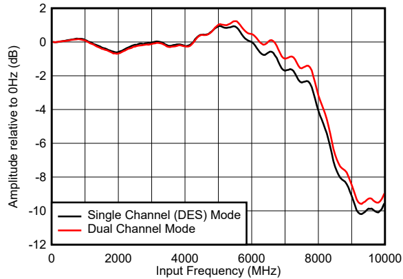
図 5-1. Input Amplitude vs Input Frequency
