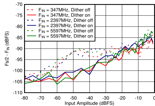
図 5-82. デュアル チャネル モード : F_{\text{s}}/2 - F_{\text{IN}} と入力振幅およびディザとの関係
