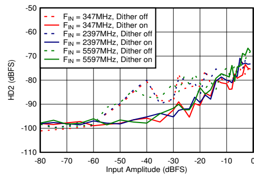
図 5-78. デュアル チャネル モード : HD2 と入力振幅およびディザとの関係
