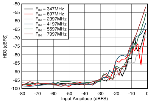
図 5-79. デュアル チャネル モード : HD3 と入力振幅および周波数との関係
