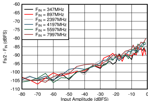
図 5-81. デュアル チャネル モード : F_{\text{s}}/2 - F_{\text{IN}} と入力振幅および周波数との関係
