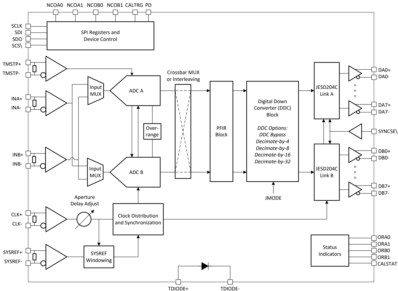
ブロック図
