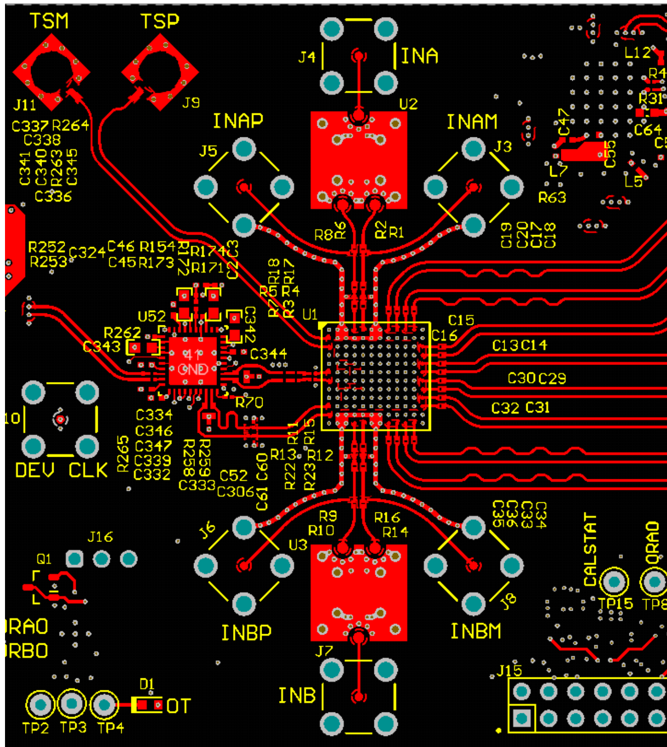
図 7-7. 最上層の配線：アナログ入力、CLK および SYSREF、DA0-3、DB0-3
