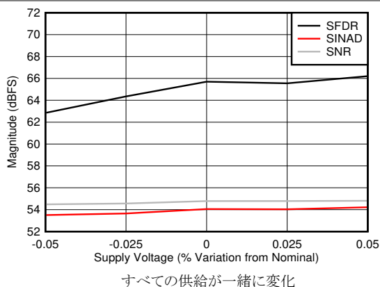
図 5-97. デュアル チャネル モード : SNR、SINAD、SFDR と電源電圧との関係
