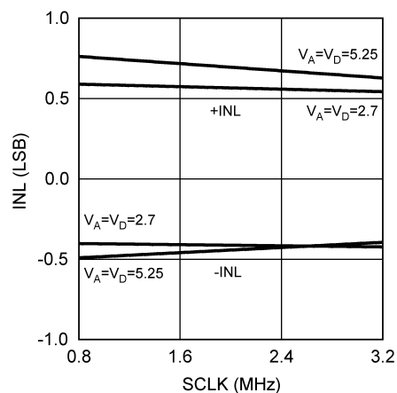
6-19. INL vs SCLK
