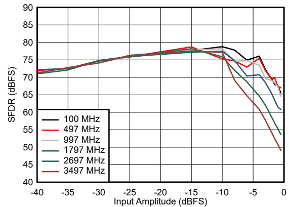
図 5-28. SFDR vs Input Amplitude
