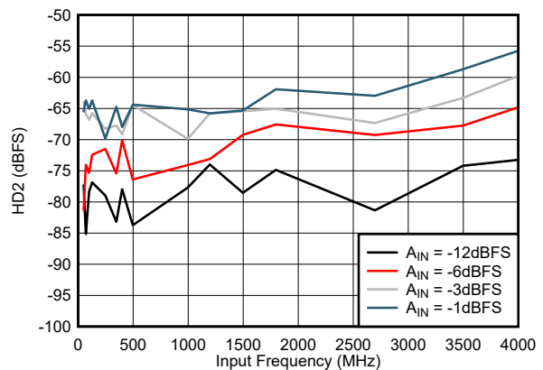
图 5-18. HD2 vs Input Frequency
