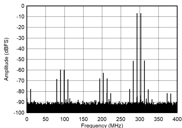
図 5-55. Dual Tone FFT at 2698 MHz
