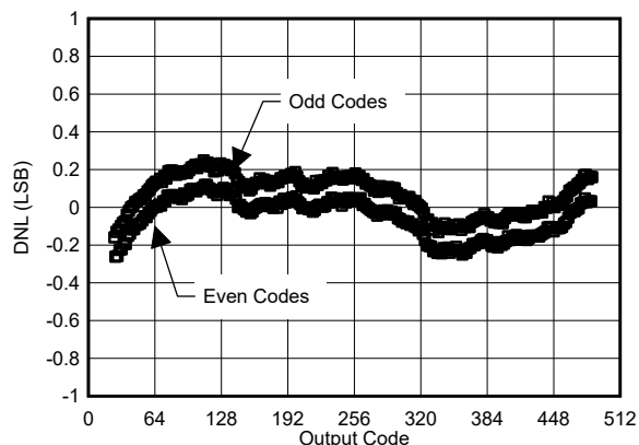
図 5-2. INL vs Code
