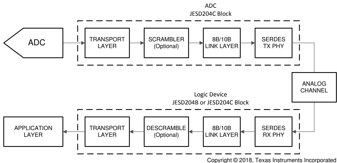
図 6-7. Simplified 8B/10B Encoded JESD204C Interface Diagram
