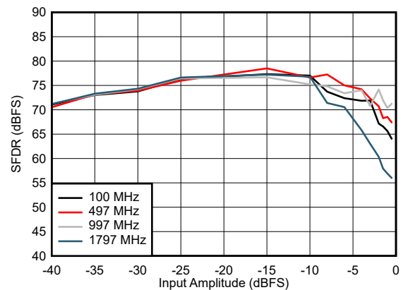
図 5-30. SFDR vs Input Amplitude
