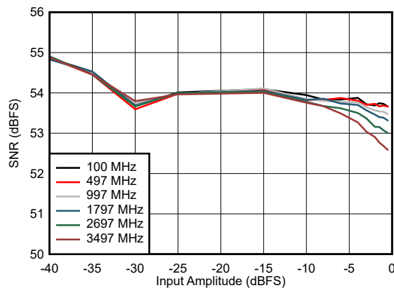
図 5-29. SNR vs Input Amplitude
