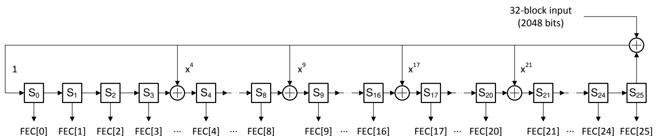
図 6-10. FEC Parity Bit Generator
