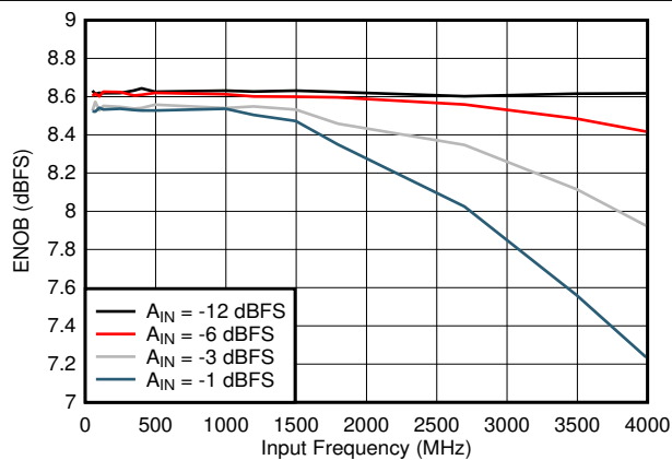
図 5-18. ENOB vs Input Frequency
