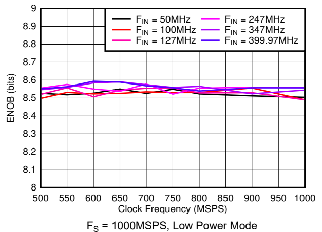
図 5-28. ENOB vs Sample Rate
