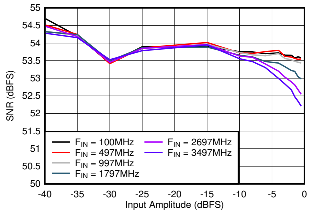
図 5-30. SNR vs Input Amplitude
