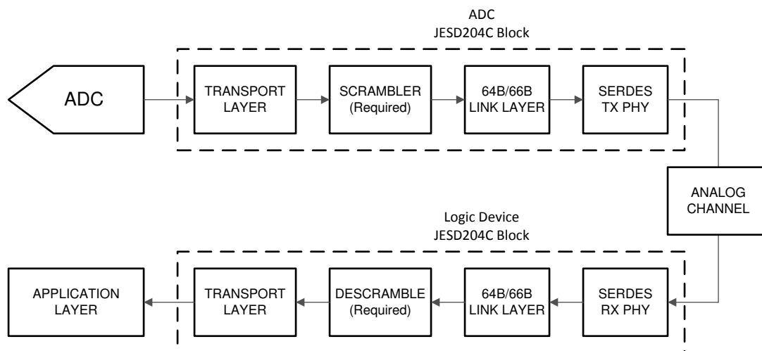
図 6-8. Simplified 64B/66B Encoded JESD204C Interface Diagram
