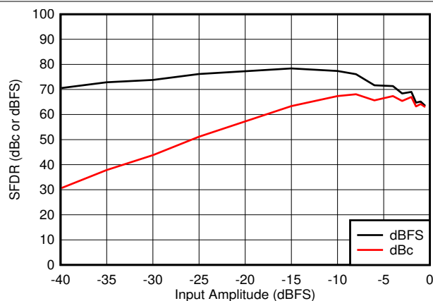
図 5-31. SFDR vs Input Amplitude
