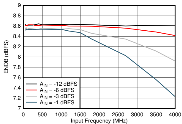
図 5-18. ENOB vs Input Frequency
