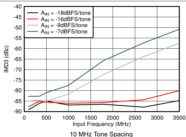
図 5-57. IMD3 vs Input Frequency
