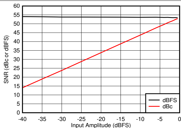
図 5-32. SNR vs Input Amplitude
