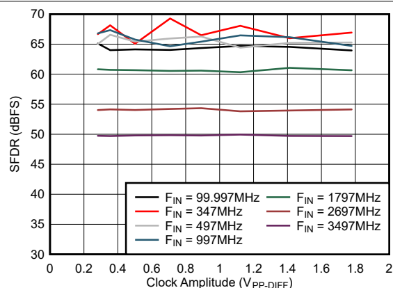
図 5-33. SFDR vs Clock Amplitude
