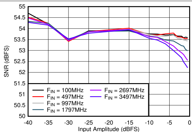
図 5-30. SNR vs Input Amplitude
