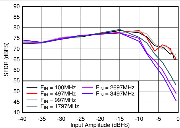
図 5-29. SFDR vs Input Amplitude
