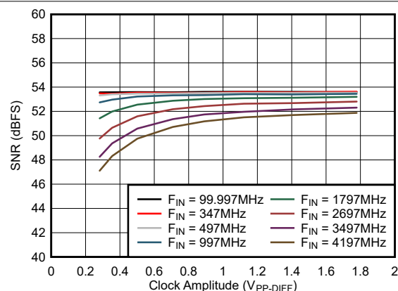
図 5-34. SNR vs Clock Amplitude
