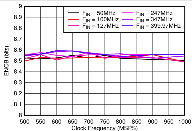
図 5-28. ENOB vs Sample Rate
