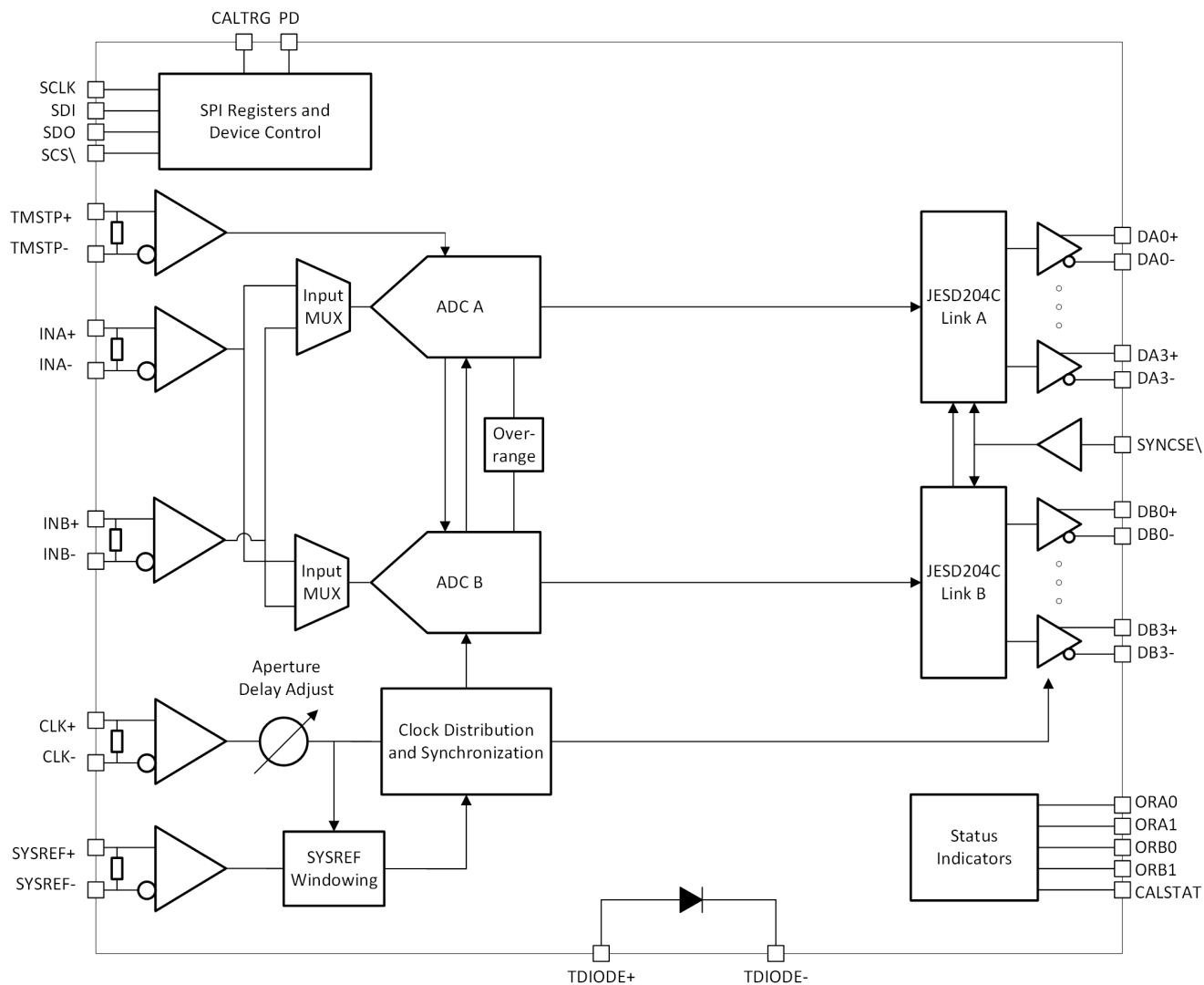
ADC08DJ5200RF ブロック図
