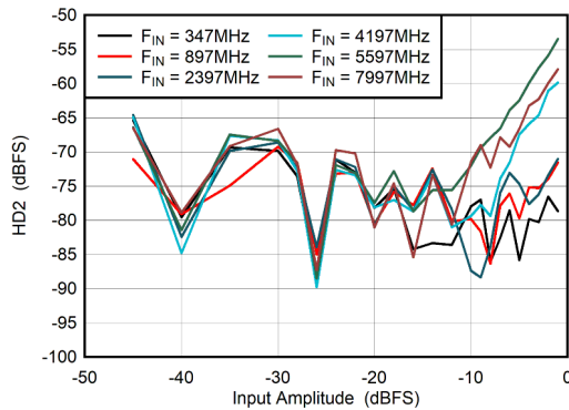
図 5-61. DES Mode: HD2 vs Input Amplitude
