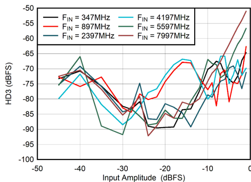
図 5-63. DES Mode: HD3 vs Input Amplitude
