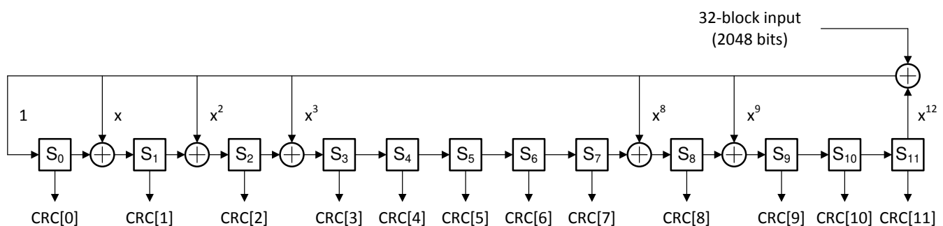
図 6-10. CRC-12 Parity Bit Generator
