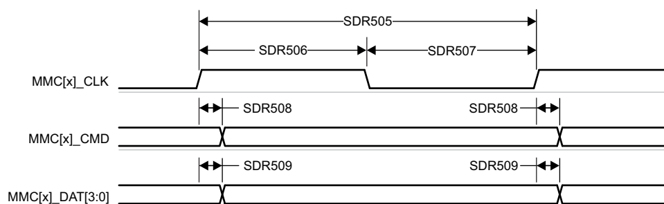
図 6-94. MMC1/2 – UHS-I SDR50 – 送信モード
