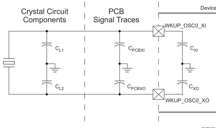
図 6-25. 負荷容量
