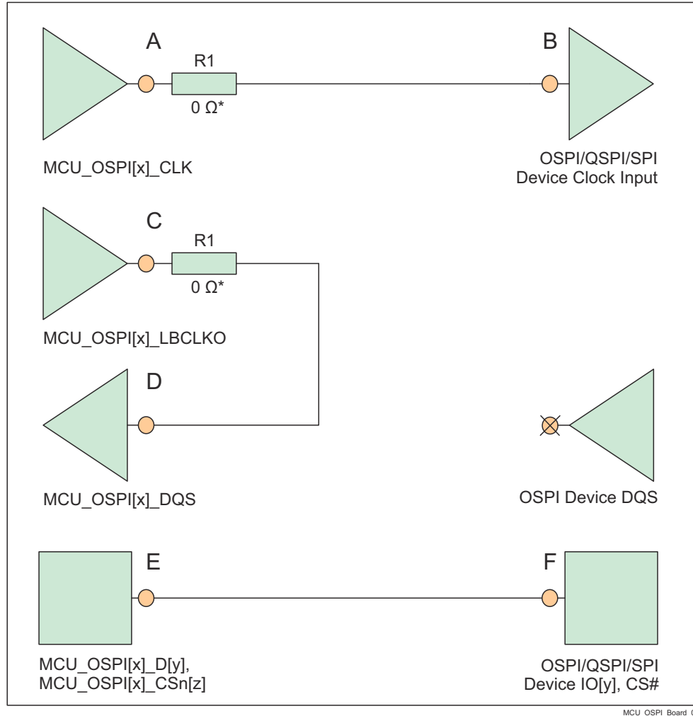
図 7-2. OSPI インターフェイスの概略回路図
