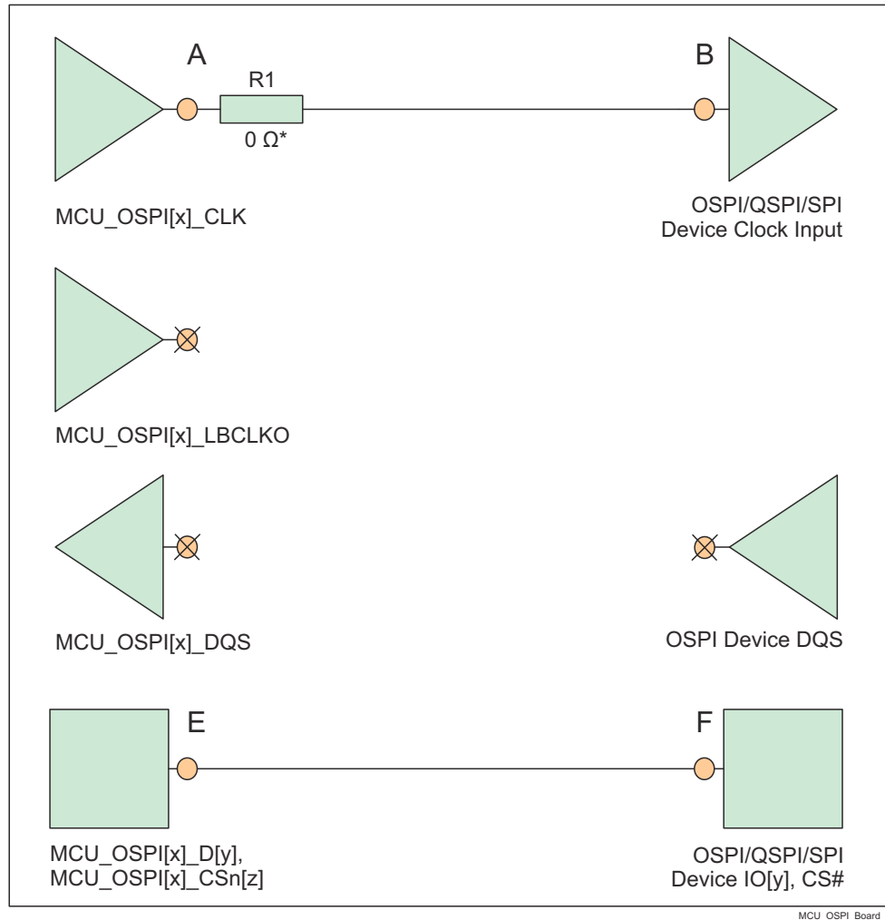
図 10-1. OSPI インターフェイスの概略回路図
