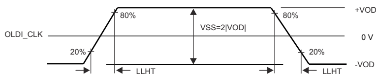
図 6-113. LVDS 出力遷移時間
