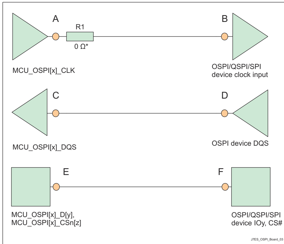
図 8-3. OSPI インターフェ이스の概略回路図
