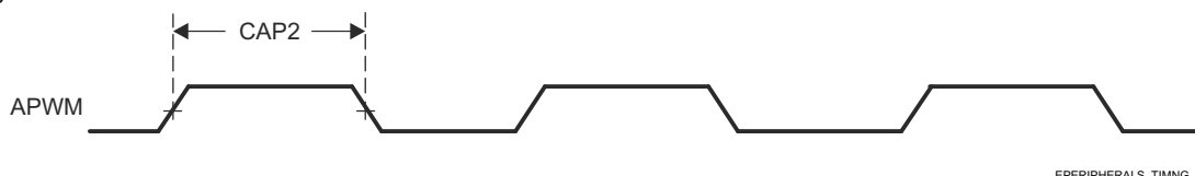
図 6-45. eCAP の出力タイミング
