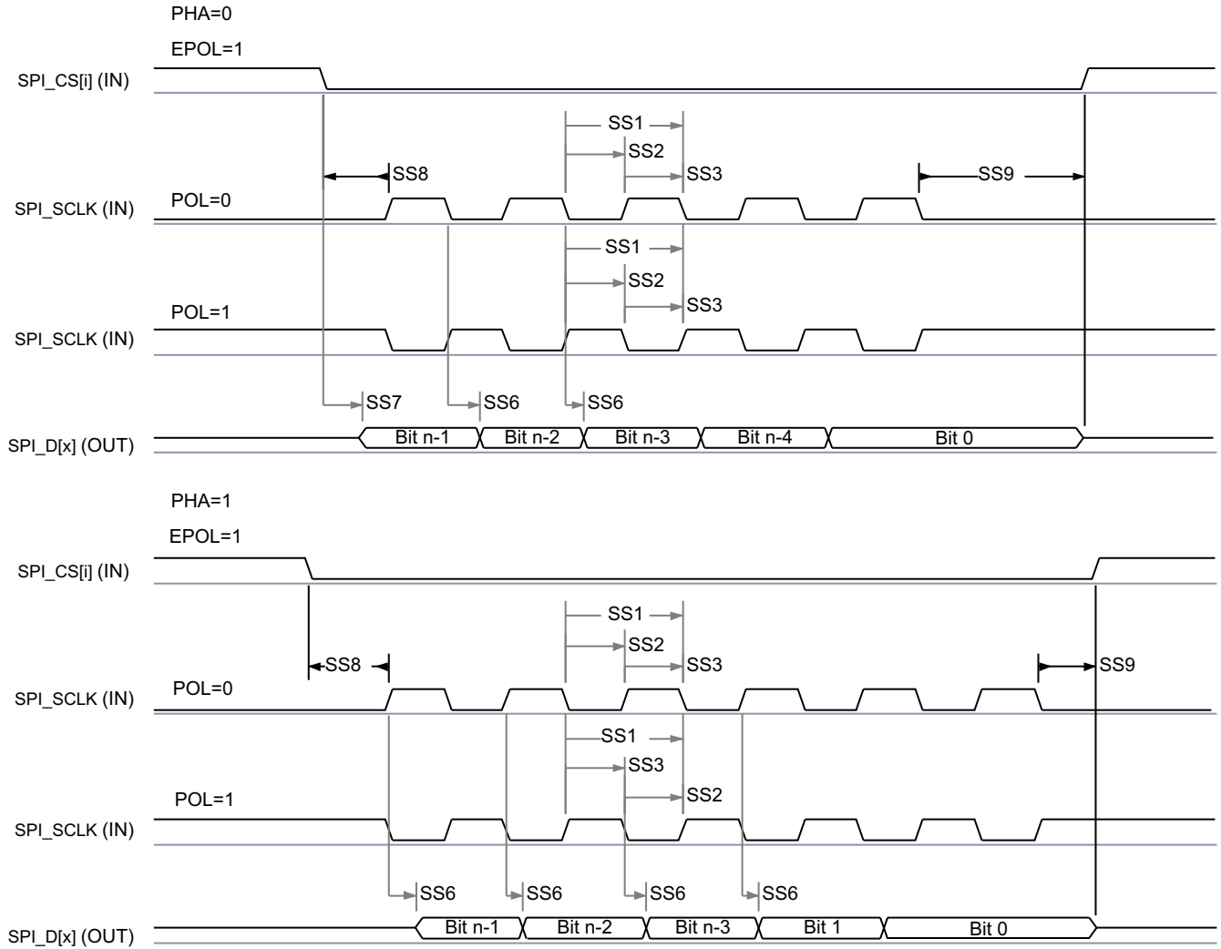
図 7-66. SPI ペリフェラル モードの送信タイミング
