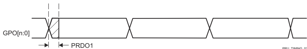
図 7-106. PRUSS PRU 直接出力タイミング
