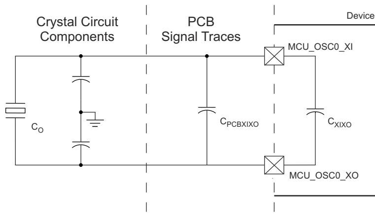
図 7-19. シャント容量
