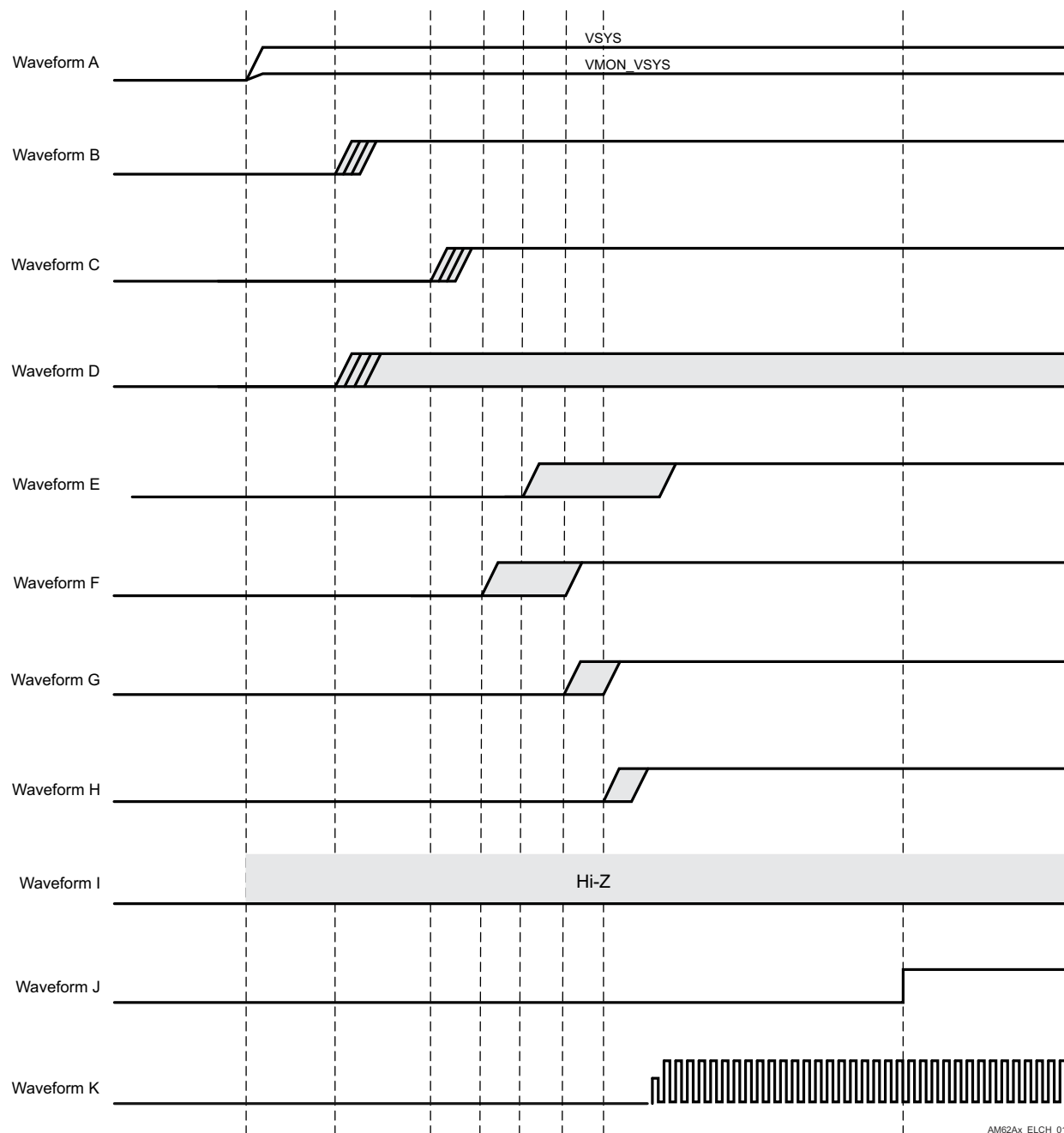
図 7-5. パワーアップ シーケンス
