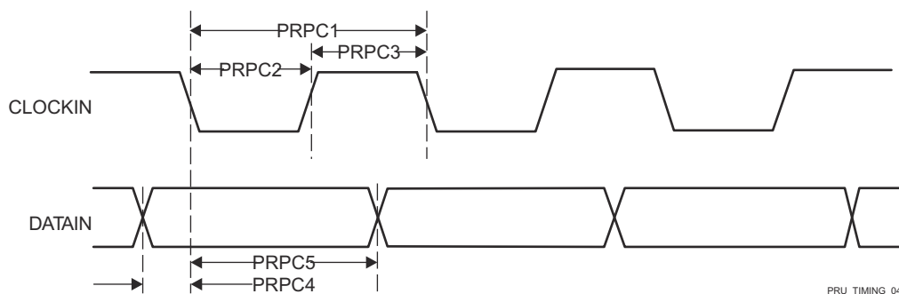
図 7-108. PRUSS PRU パラレル キャプチャのタイミング要件 – 立ち下がりエッジ モード
