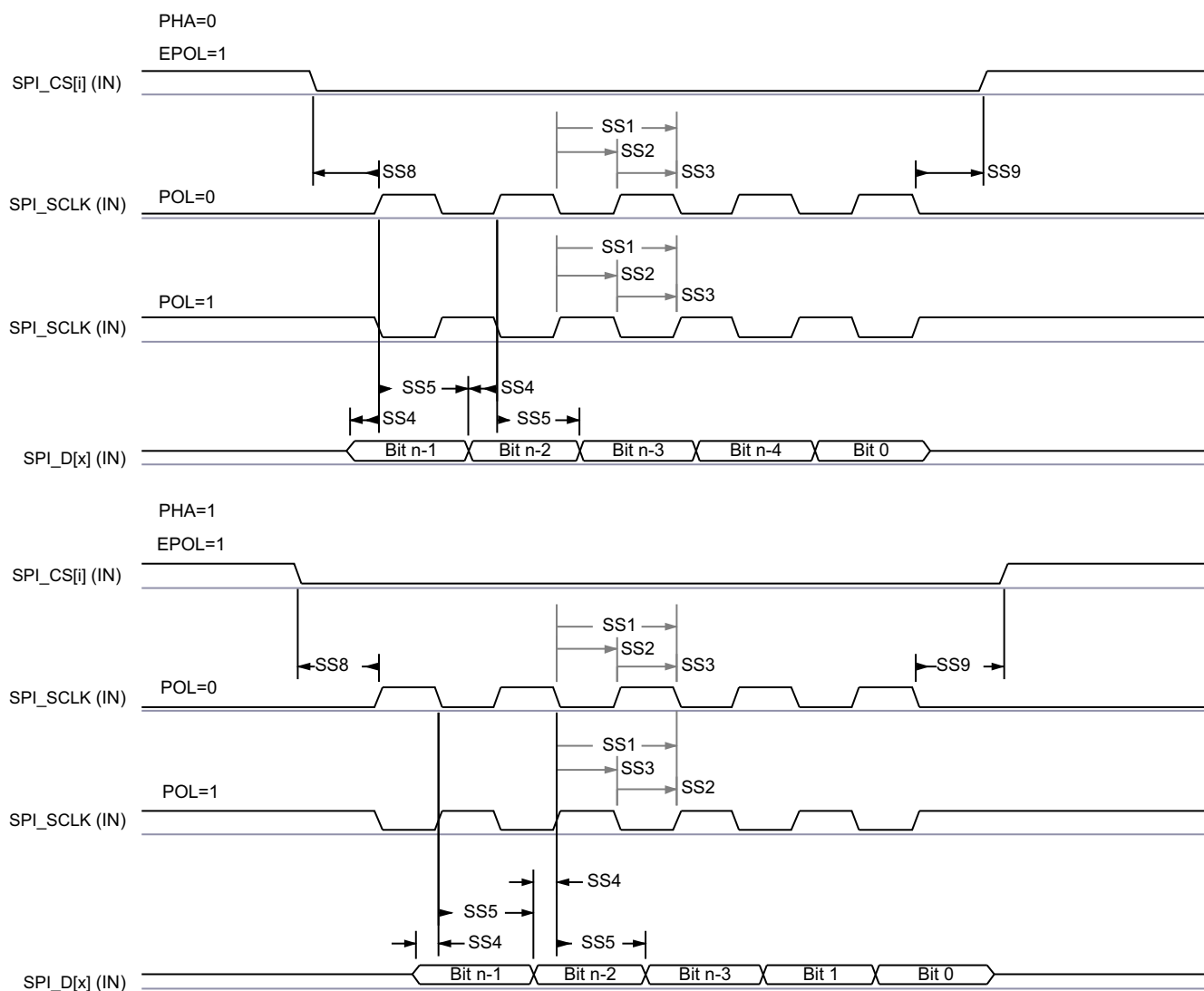
図 7-65. SPI ペリフェラル モードの受信タイミング
