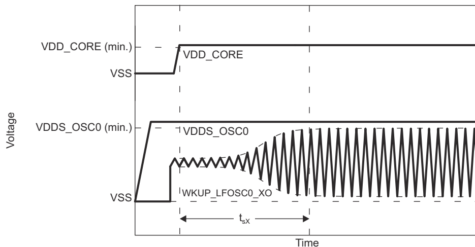
図 7-23. WKUP_LFOSC0 スタートアップ時間
