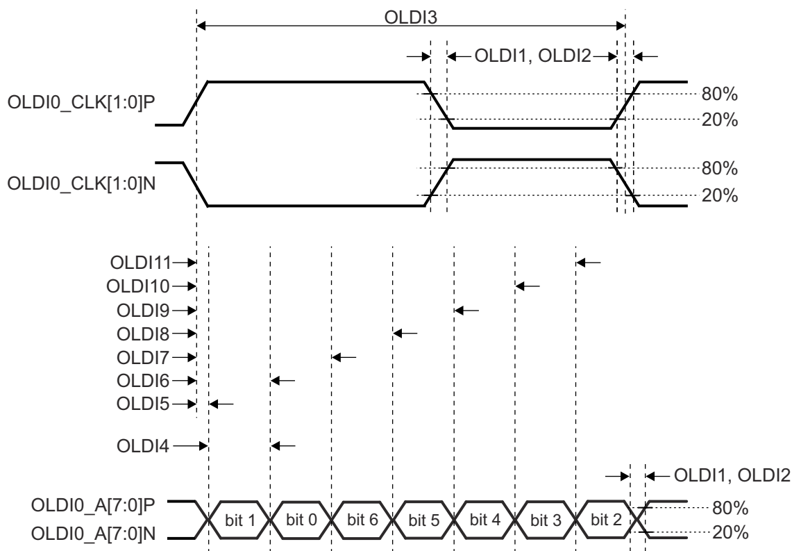
図 7-94. OLDI0 のスイッチング特性
