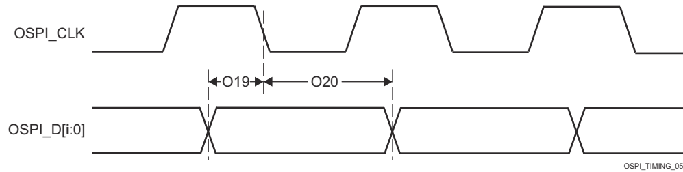
図 7-102. OSPI0 のタイミング要件 – タップ SDR、ループバックなし
