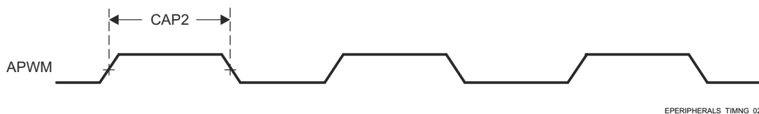
図 7-38. ECAP のスイッチング特性
