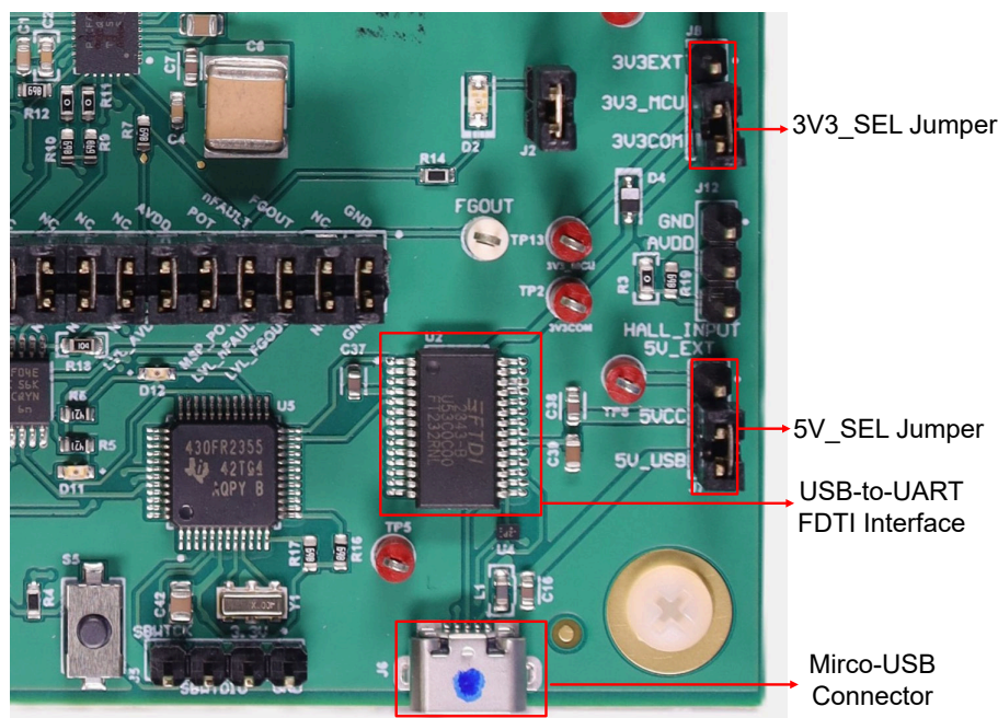
图 2-4. Micro-USB 连接器和 USB 转 UART 接口
