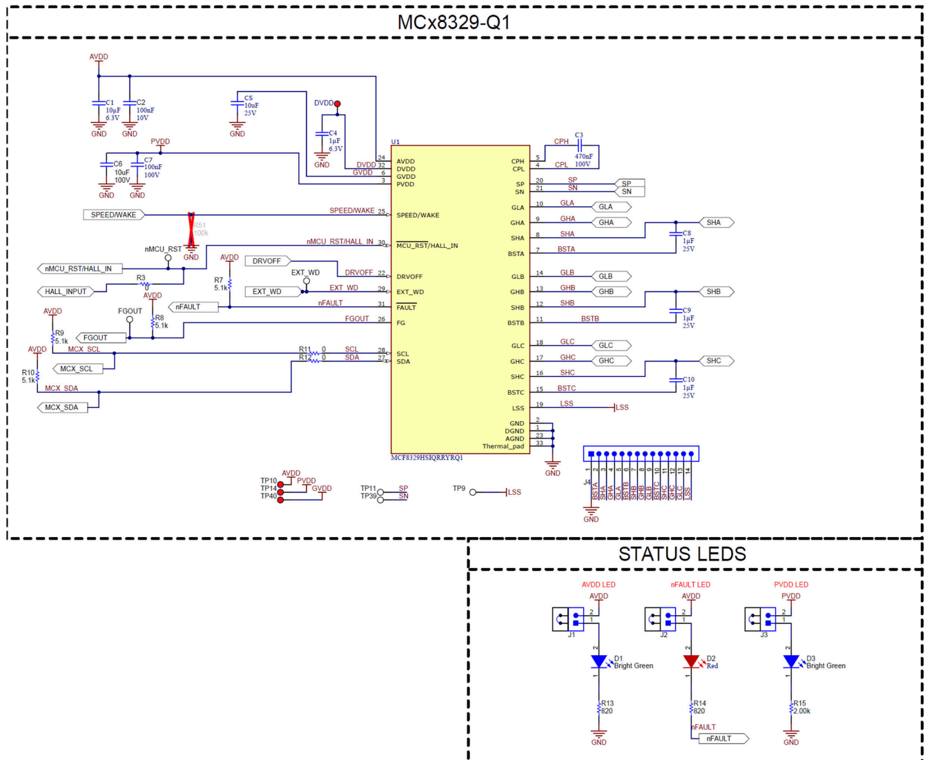
图 4-2. 驱动器
