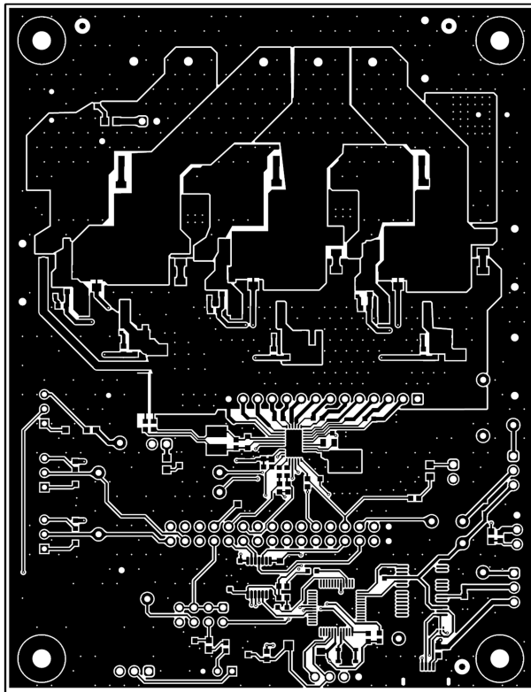
图 4-7. EVM 顶层
