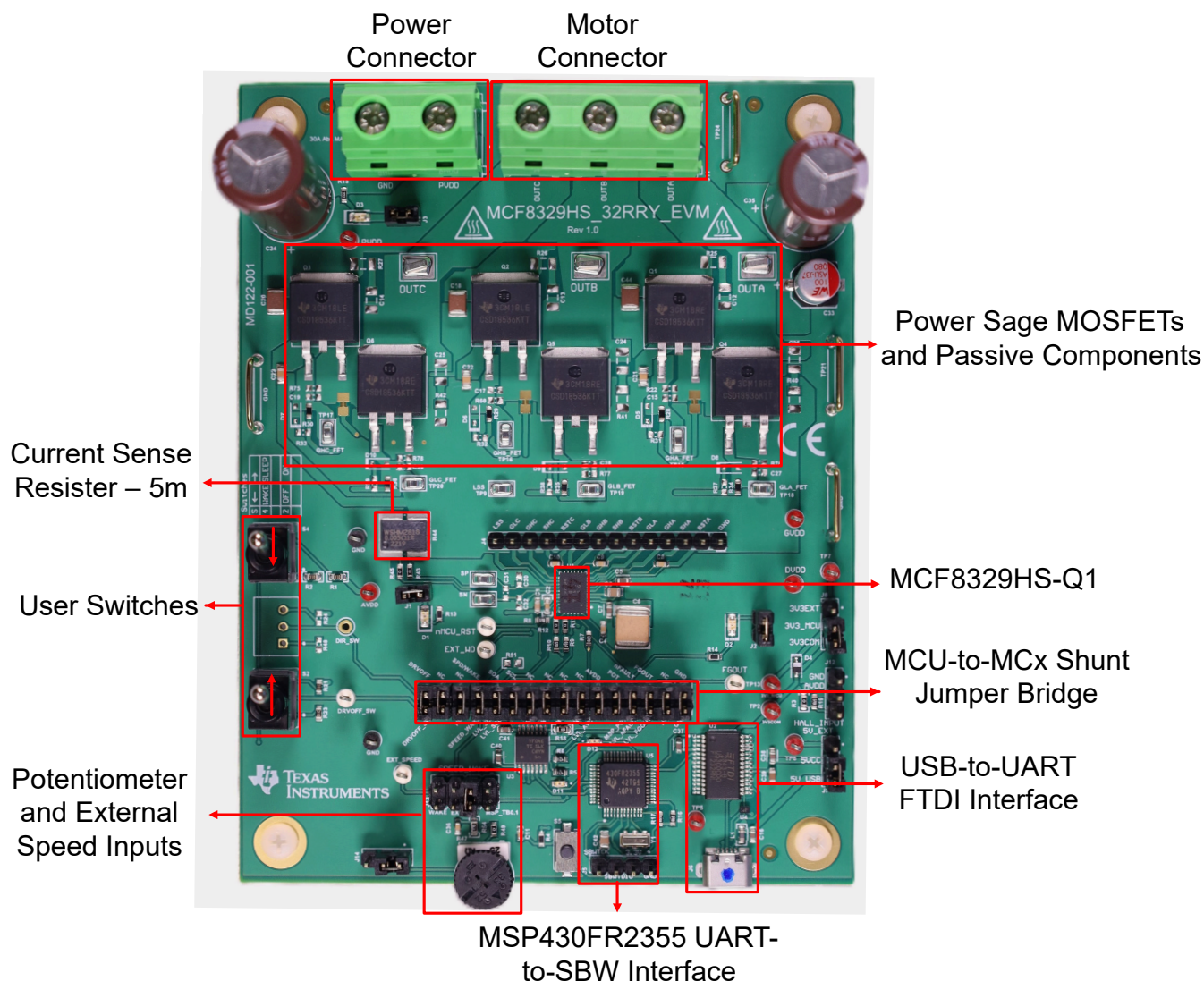
图 2-2. MCF8329HSRRYEVM 主要硬件模块
