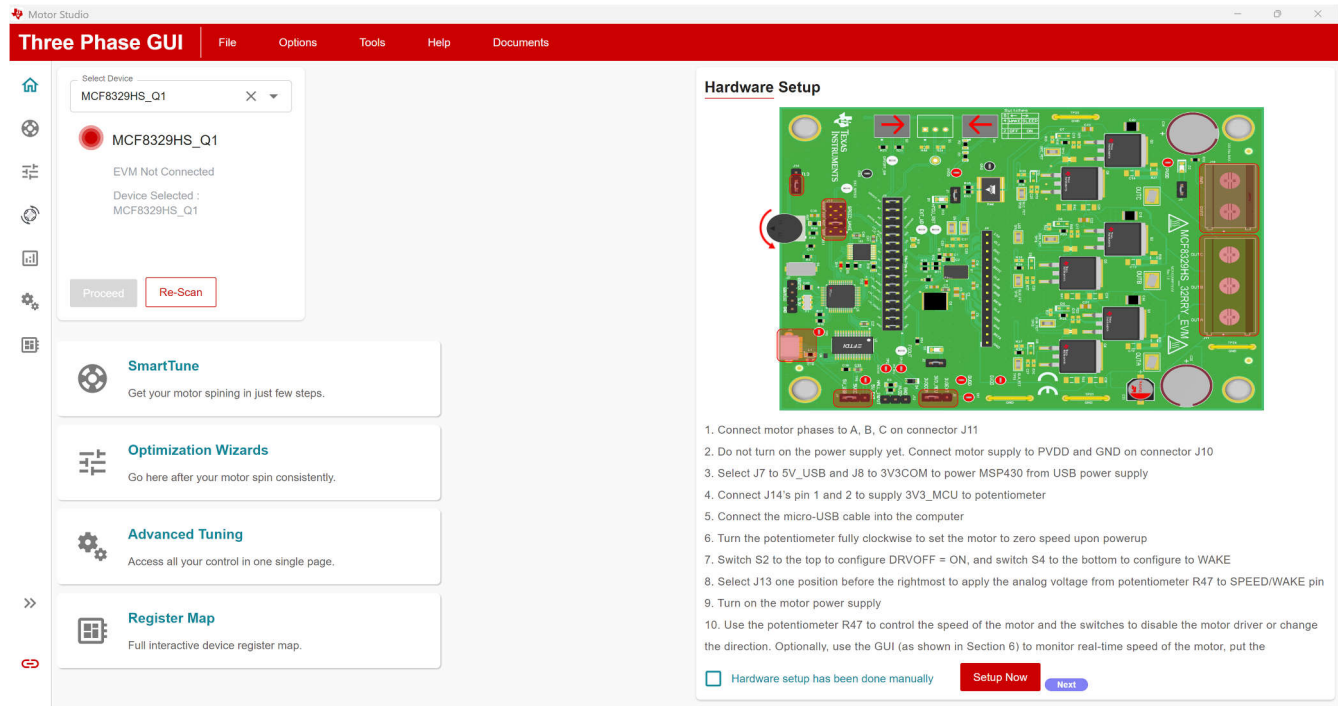
图 3-1. Motor Studio GUI MCF8329HS-Q1 主页
