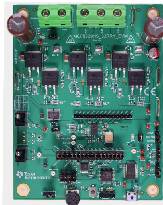
MCF8329HSRRYEVM ( 顶视图 )
