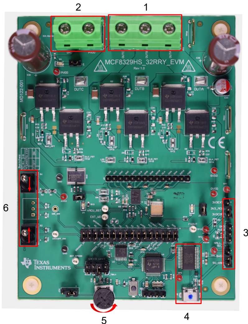
图 2-1. 快速入门指南参考
