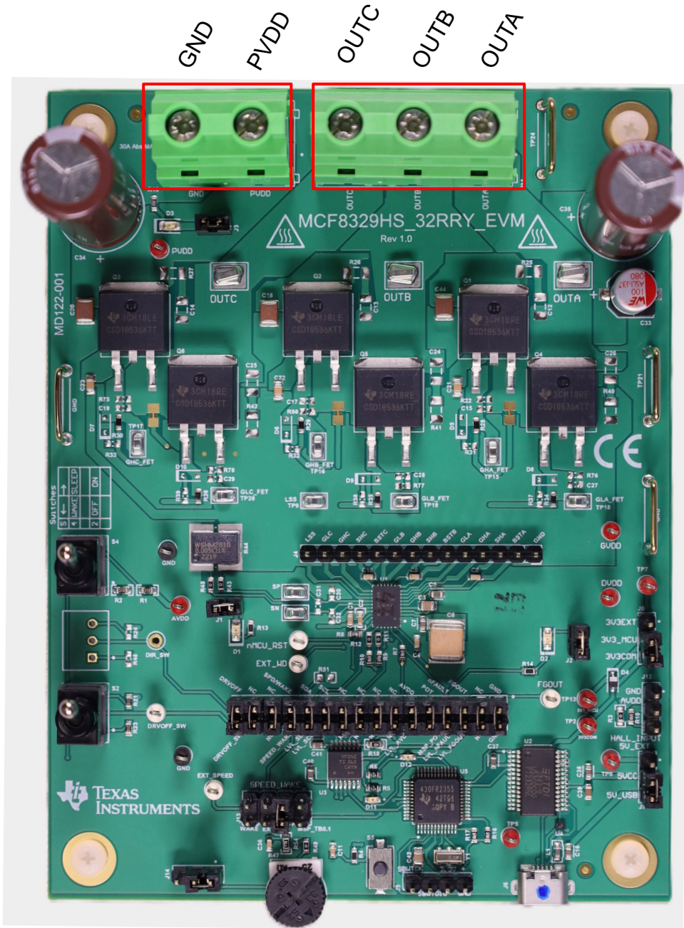
图 2-3. 从电机到 MCF8329HSRRYEVM 的连接
