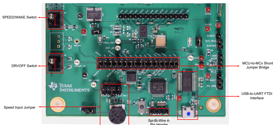
图 2-5. MCF8329RRYEVM 上的 MSP430FR2355 MCU
