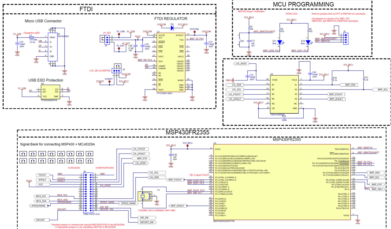
图 4-1. 接口
