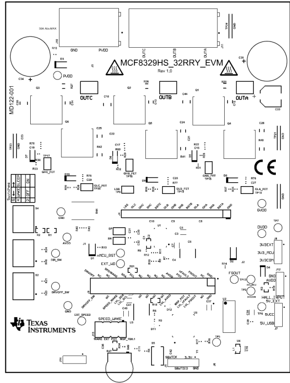
图 4-6. EVM 顶部覆盖层
