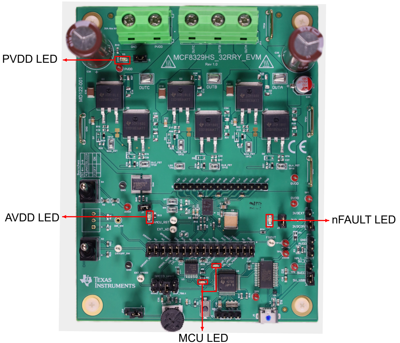
图 2-6. MCF8329HSRRYEVM LED 位置
