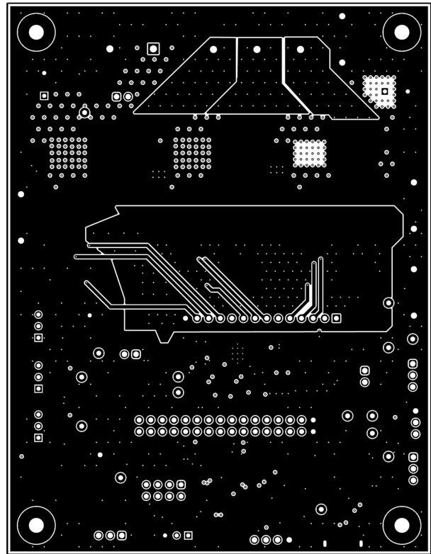
图 4-8. EVM 信号层 1
