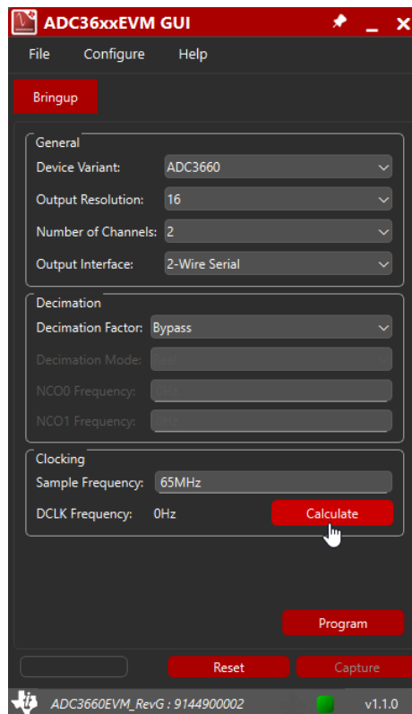
图 4-5. 计算 ADC3660 的 DCLK 频率
