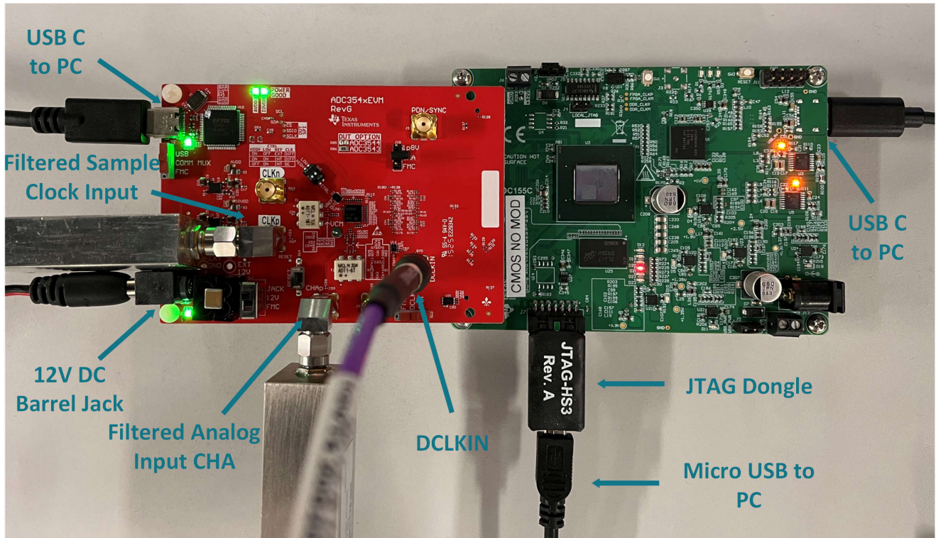
图 4-2. ADC3660EVM 硬件设置
