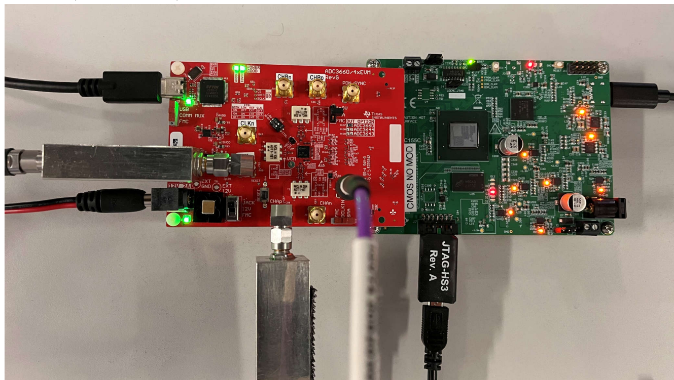
图 4-20. TSWDC155EVM 已上电
