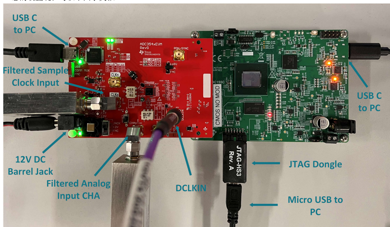
图 4-10. ADC3644EVM 硬件设置
