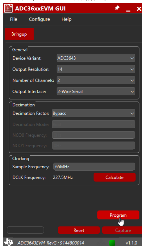
图 4-22. 对 ADC3643EVM 进行编程
