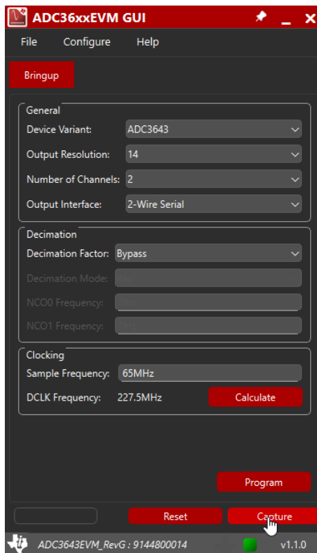
图 4-23. 采集 FFT
