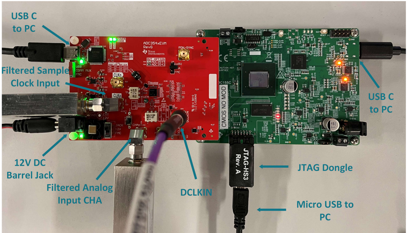
图 4-18. ADC3643EVM 硬件设置
