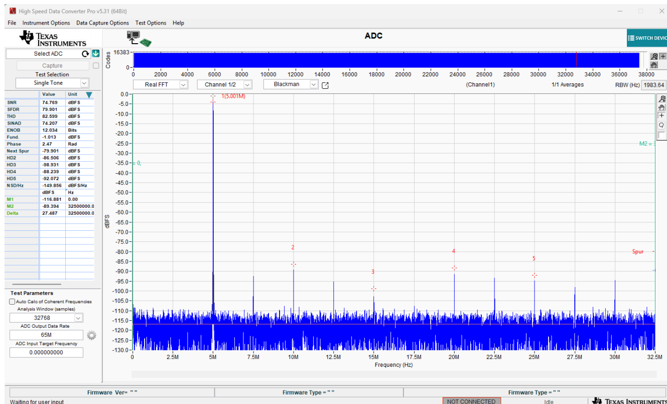
图 4-16. HSDC Pro 中的 ADC3644EVM FFT 数据采集
