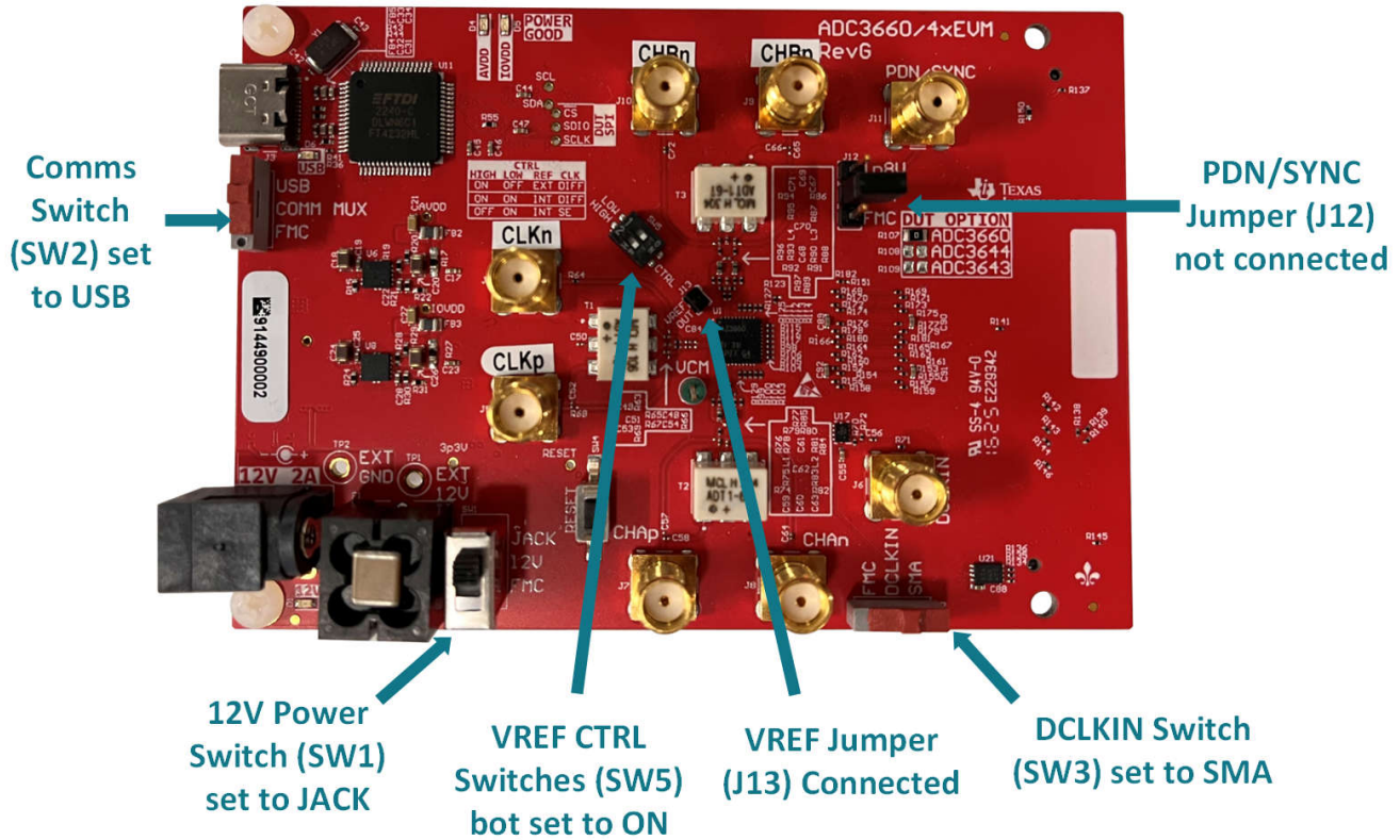
图 2-2. ADC3660/ADC364xEVM 开关和跳线
