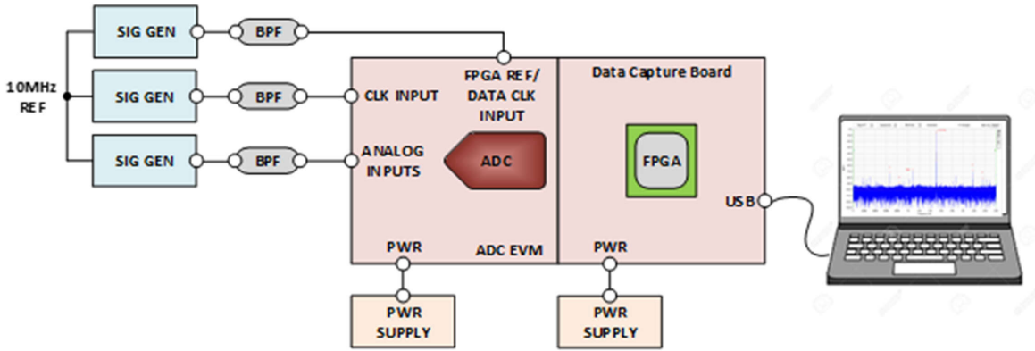
图 4-17. 基本测试测量设置
