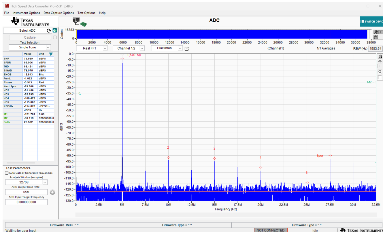
图 4-24. HSDC Pro 中的 ADC3643EVM FFT 数据采集
