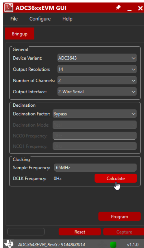
图 4-21. 计算 ADC3643 的 DCLK 频率
