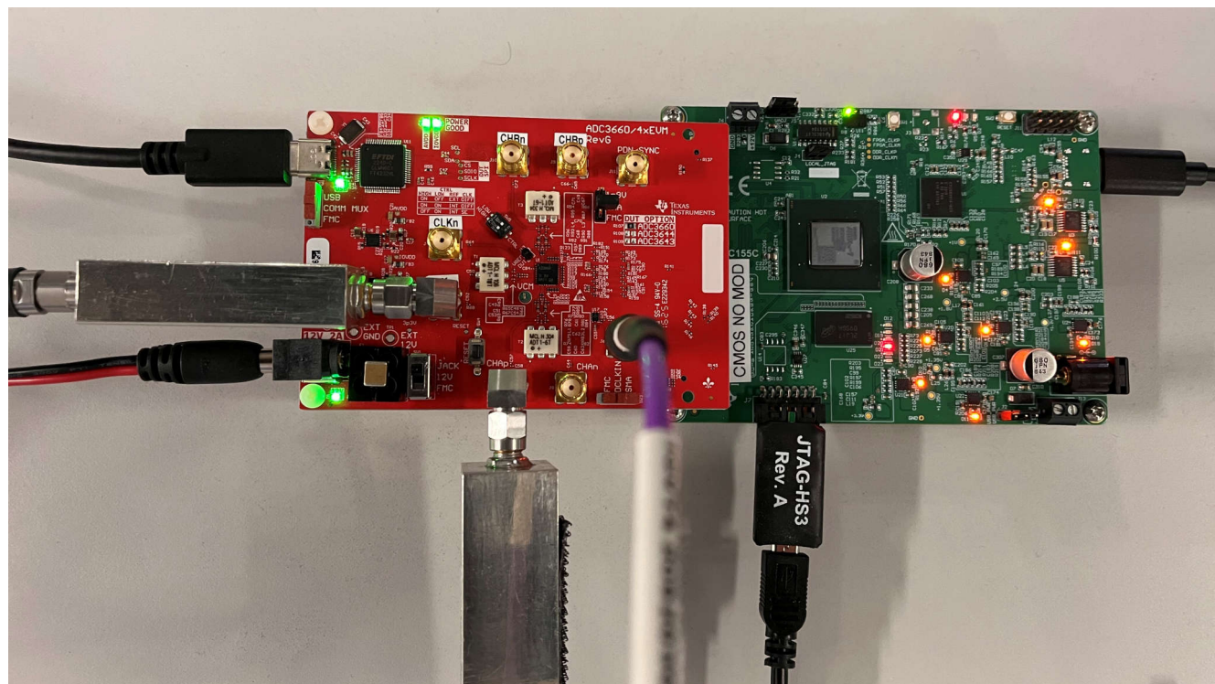
图 4-12. TSWDC155EVM 已上电
