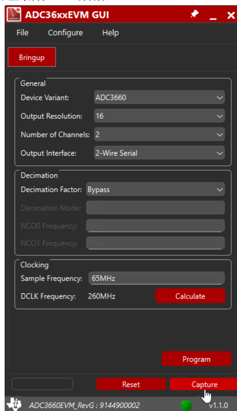
图 4-7. 采集 FFT
