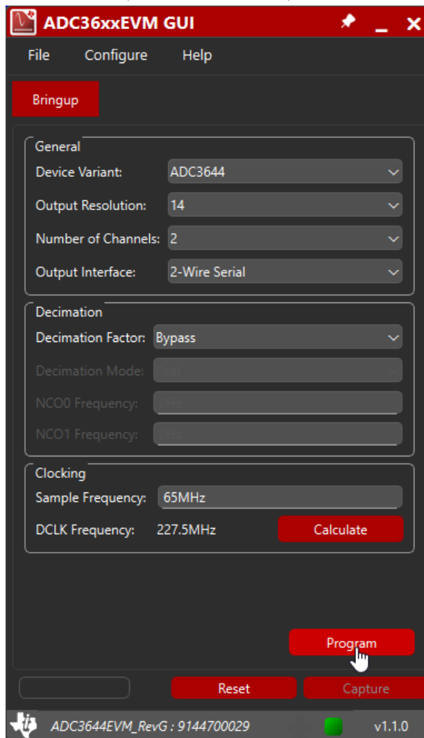
图 4-14. 对 ADC3644EVM 进行编程
