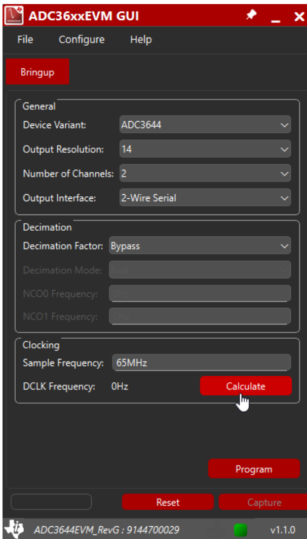
图 4-13. 计算 ADC3644 的 DCLK 频率
