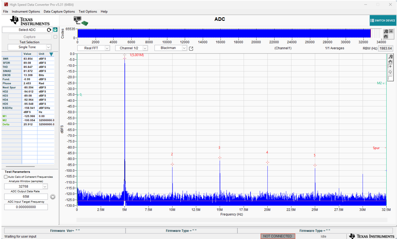
图 4-8. HSDC Pro 中的 ADC3660EVM FFT 数据采集
