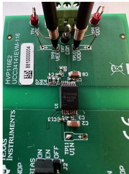
图 2-2. PCB 示波器探头测试点
