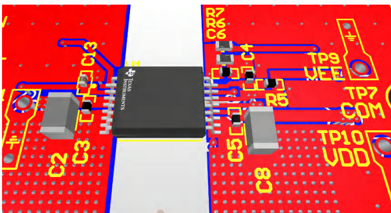
图 3-13. 顶面，元件放置和布线
