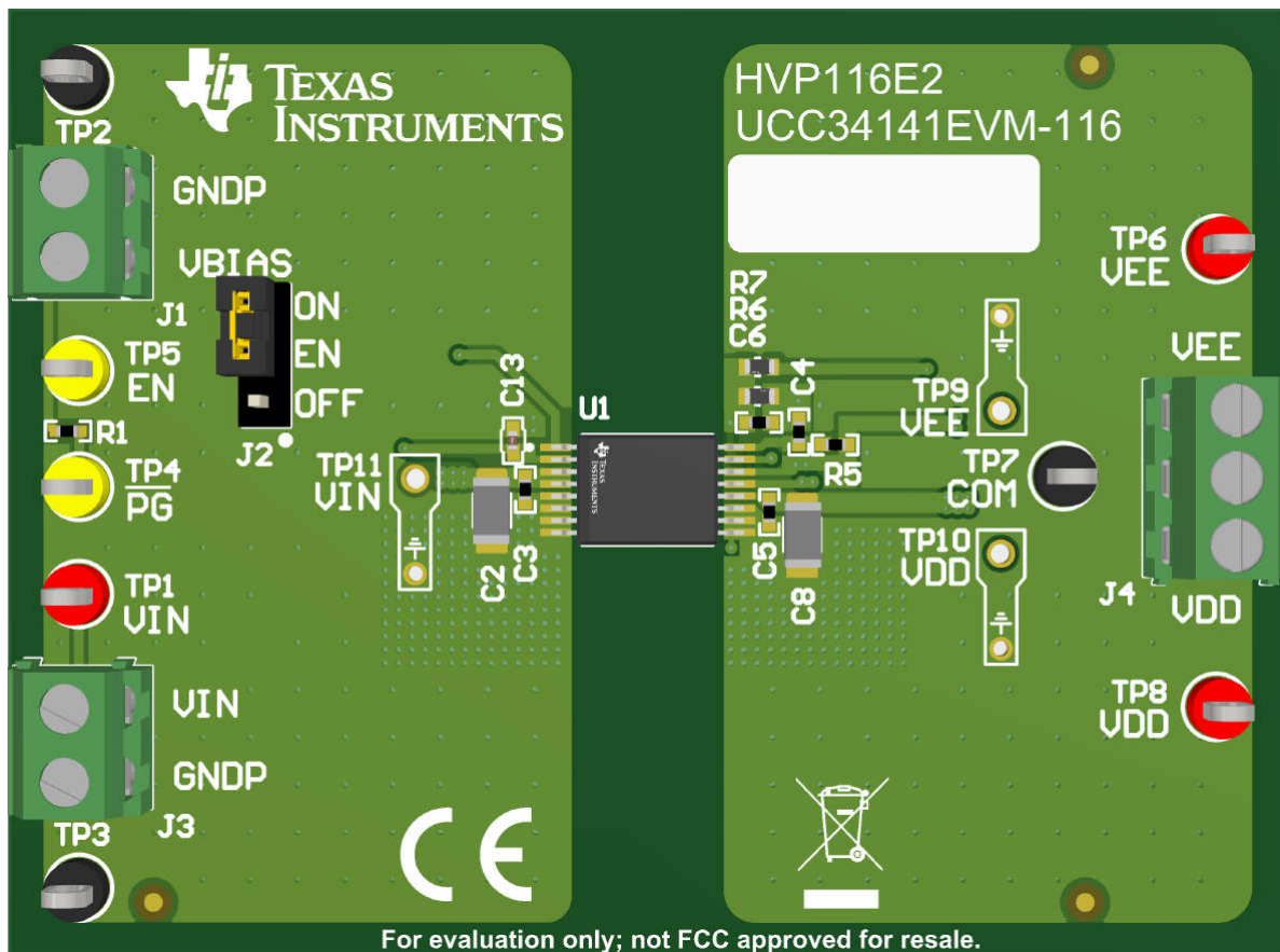
图 3-2. 经全面组装的 3D 顶视图
