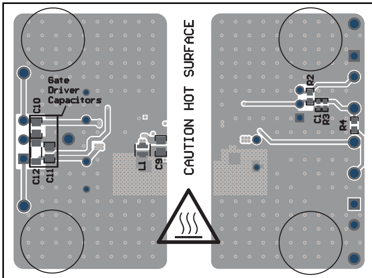
图 3-7. PCB 底层，组装（镜像视图）
