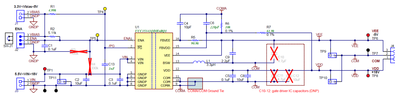
图 3-1. 原理图 ( UCC35341 型号 )
