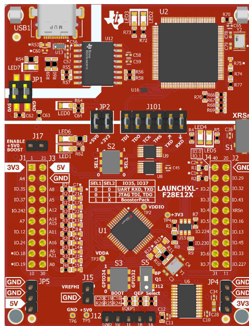
F28E12x LaunchPad™ 电路板
