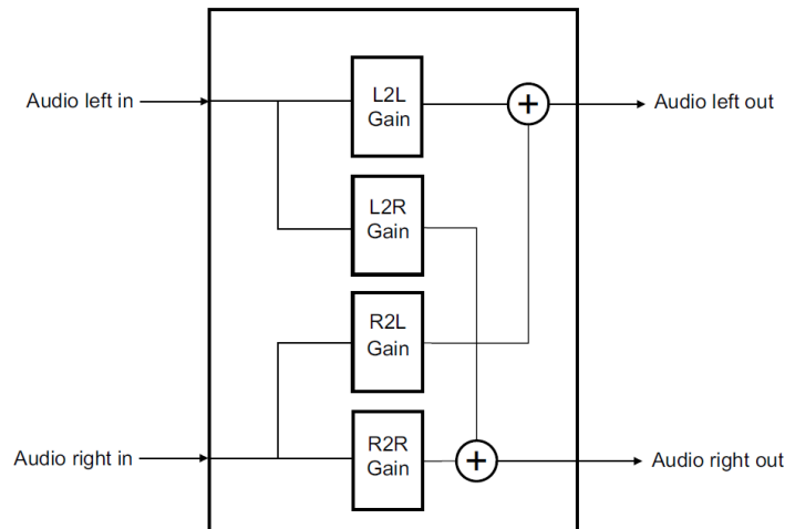
图 3-1. 输入混合器
