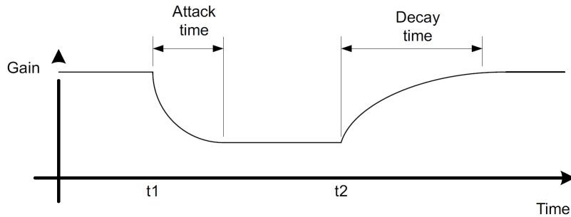
图 3-14. 双频带 DRC 起音和衰减
