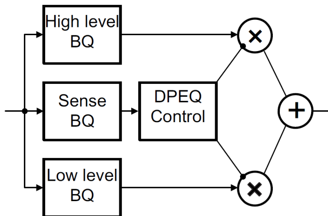
图 3-8. DPEQ
