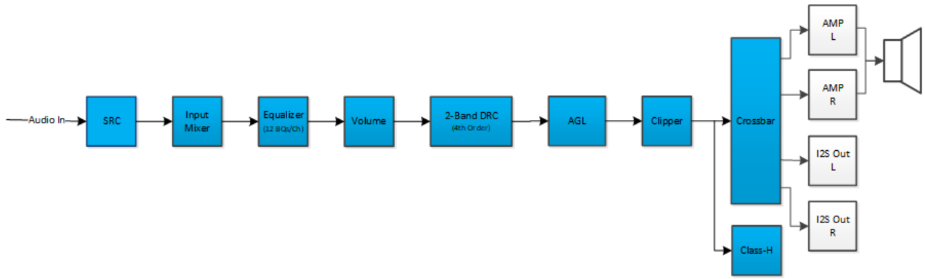
图 2-6. 处理流程 6
