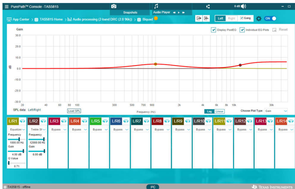
图 3-5. 均衡器调优窗口
