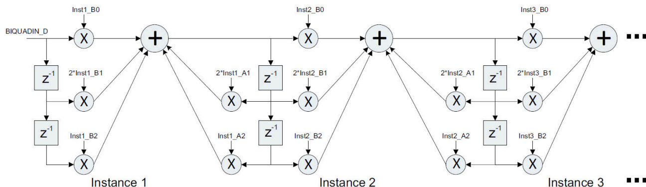
图 3-4. 级联 BQ 结构
