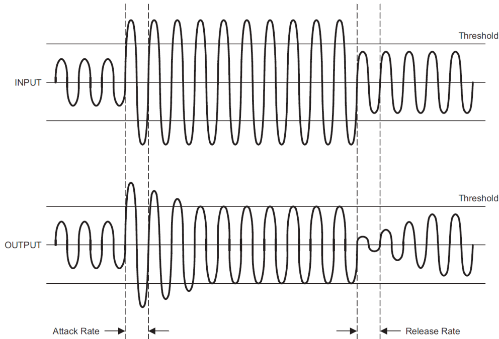
图 3-17. AGC 起音和释放
