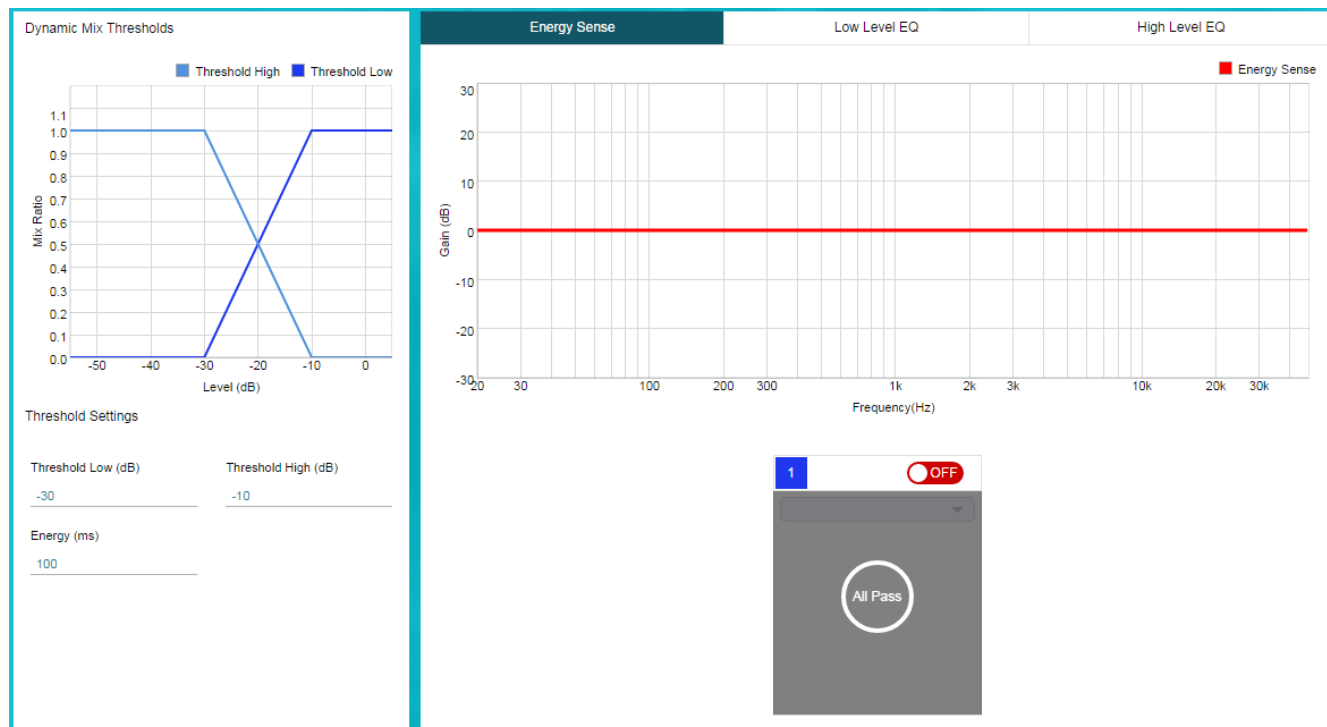
图 3-9. DPEQ 调优窗口
