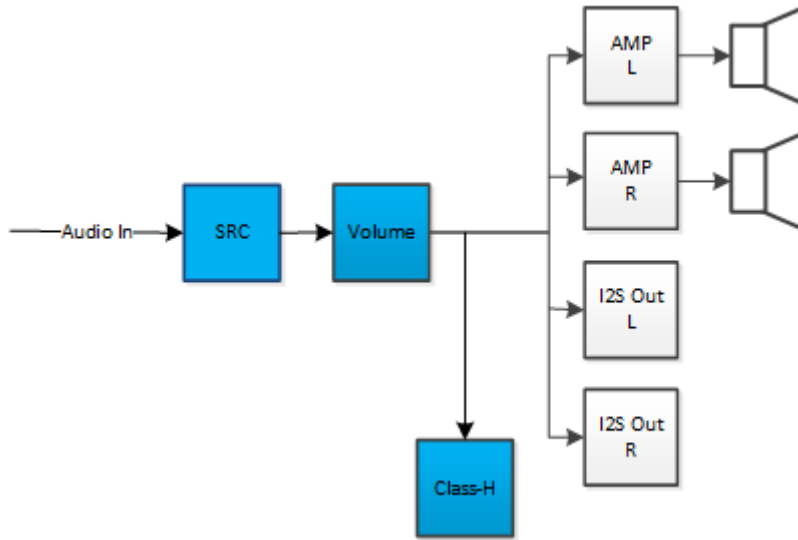
图 2-4. 处理流程 4
