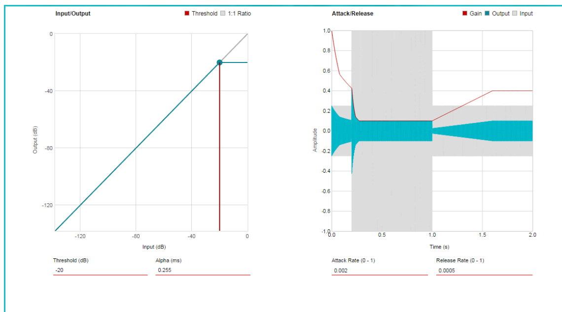
图 3-16. AGL 调优窗口
