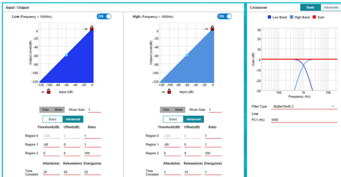
图 3-15. 双频带 DRC 调优窗口
