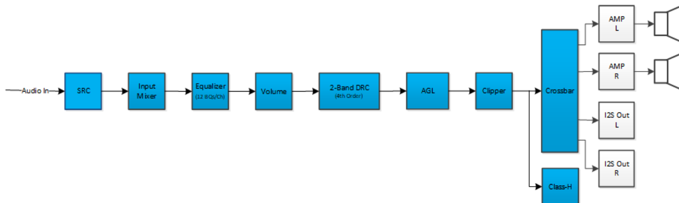
图 2-3. 处理流程 3
