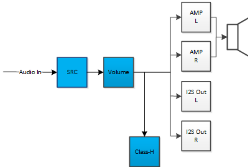
图 2-8. 处理流程 8
