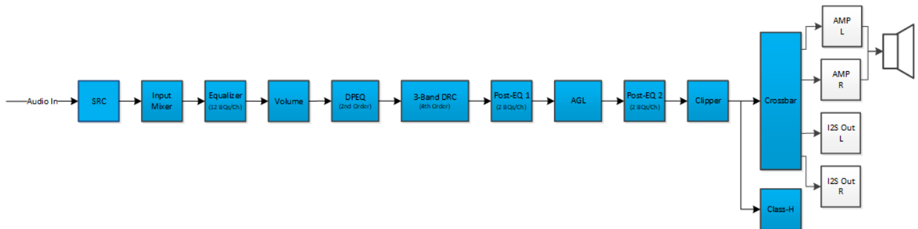
图 2-5. 处理流程 5
