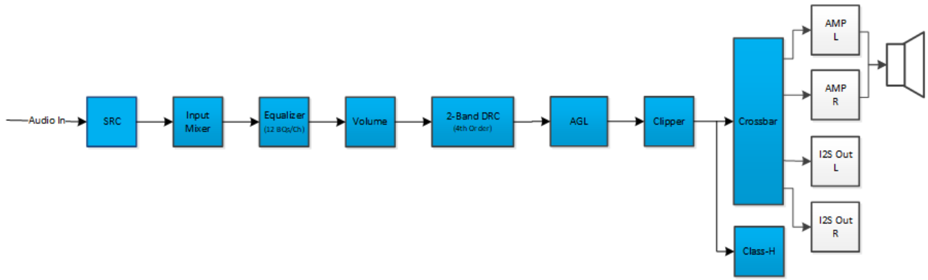
图 2-7. 处理流程 7
