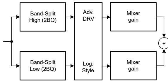
图 3-13. 双频带 DRC
