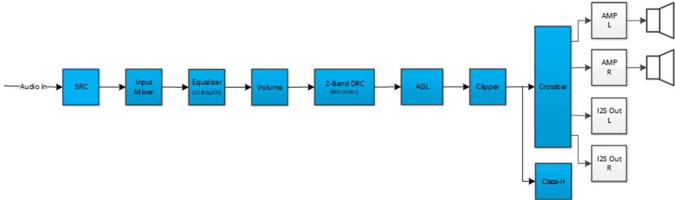
图 2-2. 处理流程 2
