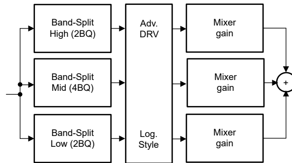
图 3-10. 三频带 DRC
