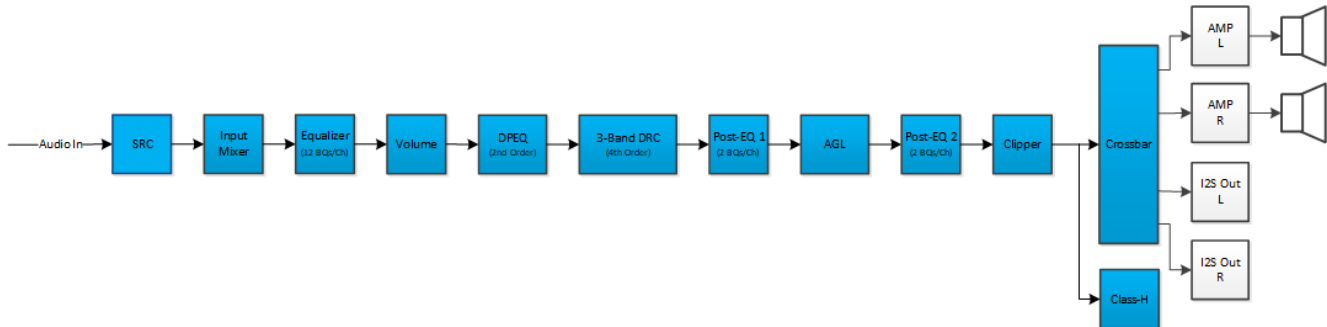
图 2-1. 处理流程 1
