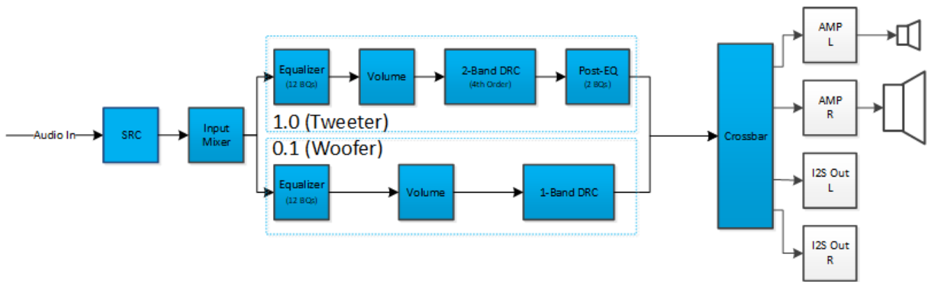
图 2-9. 处理流程 9
