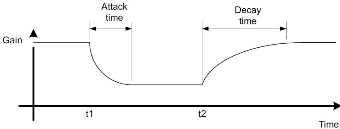
图 3-11. DRC 起音和衰减
