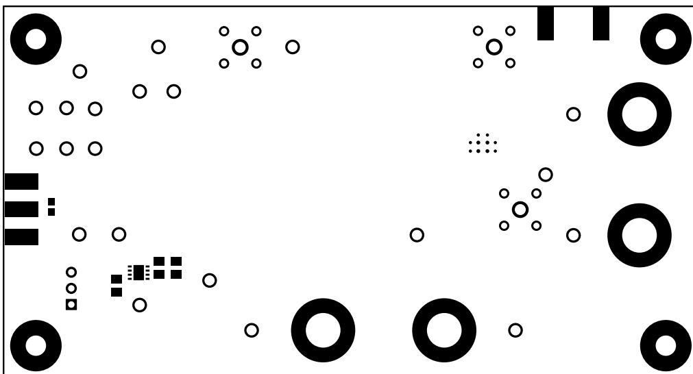
图 4-8. 底部阻焊层
