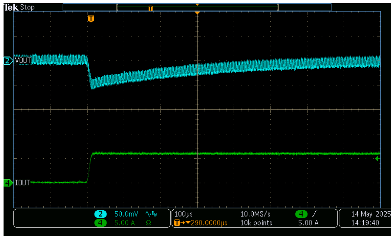
图 3-3. 对 100mA 至 6A 负载阶跃的瞬态响应 (以 8A/µs 的速率)
