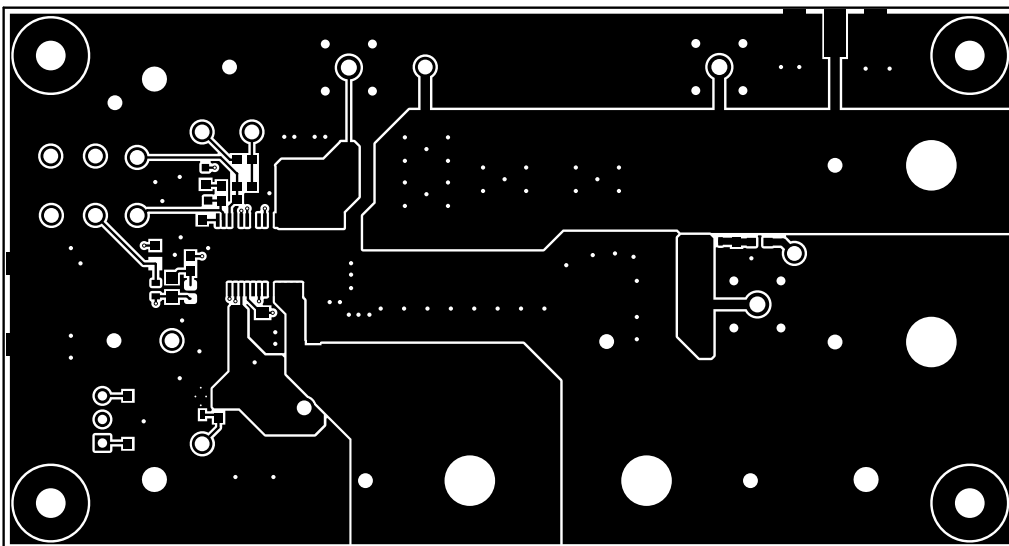
图 4-4. 第 1 层 ( 顶部 )
