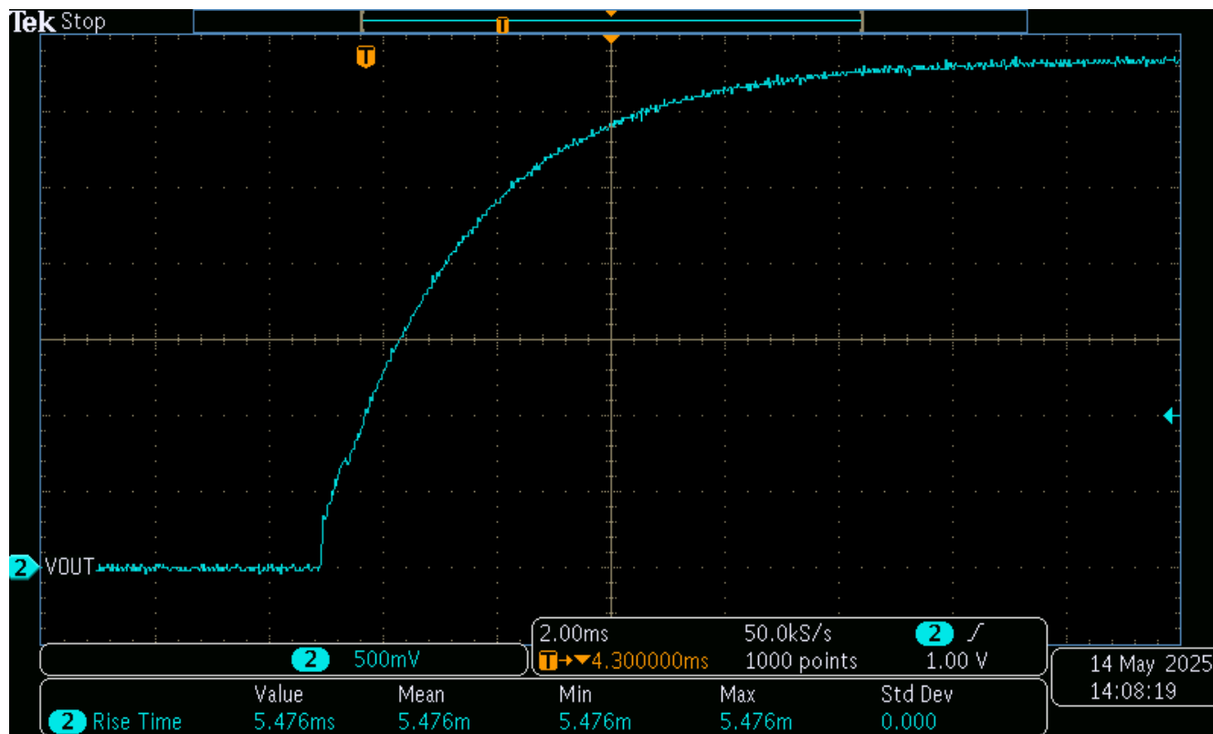
图 3-1. 软启动进入 550mΩ 负载
