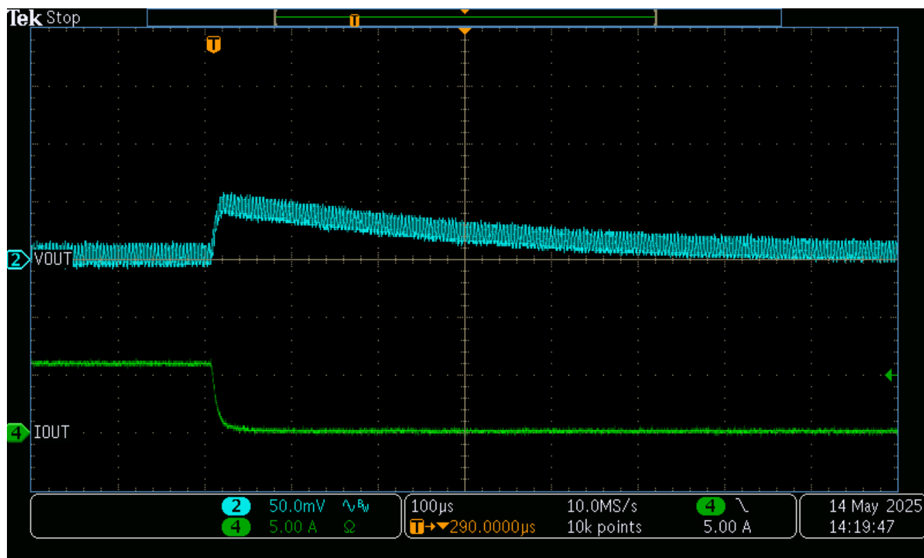
图 3-4. 对 6A 至 100mA 负载阶跃的瞬态响应 (以 8A/µs 的速率)
