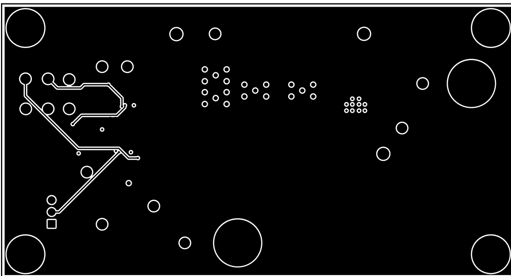
图 4-5. 第 2 层
