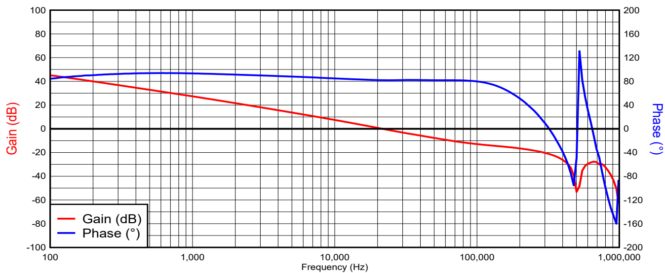
图 3-5. 频率响应 IOUT = 6A
