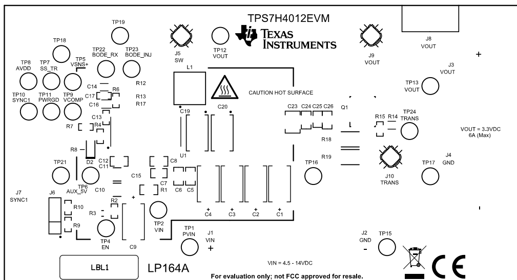
图 4-2. 顶层丝印层
