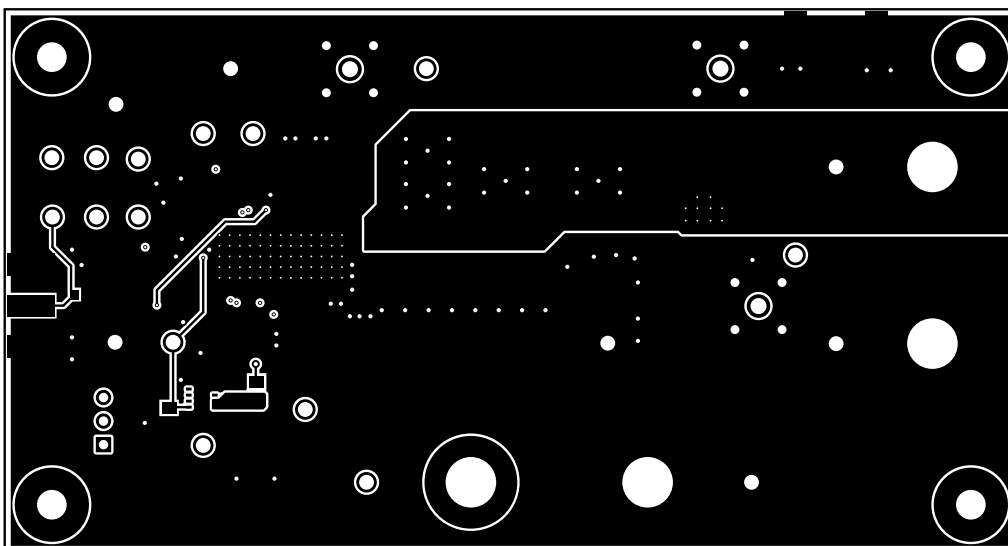
图 4-7. 第 4 层 (底部)
