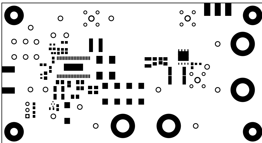
图 4-3. 顶部阻焊层
