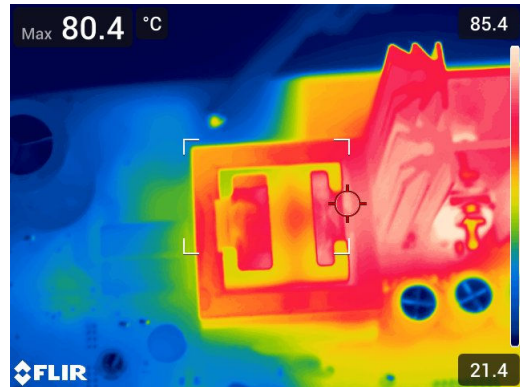
图 3-5. 热像图顶部
