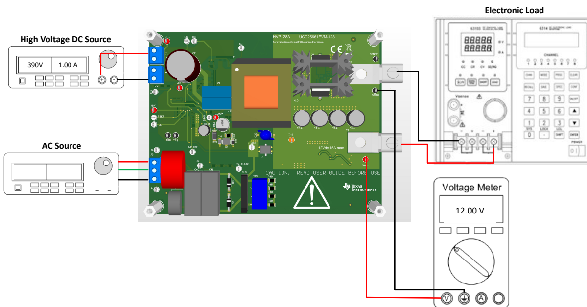
图 2-1. UCC25661EVM-128 测试设置图
