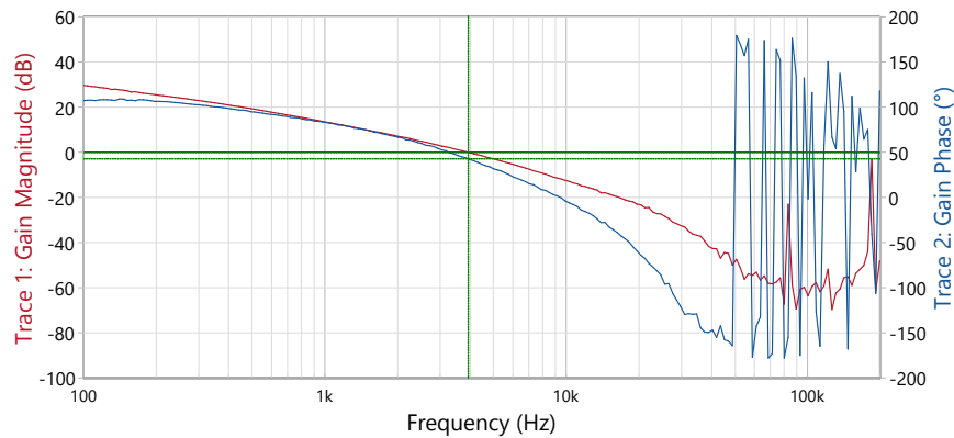
图 3-9. 15A 负载时的波特图
