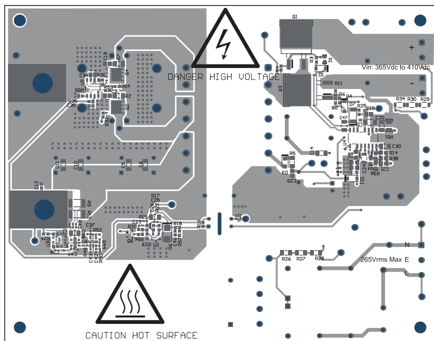
图 4-4. UCC25661EVM-128 (底视图)
