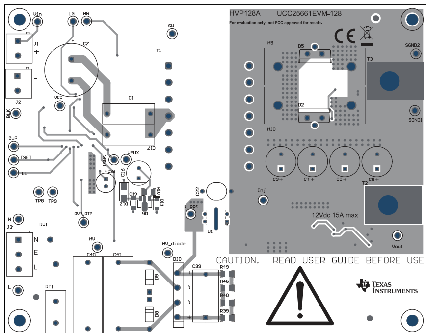
图 4-3. UCC25661EVM-128 (顶视图)
