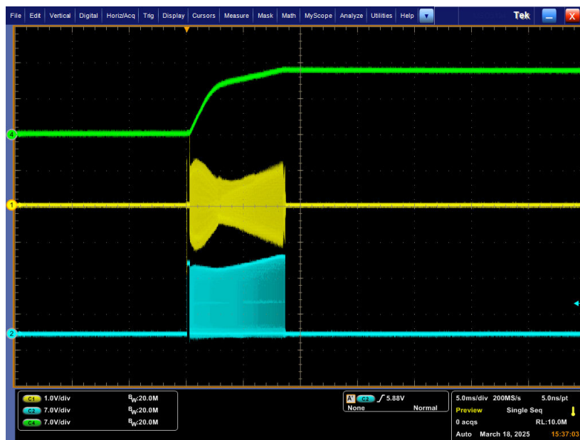
图 3-1. 无负载 (0A) 启动 ( Ch1 = ISNS ; Ch2 = LO ; Ch4 = V_{OUT} )
