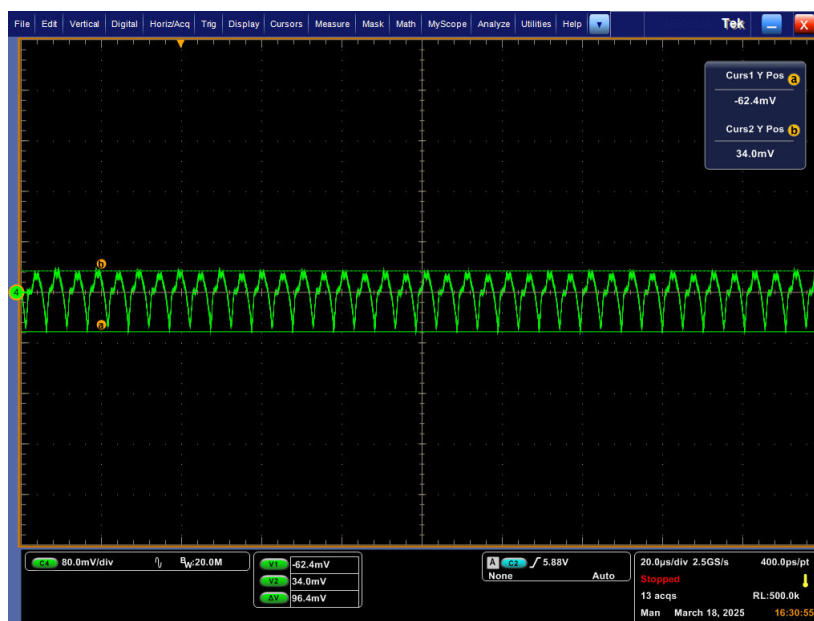
图 3-7. 满载 (15A) 输出纹波 (Ch4 = V_{OUT} )
