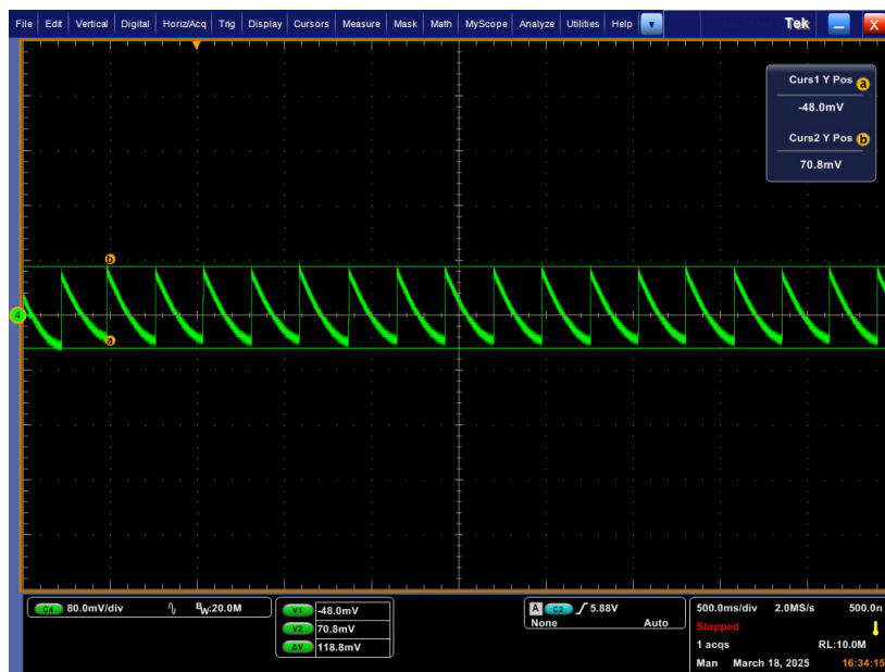
图 3-6. 无负载 (0A) 输出纹波 (Ch4 = V_{OUT} )
