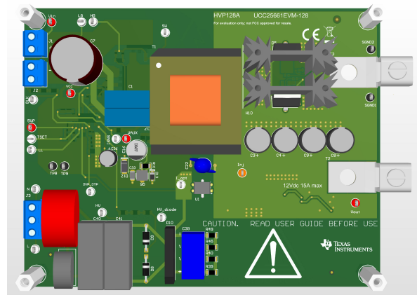
UCC25661EVM-128 180W LLC 谐振直流/直流转换器 ( 顶视图 )
