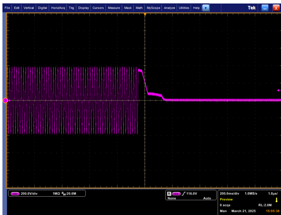
图 3-13. X 电容器放电 ( Ch1 = X 电容器、C40 和 C41 两端的电压 )
