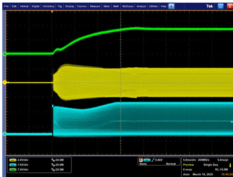
图 3-2. 满载 (15A) 启动 ( Ch1 = ISNS ; Ch2 = LO ; Ch4 = V_{OUT} )
