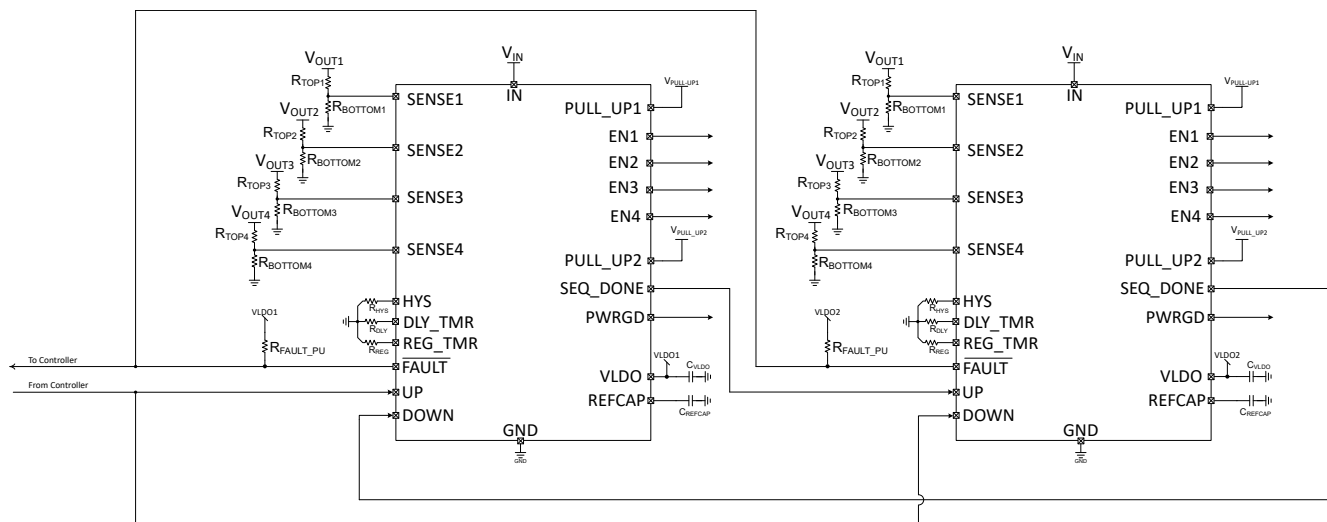
图 1-2. 菊花链配置示例
