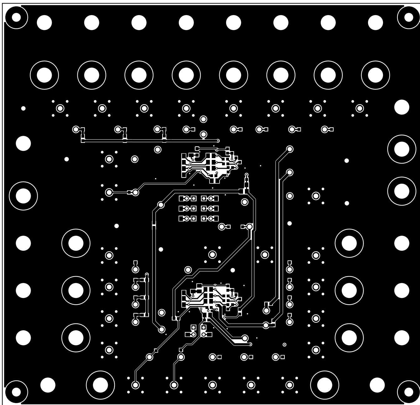
图 4-7. 第 4 层 (底部)
