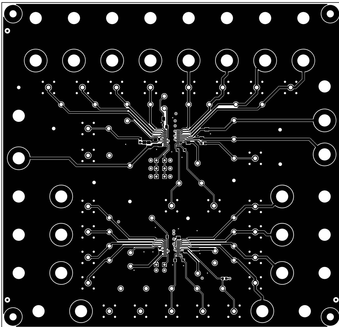
图 4-4. 第 1 层 ( 顶部 )
