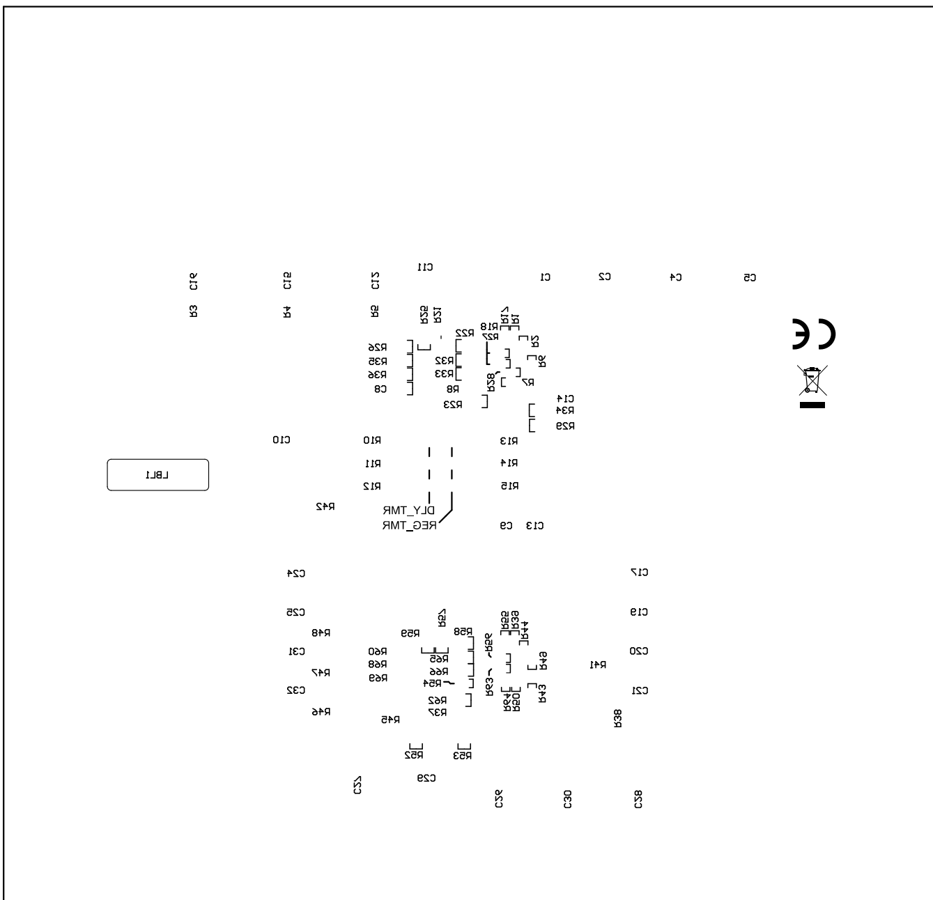
图 4-9. 底层丝印层
