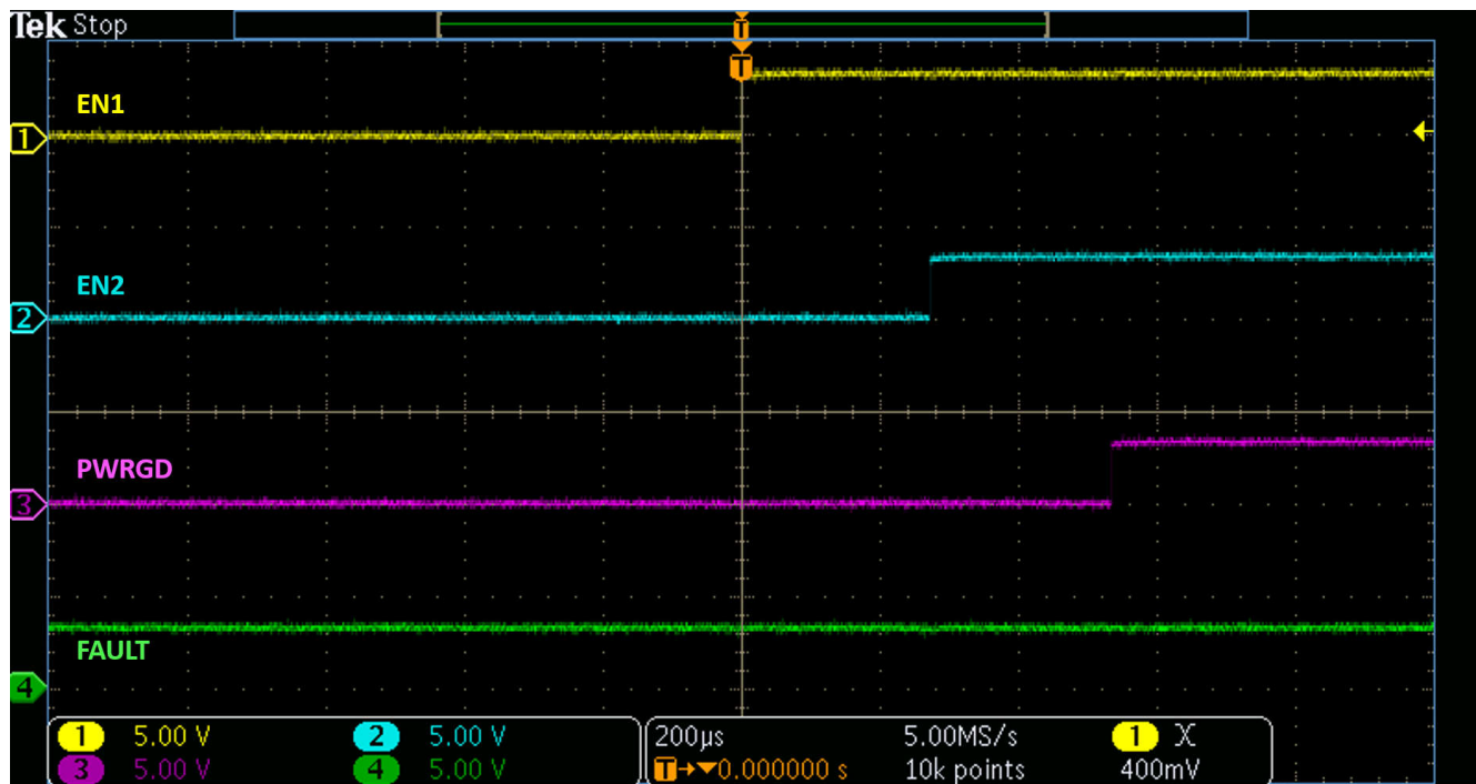
图 3-15. 定序上电
