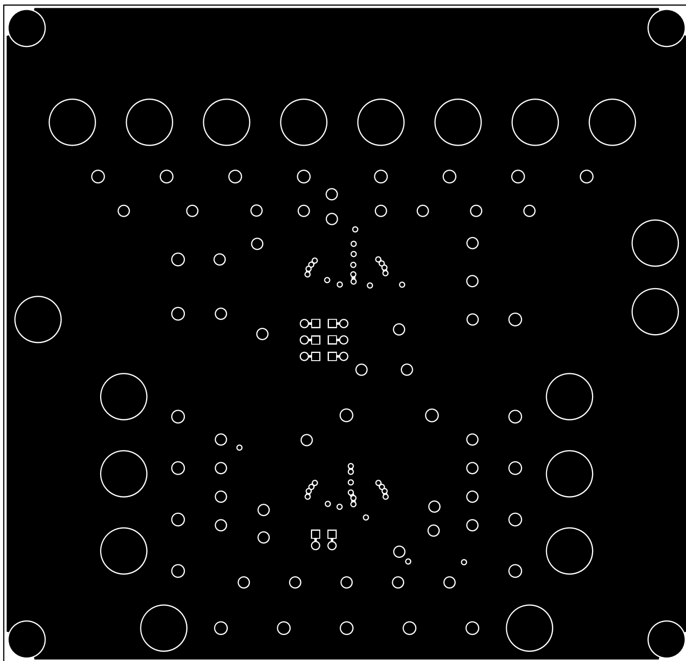
图 4-5. 第 2 层
