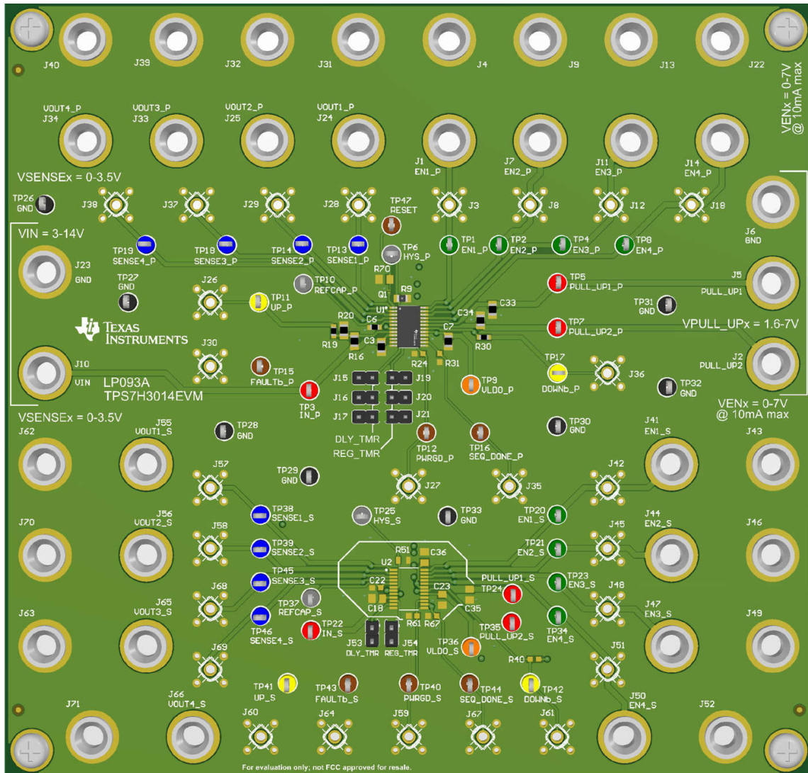
EVM 板
