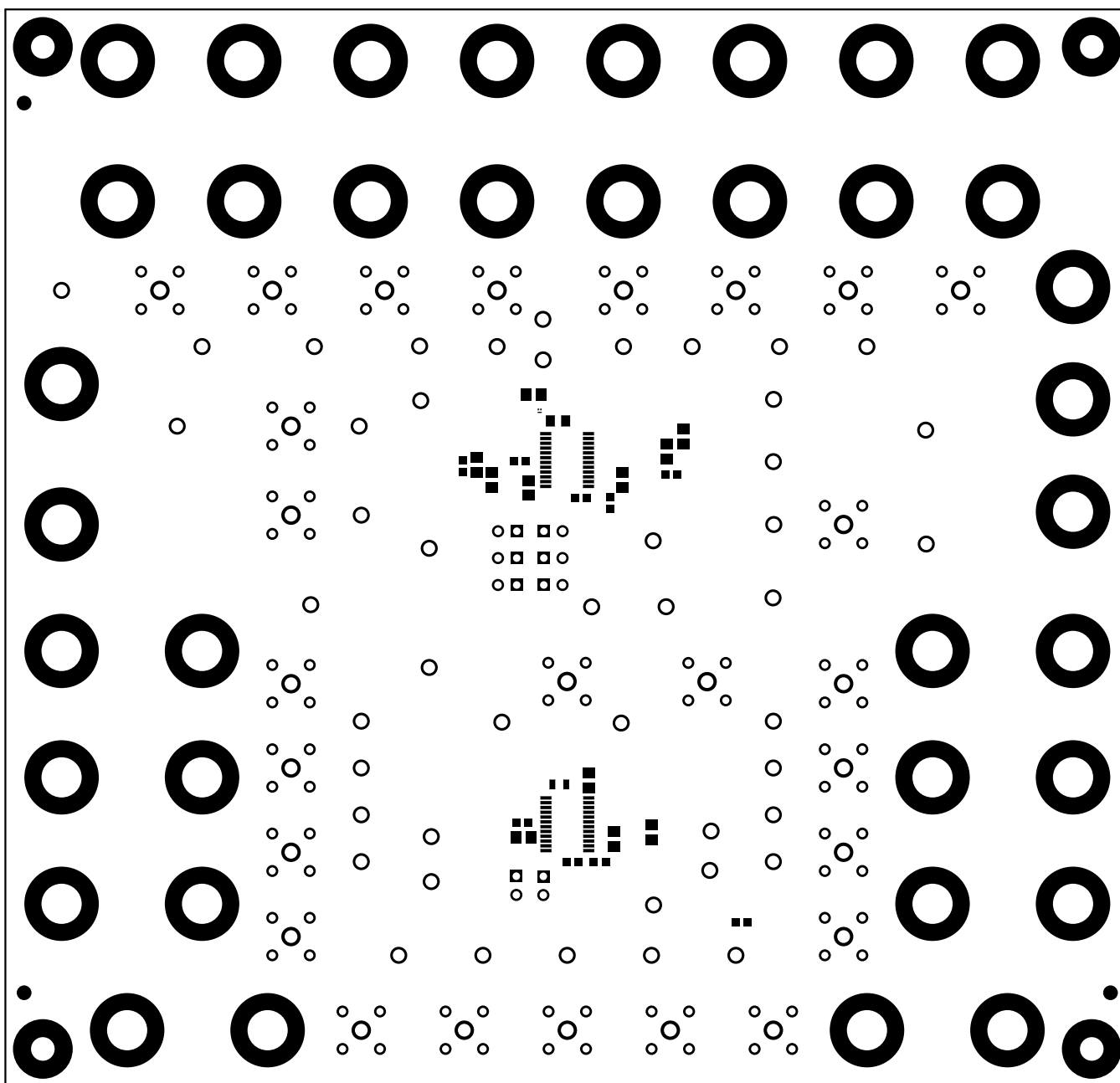
图 4-3. 顶部阻焊层
