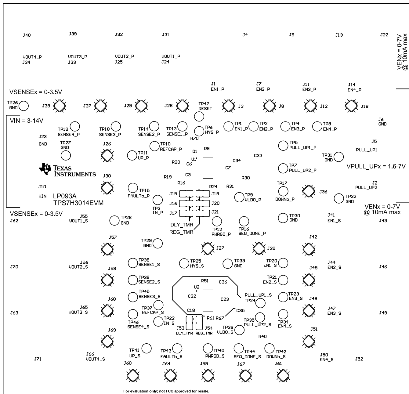
图 4-2. 顶层丝印层
