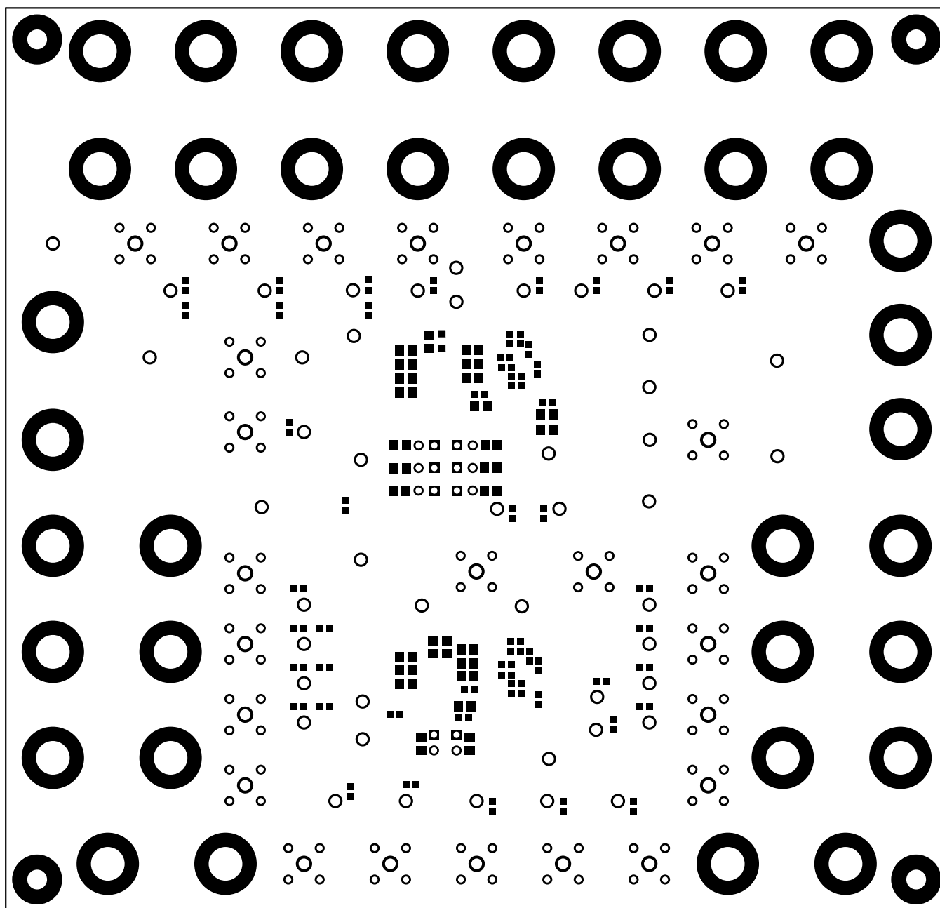
图 4-8. 底部阻焊层
