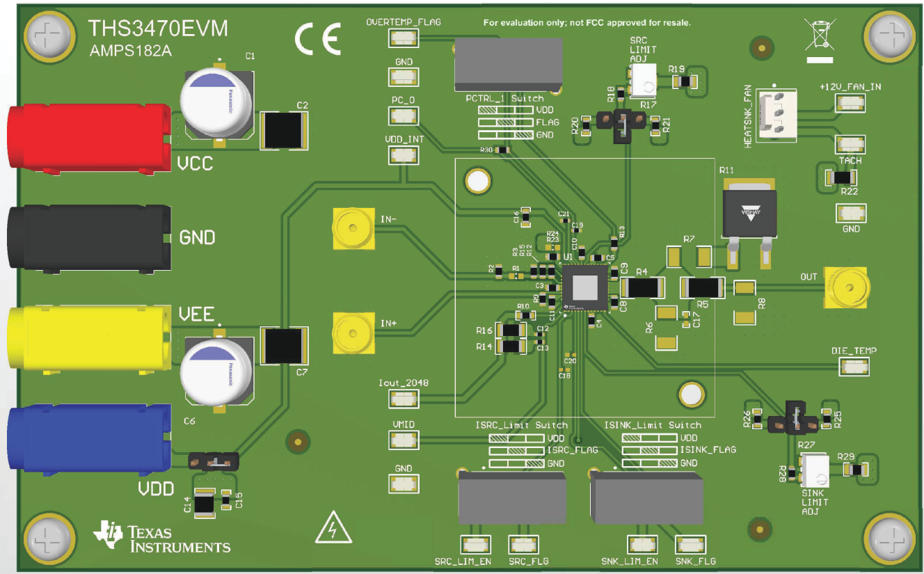
THS3470EVM
