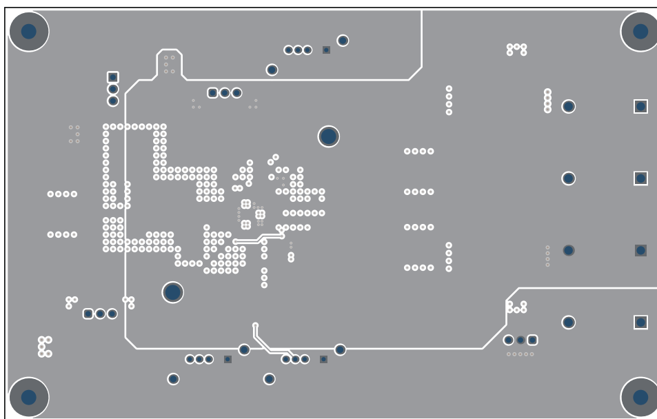
图 4-3. THS3470EVM 底层
