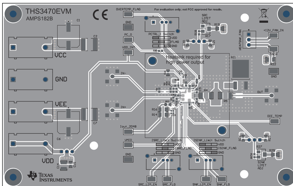
图 4-2. THS3470EVM 顶层
