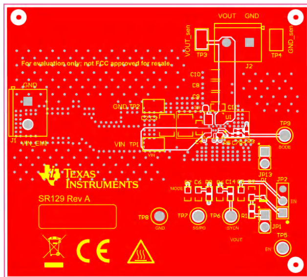
图 3-2. 顶层铜 (顶视图)
