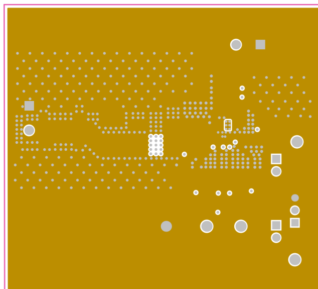
图 3-3. 第 2 层覆铜 (顶视图)
