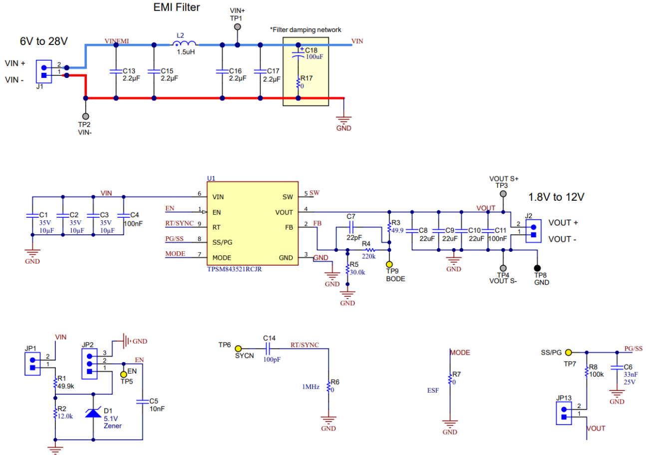
图 3-1. TPSM843521EVM 原理图
