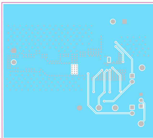
图 3-4. 第 3 层覆铜 (顶视图)
