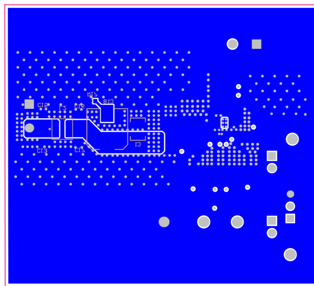
图 3-5. 底层覆铜 (顶视图)
