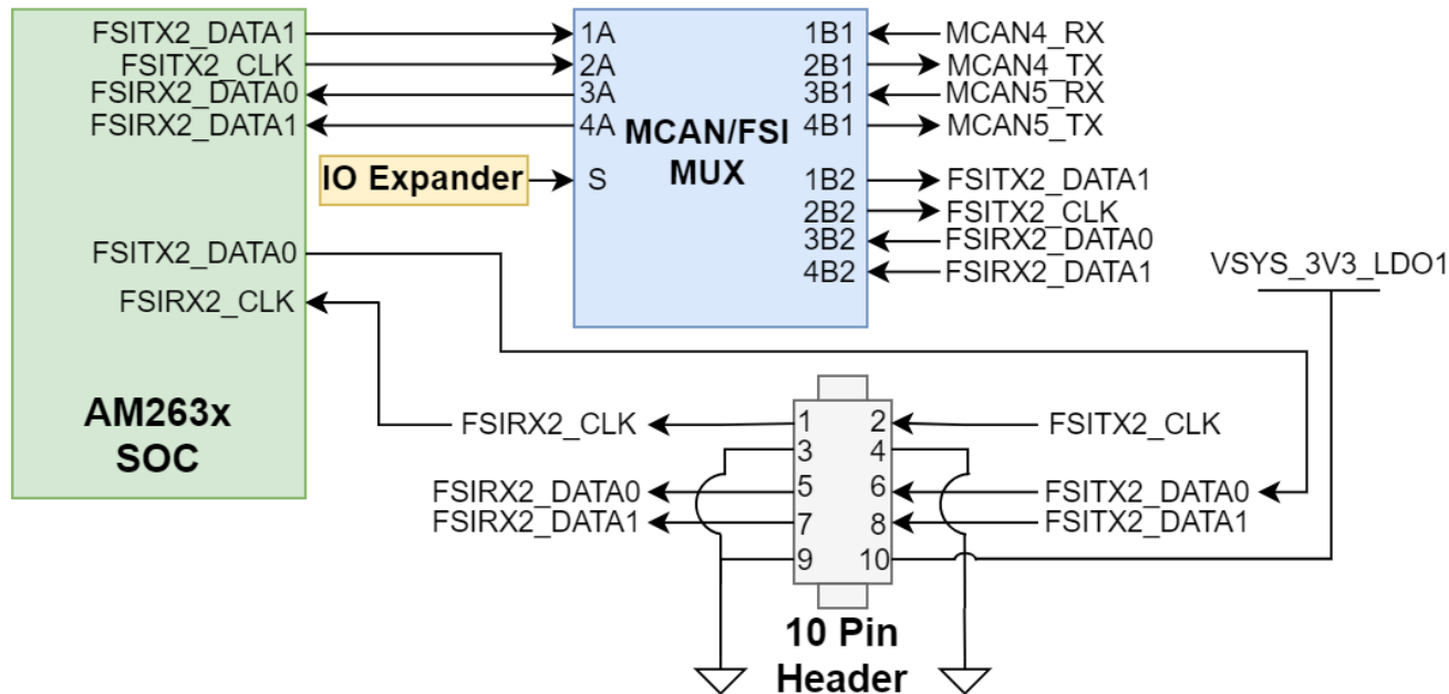
图 2-27. FSI 接头
