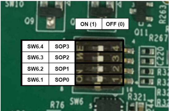
图 2-13. SW6 开关位置
