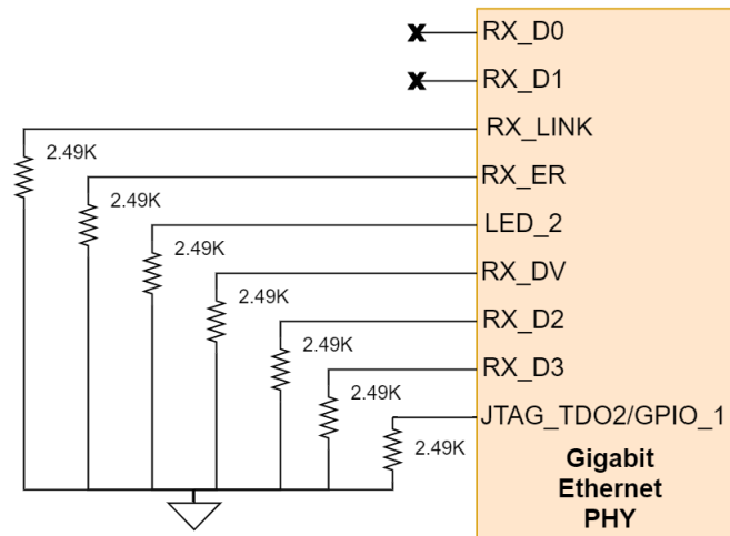
图 2-20. 工业以太网 PHY Strap 配置电阻器
