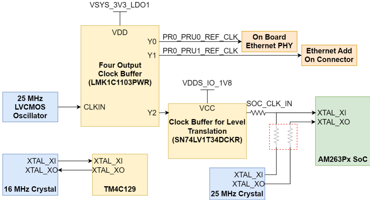
图 2-11. 振荡器时钟树
