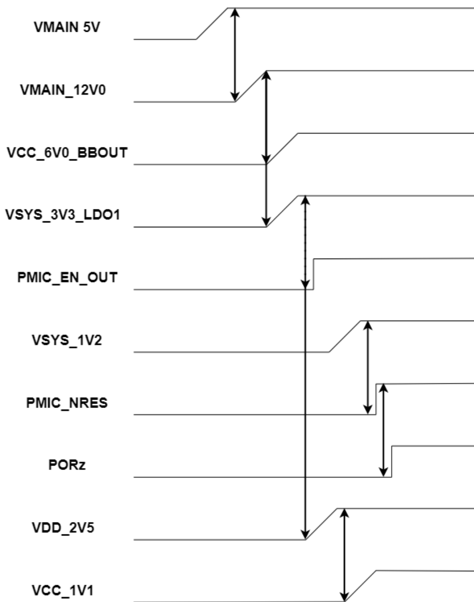
图 2-5. 电源序列图
