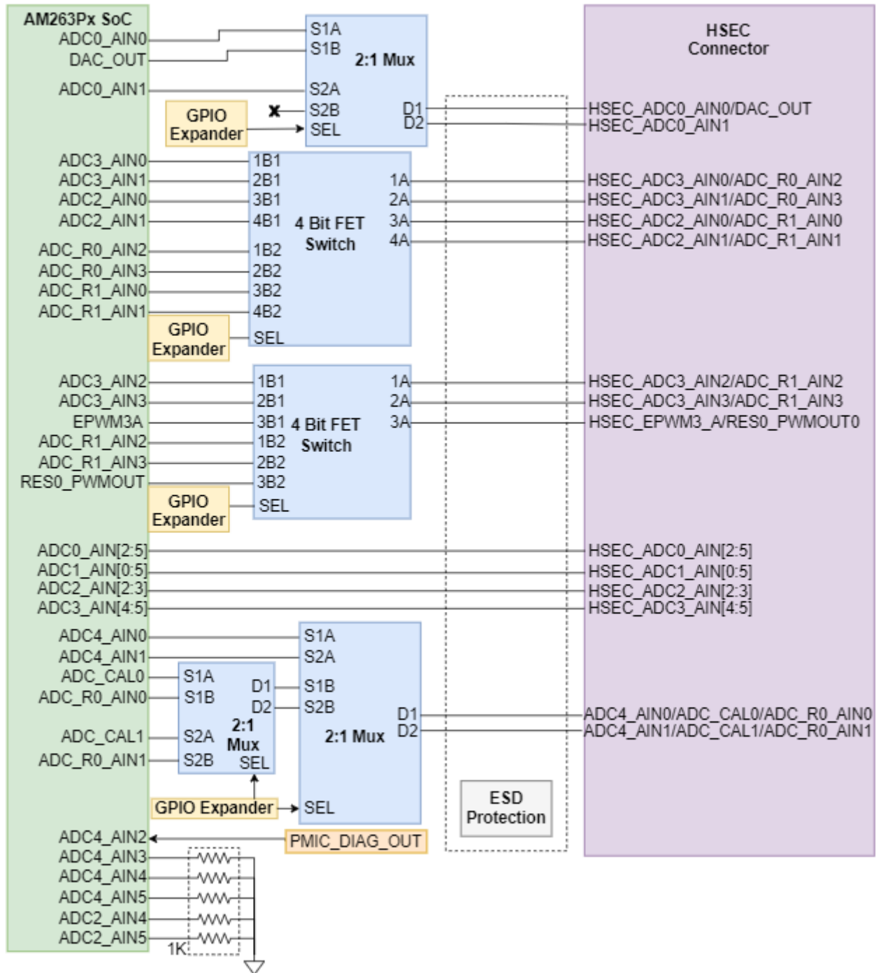
图 2-33. ADC HSEC 连接
