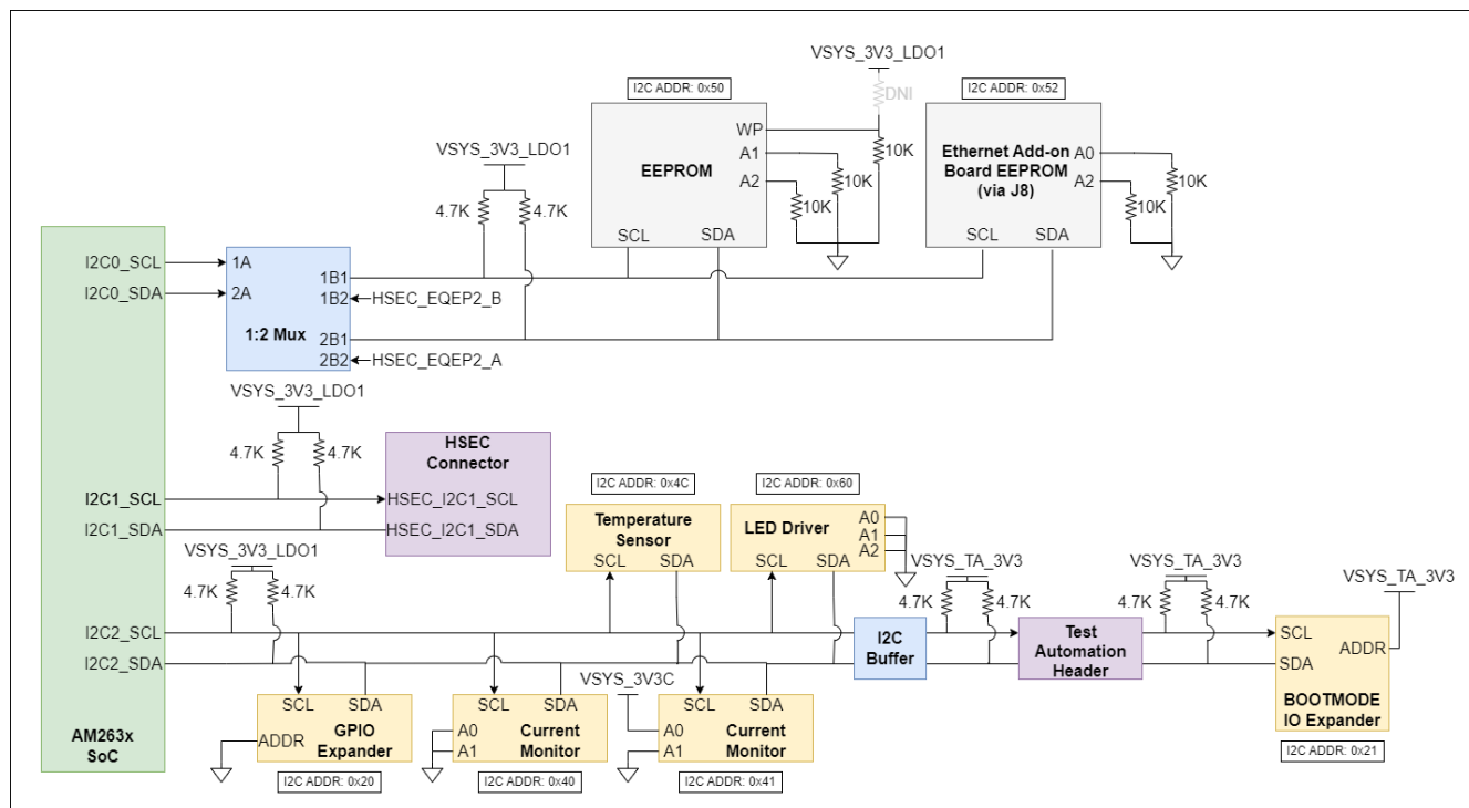
图 2-21. I2C 实例树
