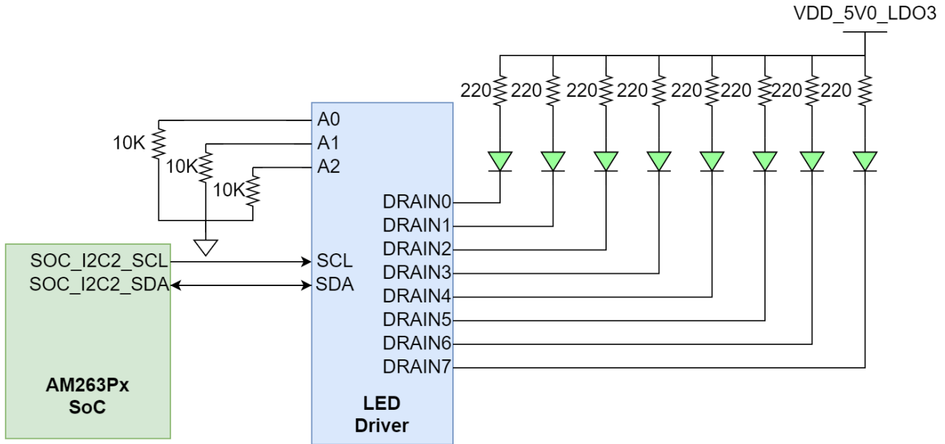
图 2-22. 工业应用 LED 驱动器
