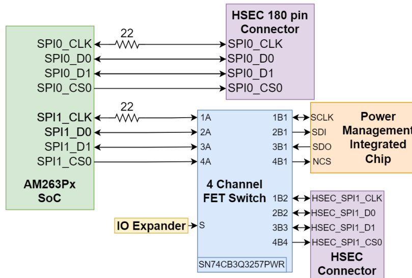
图 2-23. SPI
