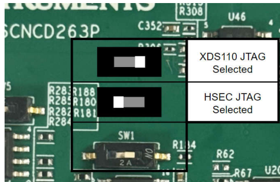
图 2-29. JTAG 路径开关
