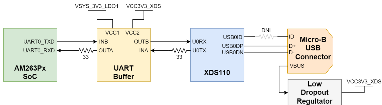
图 2-24. 用于仿真的 UART-USB 电桥
