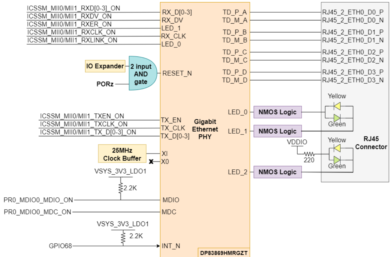
图 2-19. 控制卡板载以太网 PHY
