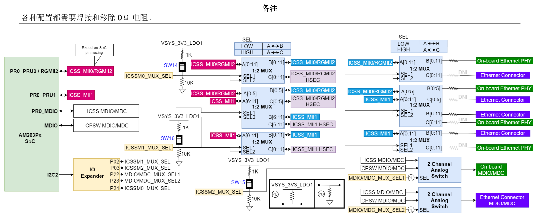
图 2-18. 以太网路由概述
