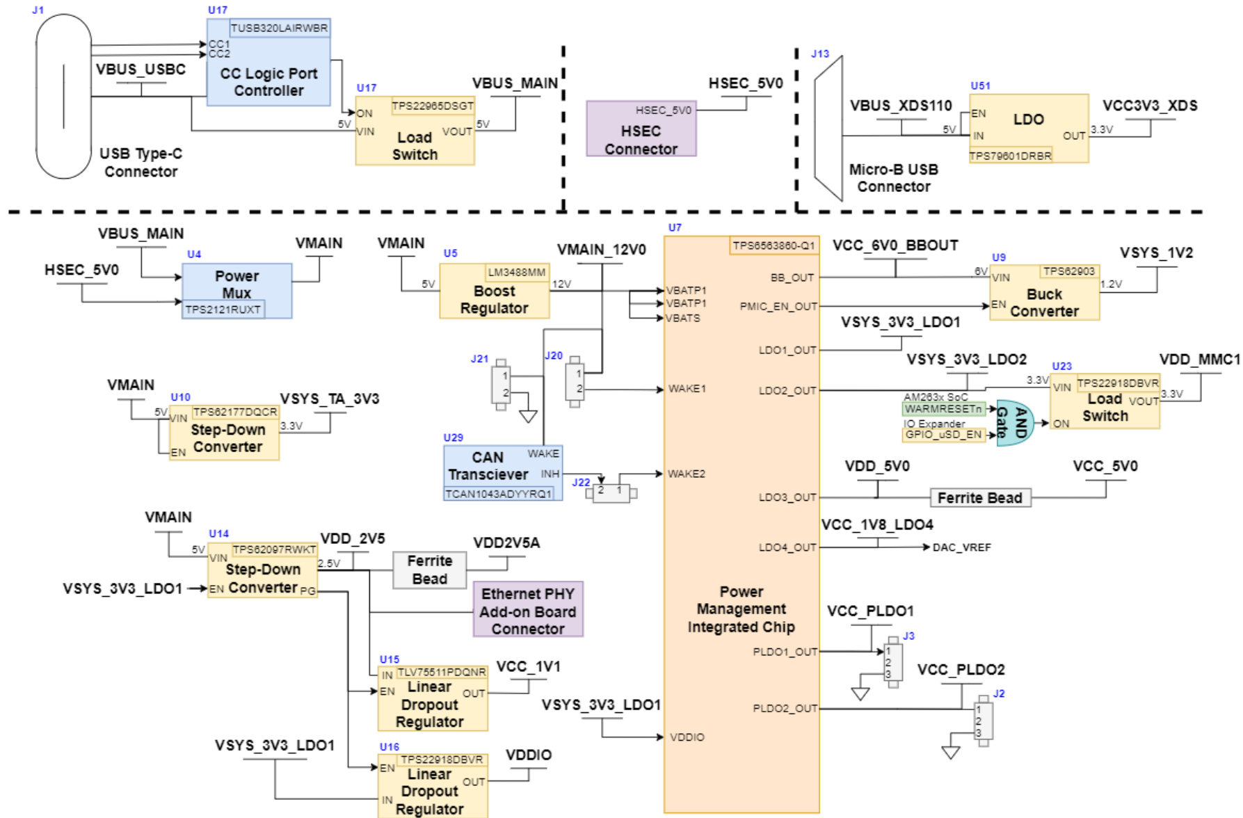
图 2-4. 电源树
