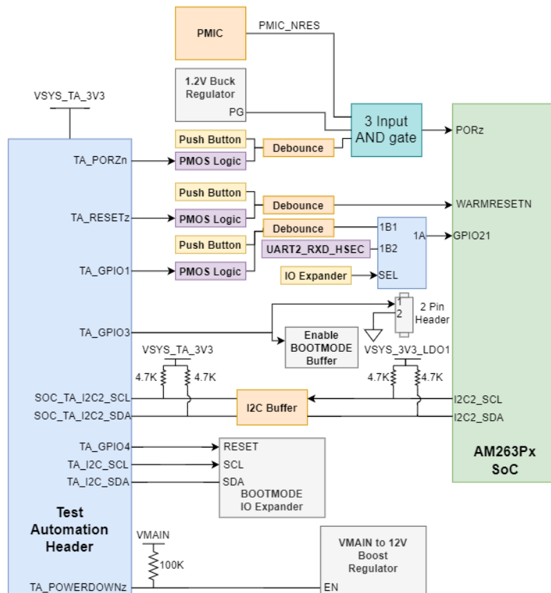
图 2-30. 测试自动化接头
