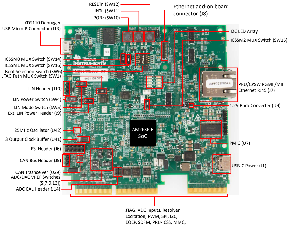
图 1-1. 元件标识 ( 前视图 )
