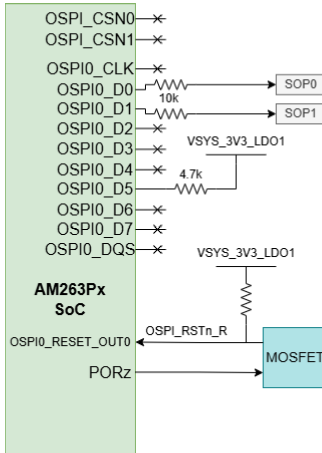
图 2-16. OSPI 接口
