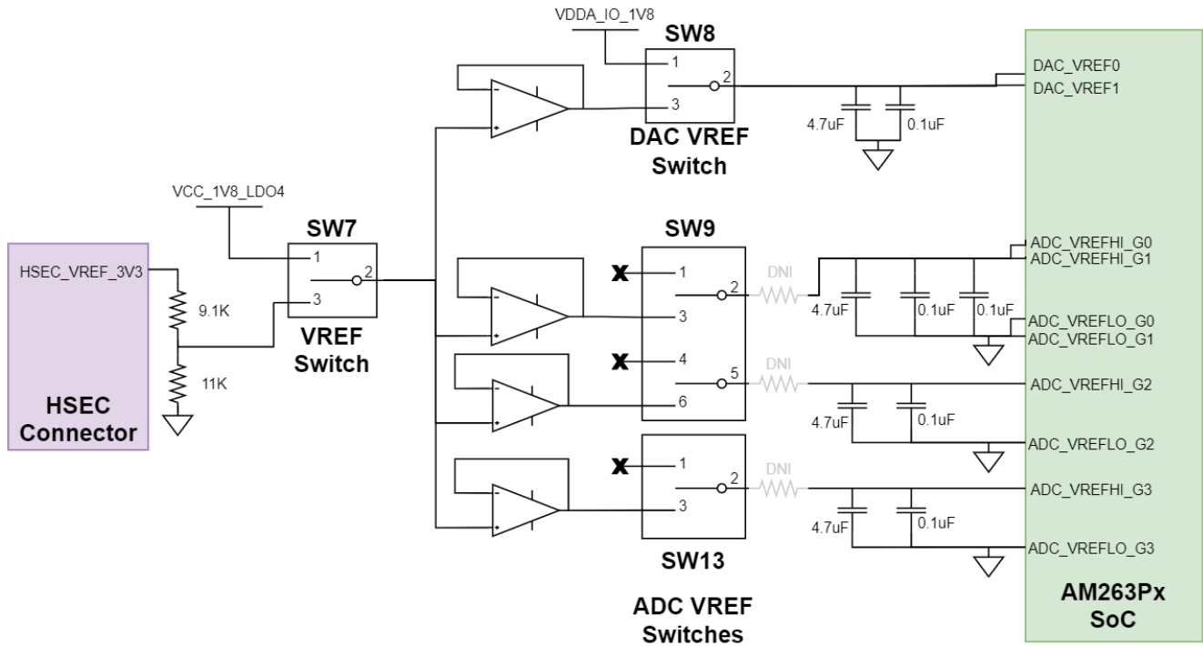
图 2-34. ADC 开关路由
