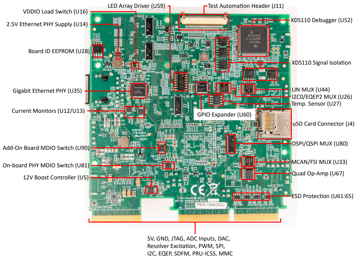
图 1-2. 元件标识 (后视图)
