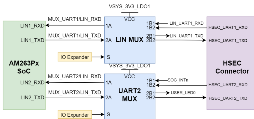
图 2-25. UART 1:2 多路复用到 HSEC
