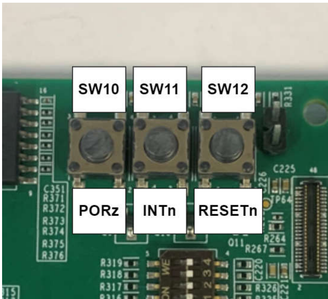
图 2-15. 按钮
