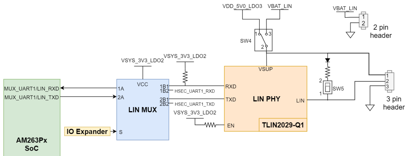
图 2-31. LIN PHY
