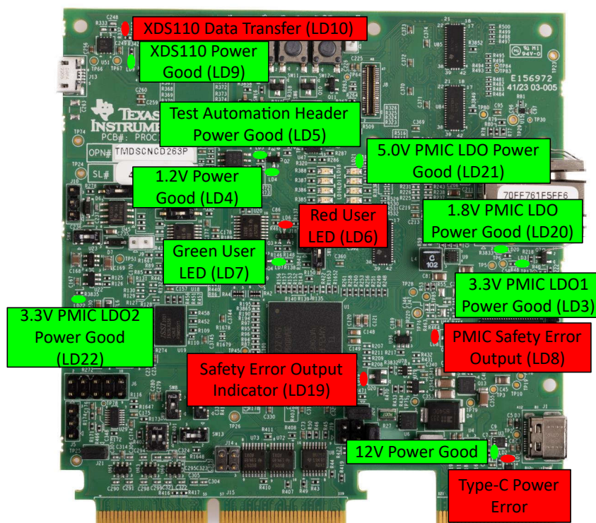
图 2-3. 电源状态 LED
