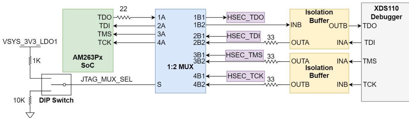
图 2-28. JTAG
