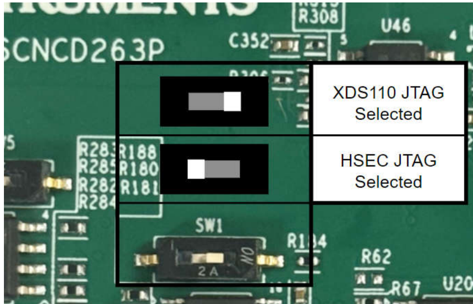
图 2-14. JTAG 路径开关位置
