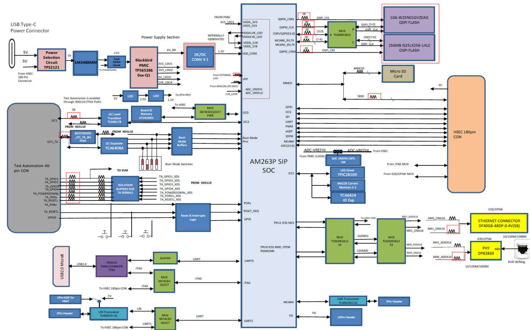
图 2-7. AM263Px-SIP 控制卡方框图
