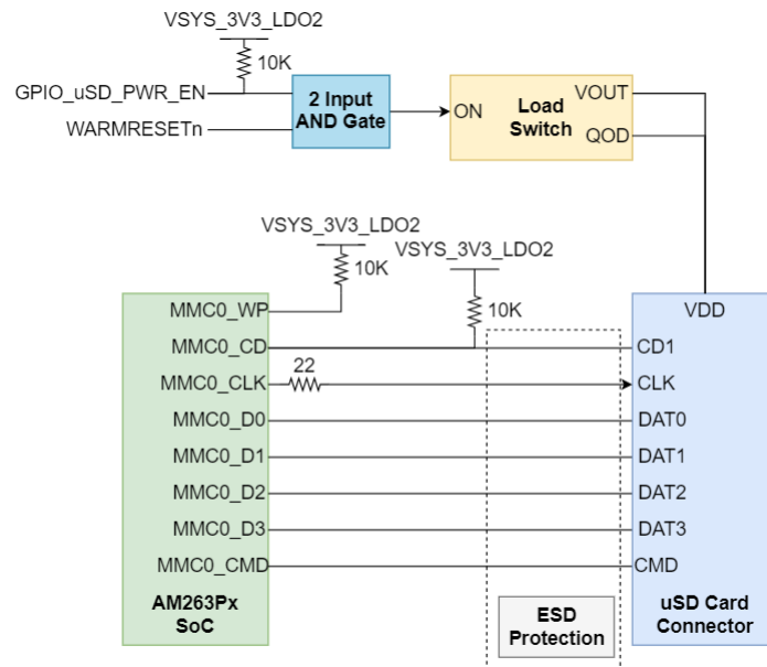
图 2-32. Micro-SD 连接器接口
