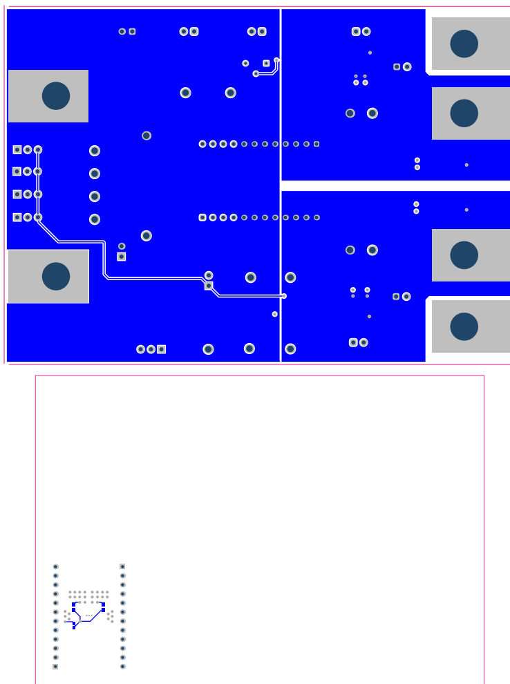
图 4-5. HCXX-BASE-EVM 和 2HC08-MOD-EVM 第四层(顶视图)
