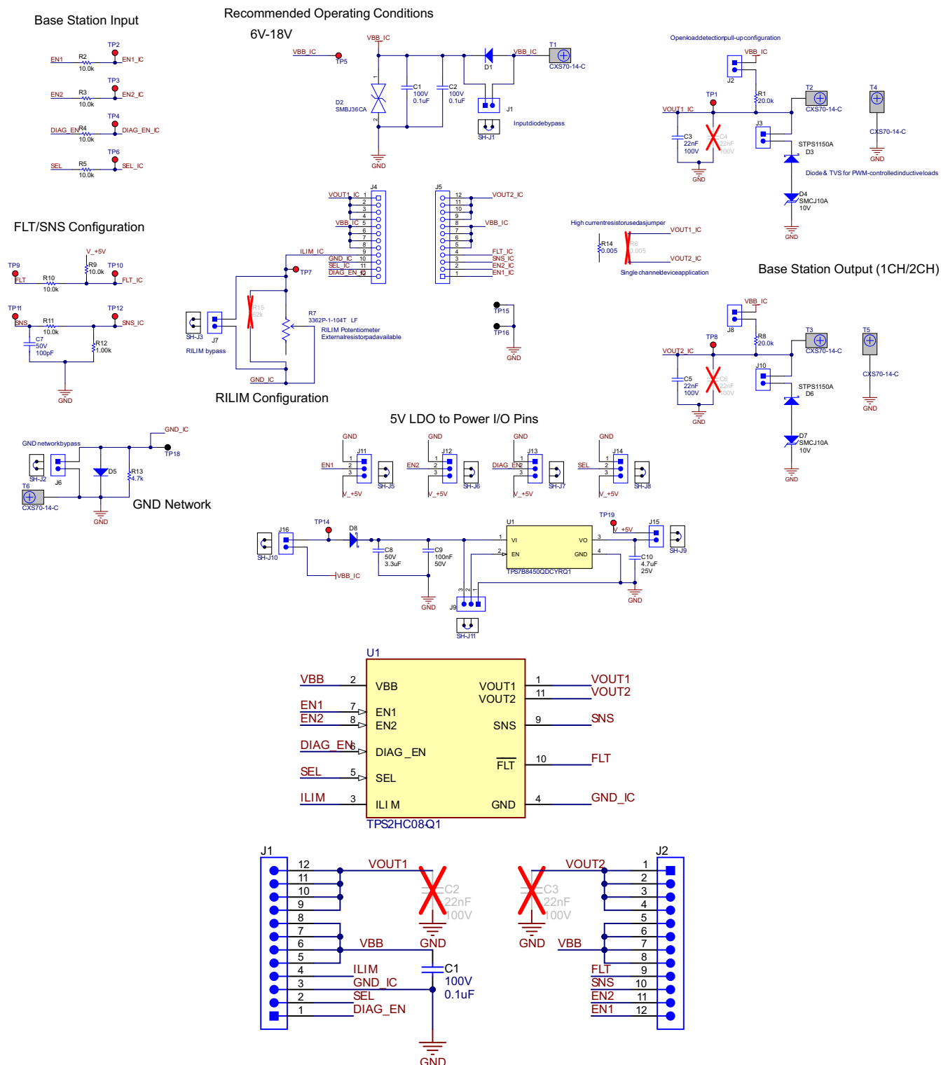
图 4-1. HCXX-BASE-EVM 和 2HC08-MOD-EVM 原理图
