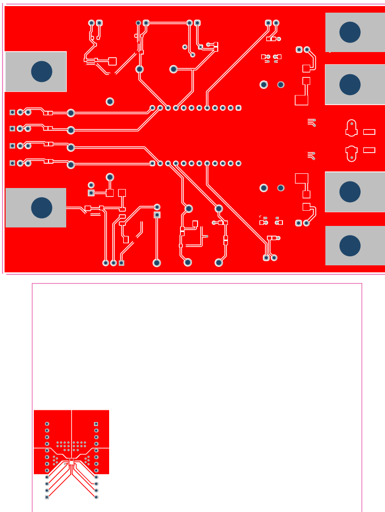
图 4-2. HCXX-BASE-EVM 和 2HC08-MOD-EVM 第一层(顶视图)
