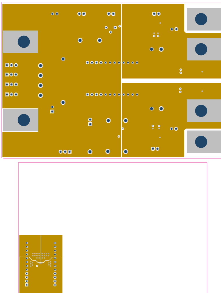
图 4-4. HCXX-BASE-EVM 和 2HC08-MOD-EVM 第三层 VCC (顶视图)
