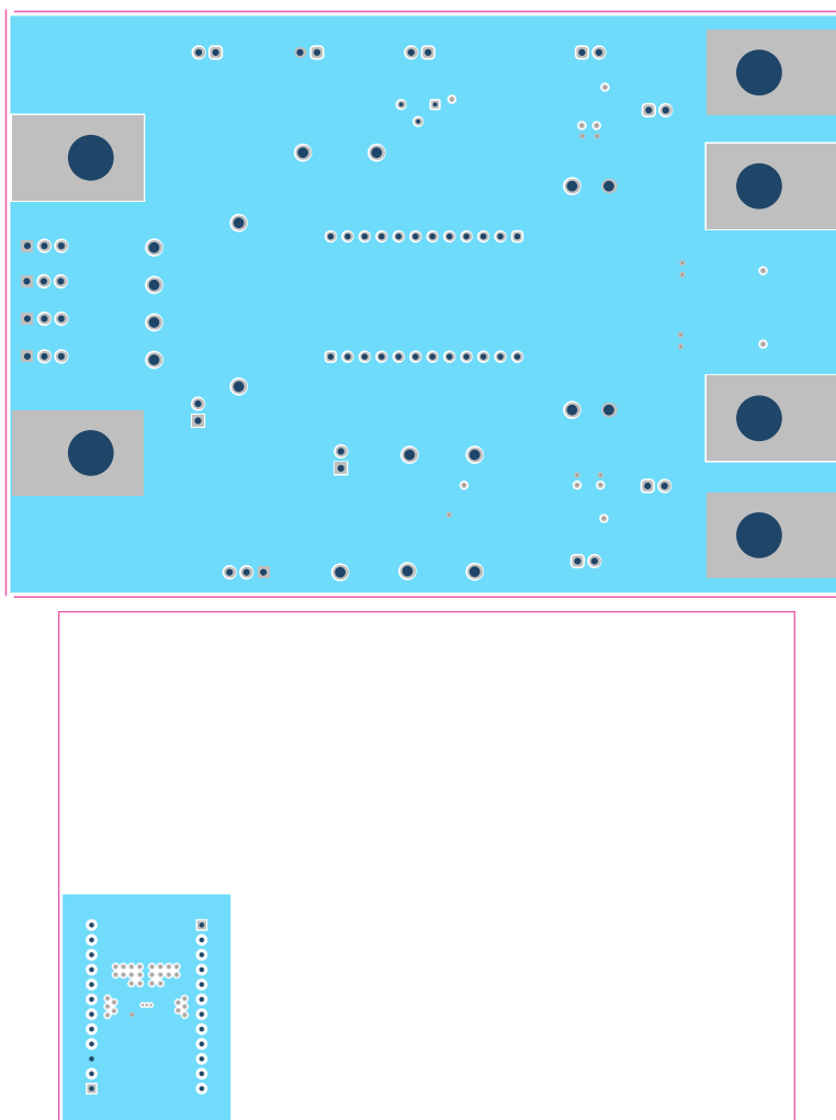
图 4-3. HCXX-BASE-EVM 和 2HC08-MOD-EVM 第二层 GND (顶视图)
