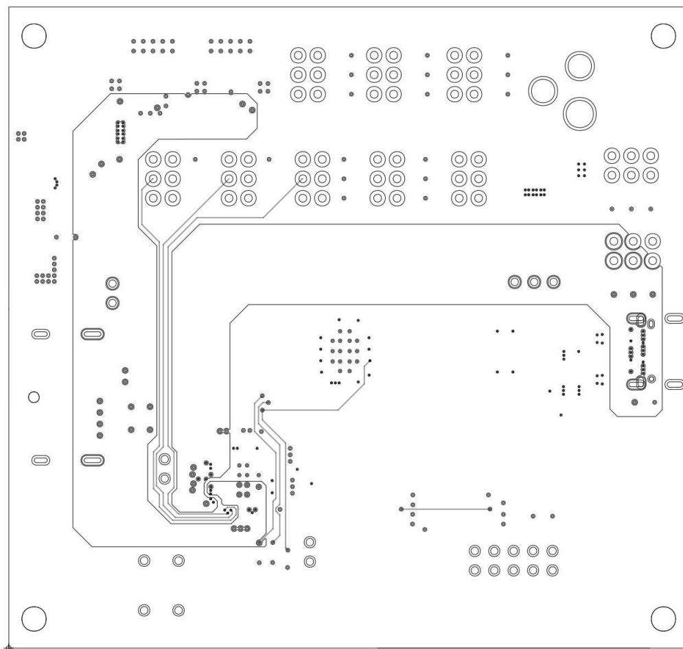
图 4-8. TUSB1146-Q1 EVM PCB 第 4 层 ( 信号 )
