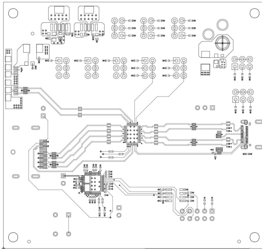
图 4-5. TUSB1146-Q1 EVB PCB 第 1 层 (顶部)
