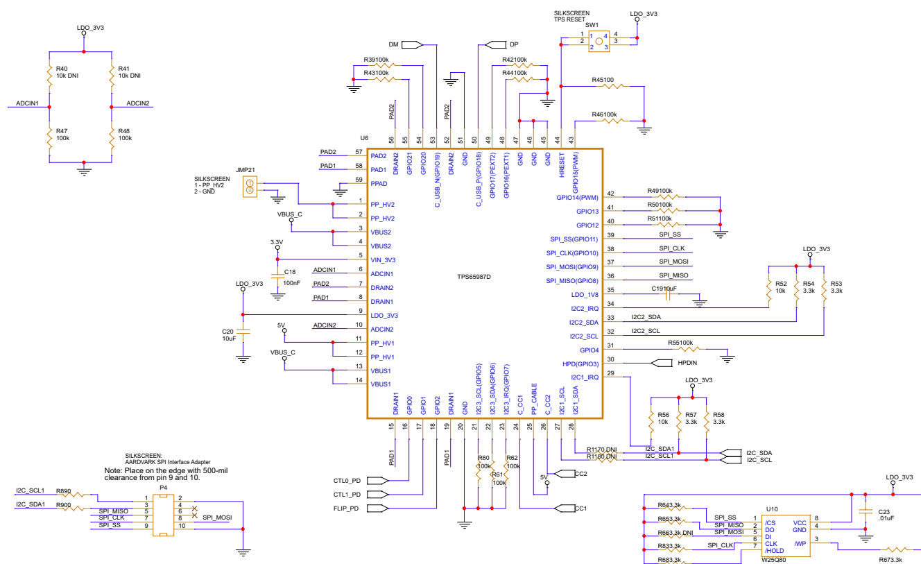
图 4-3. TUSB1146-Q1 EVM 原理图 (第 3 页)
