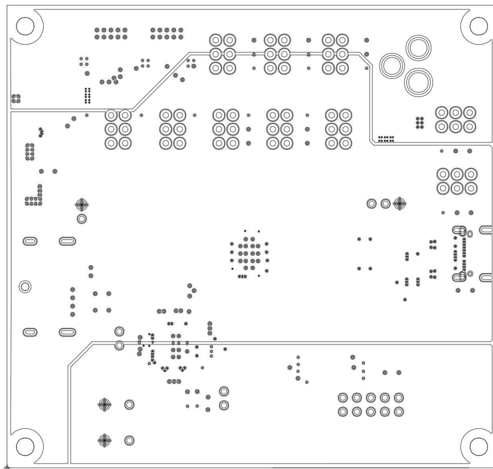
图 4-7. TUSB1146-Q1 EVM PCB 第 3 层 ( 电源 )
