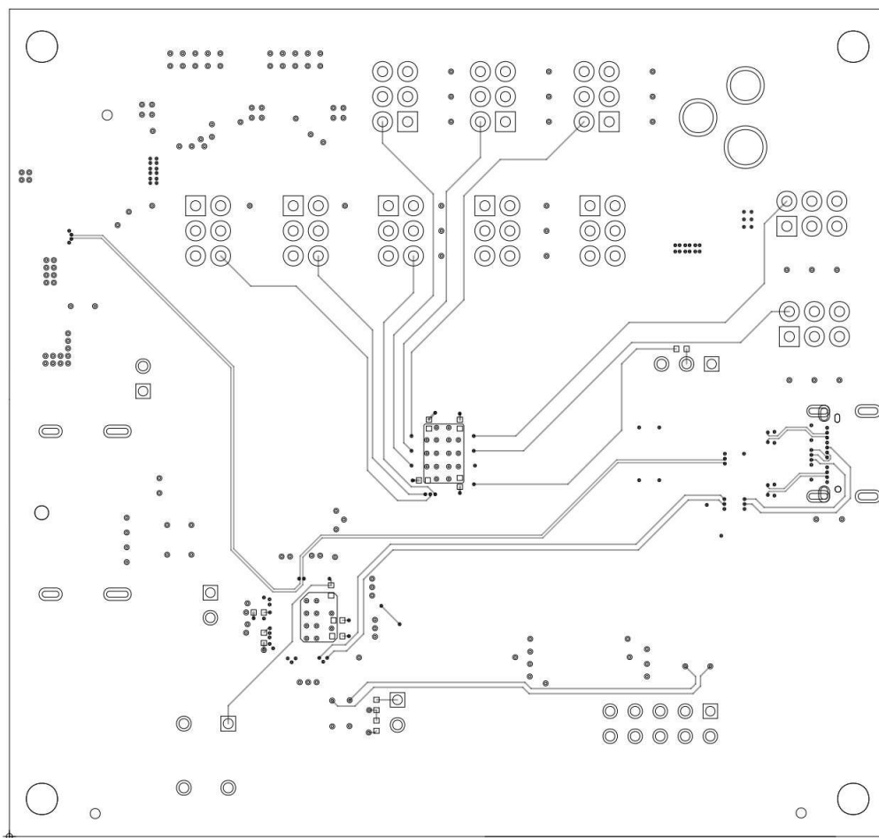
图 4-10. TUSB1146-Q1 EVM PCB 第 6 层 (底部)
