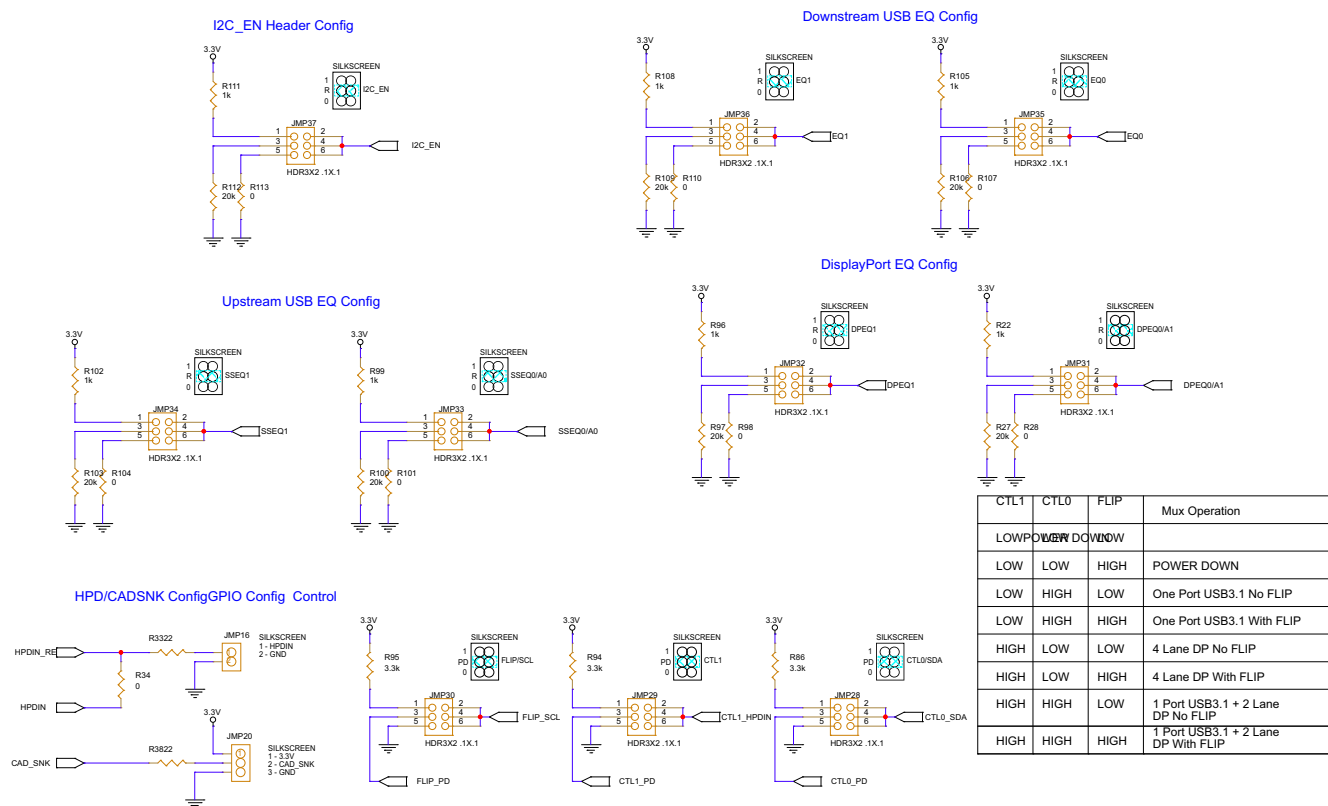
图 4-2. TUSB1146-Q1 EVM 原理图 (第 2 页)
