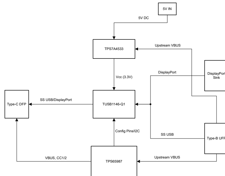
图 1-1. 方框图
