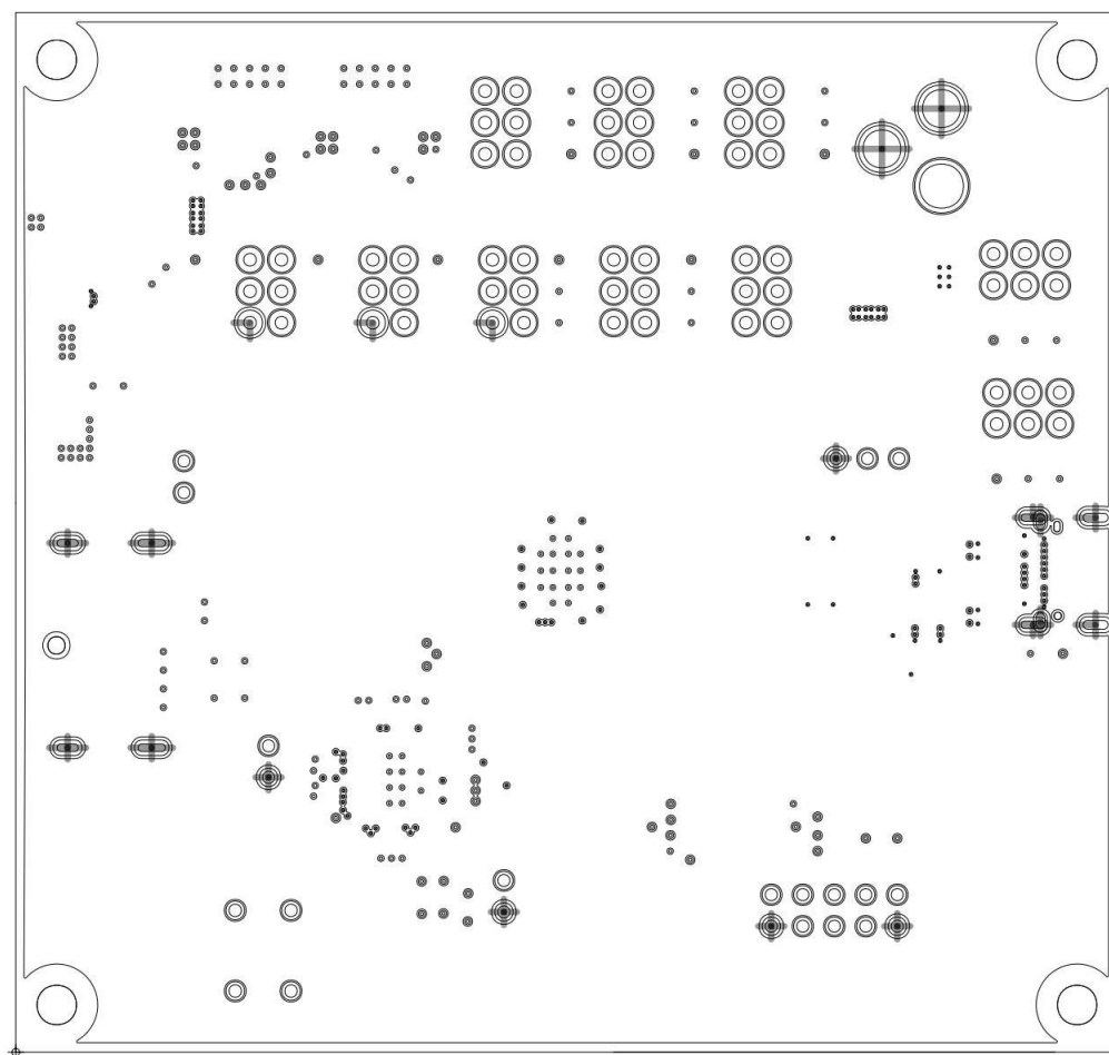
图 4-9. TUSB1146-Q1 EVM PCB 第 5 层 (GND)
