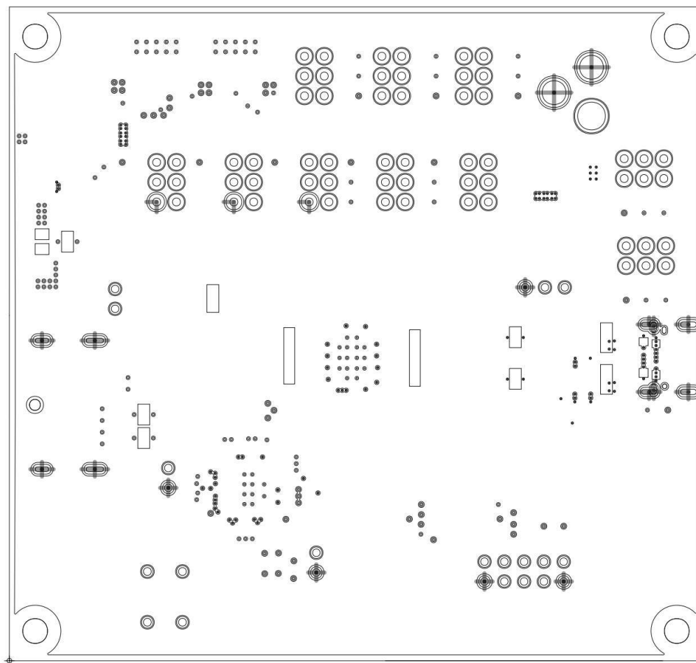
图 4-6. TUSB1146-Q1 EVM PCB 第 2 层 (GND)
