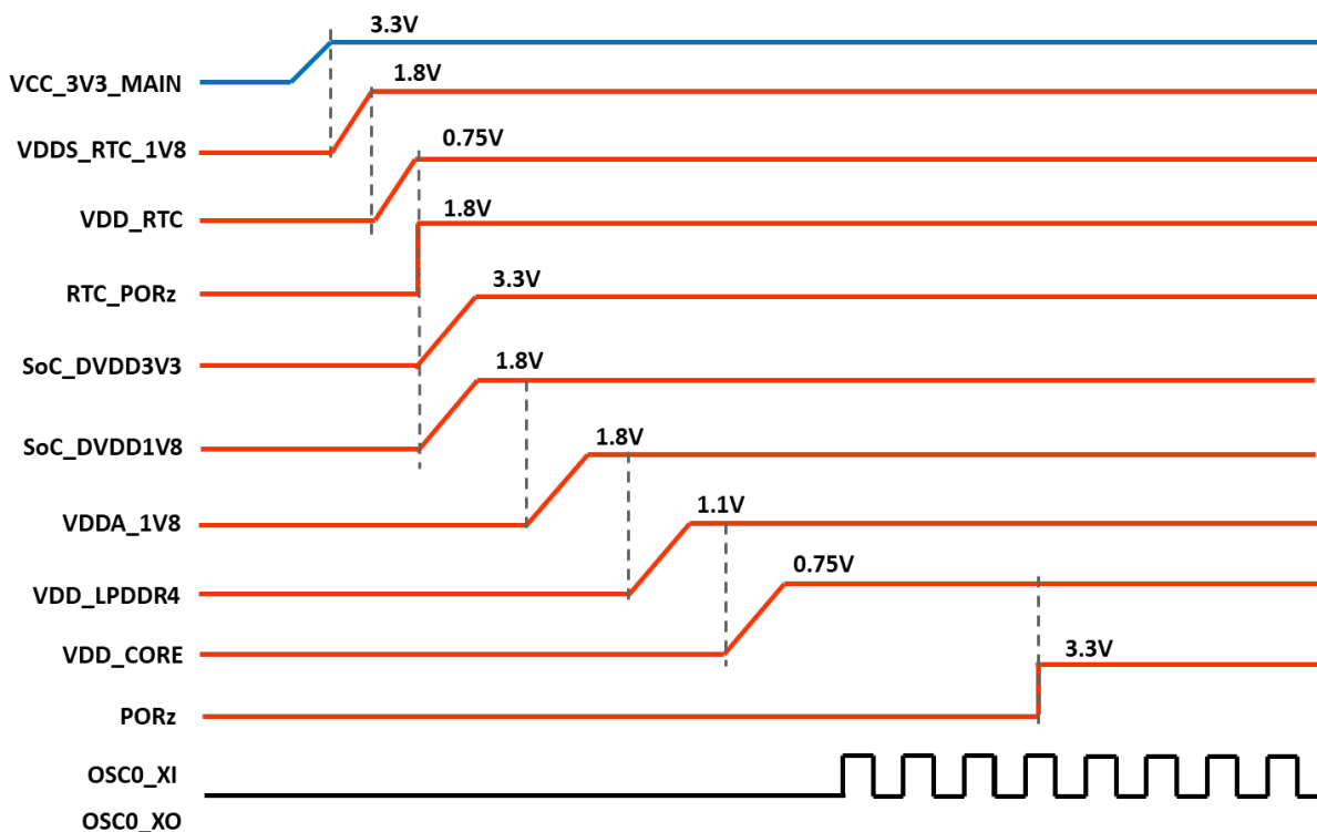
图 2-32. 电源序列
