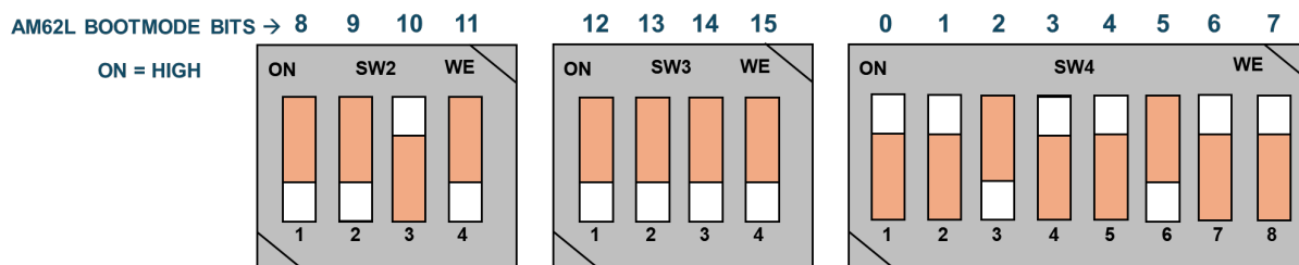
图 2-7. GPMC NAND/USB 备份的引导模式开关配置
