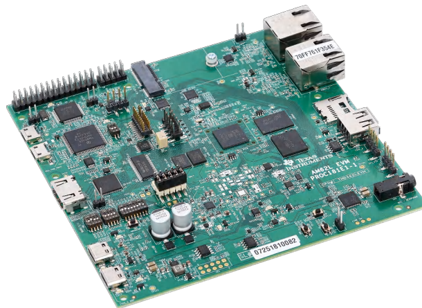
TMDS62LEVM 硬件板
