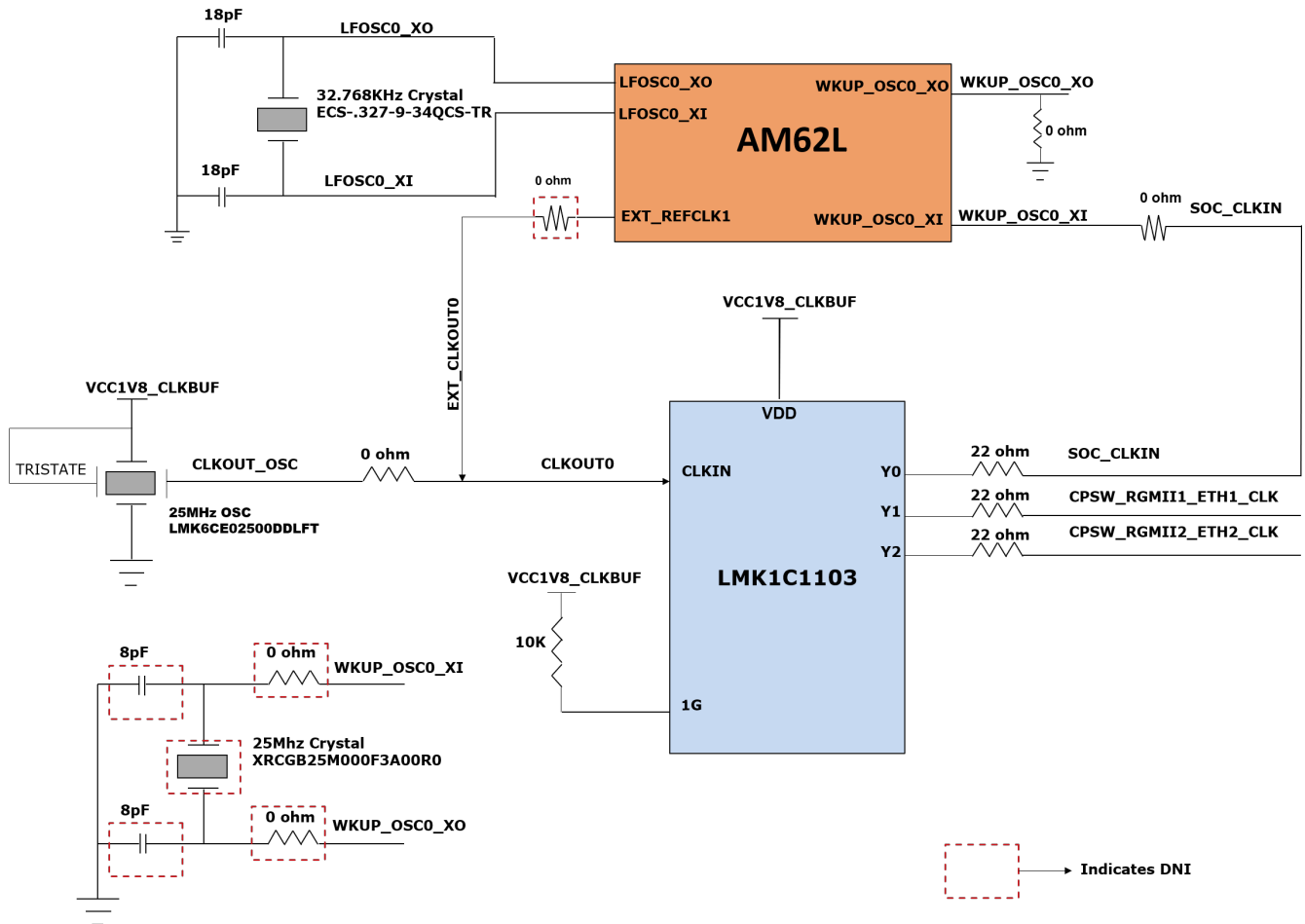
图 2-33. 时钟架构
