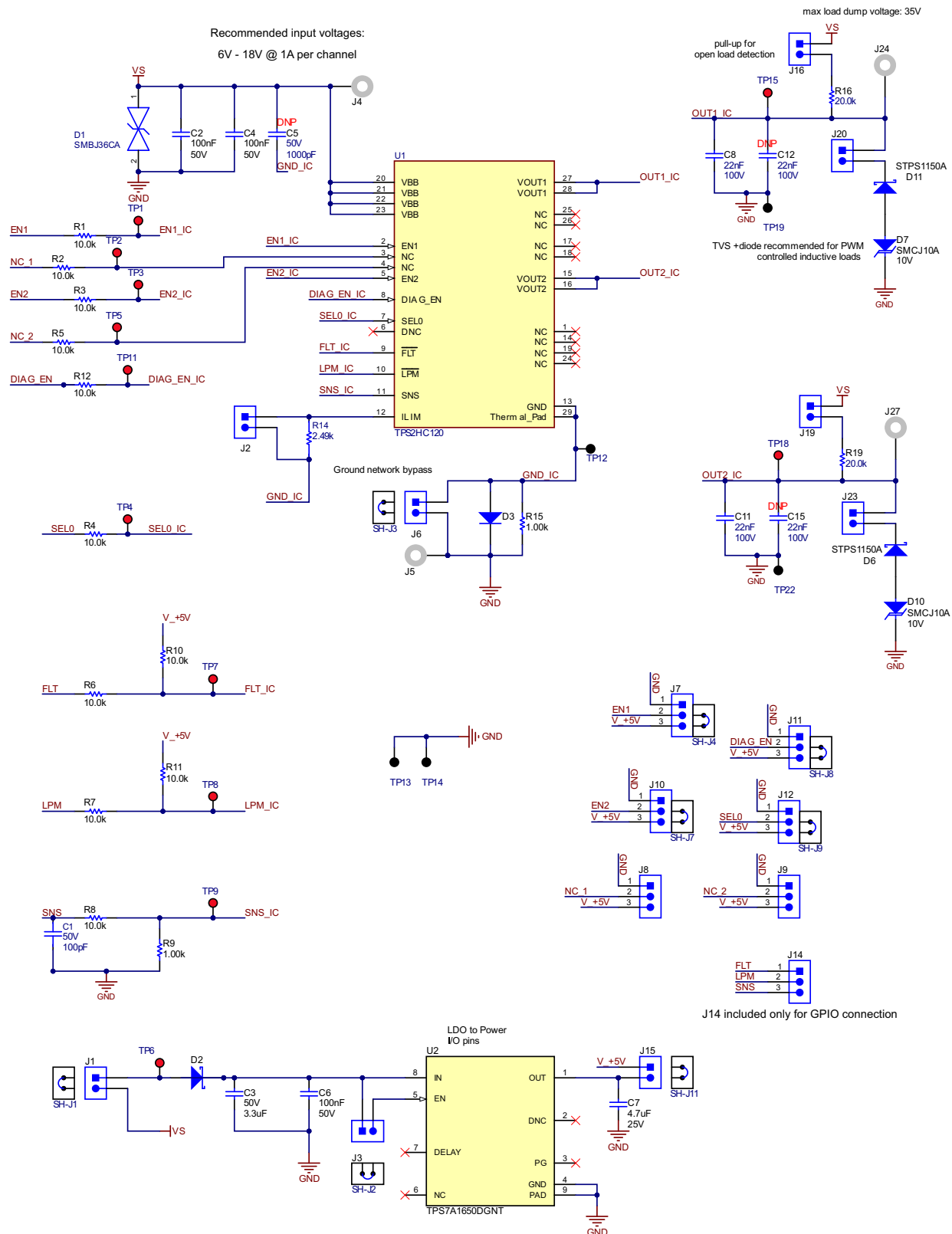
图 4-1. TPS2HC120EVm 原理图
