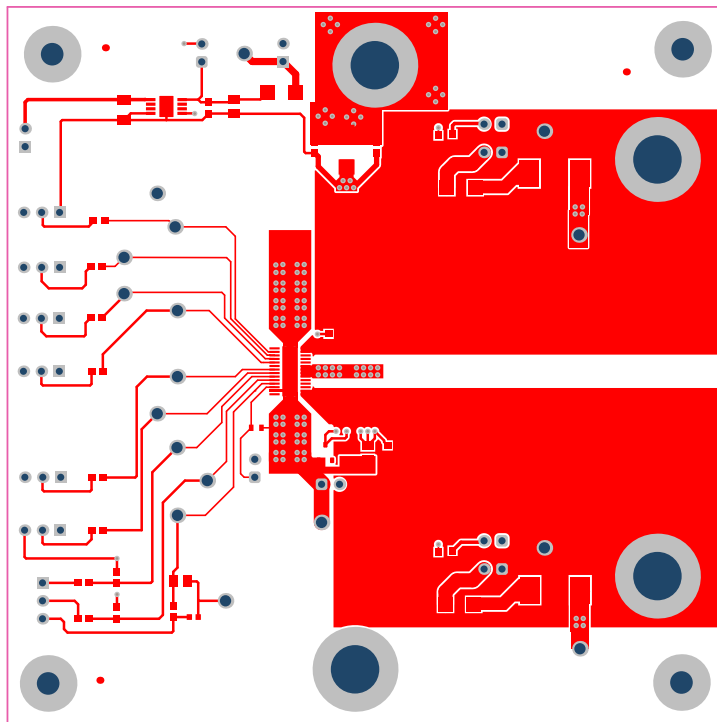
图 4-2. TPS2HC120EVM 第一层 ( 顶视图 )
