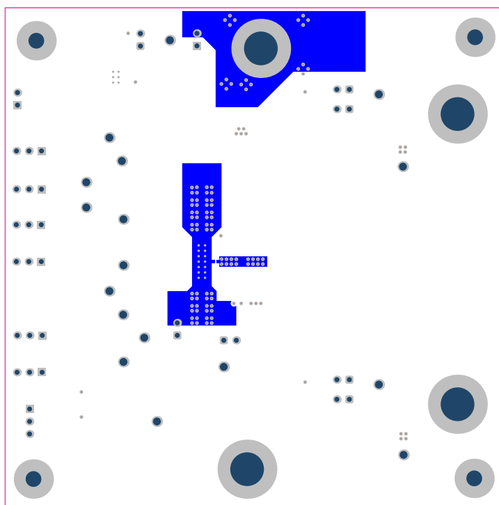
图 4-5. TPS2HC120EVM 第四层 (顶视图)
