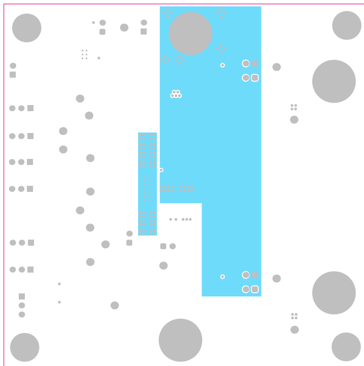
图 4-4. TPS2HC120EVM 第三层 VCC (顶视图)
