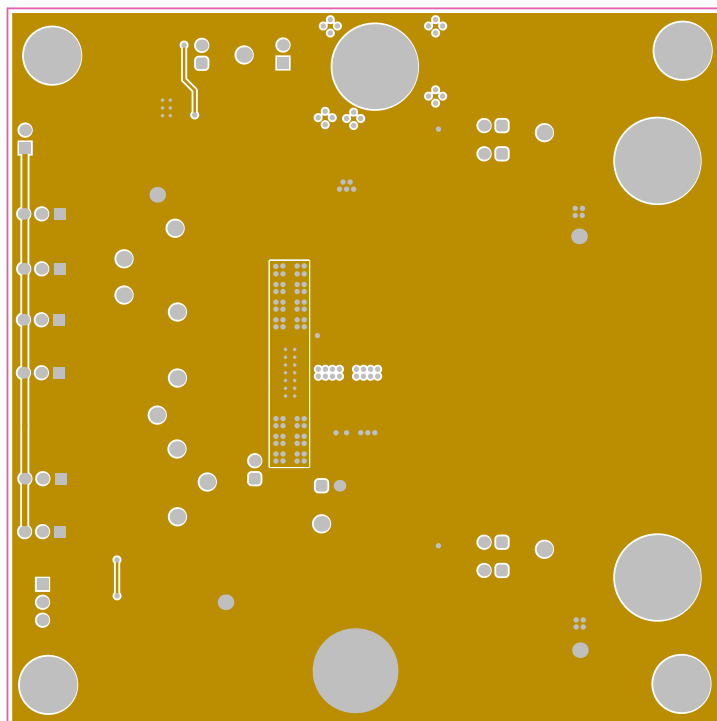
图 4-3. TPS2HC120EVM 第二层 GND ( 顶视图 )
