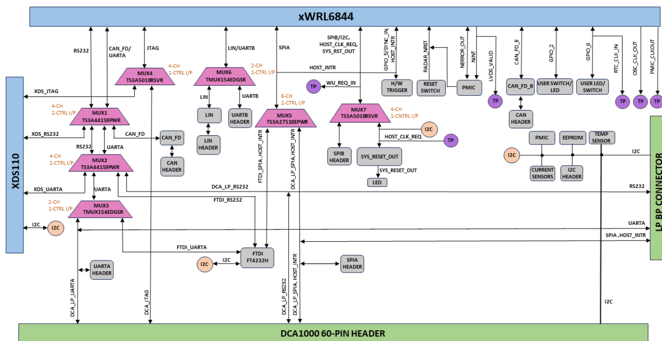
图 3-9. EVM 中的功能多路复用选项
