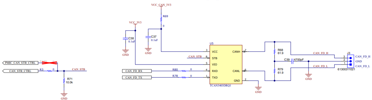
图 3-23. EVM 中使用的 CAN FD PHY
