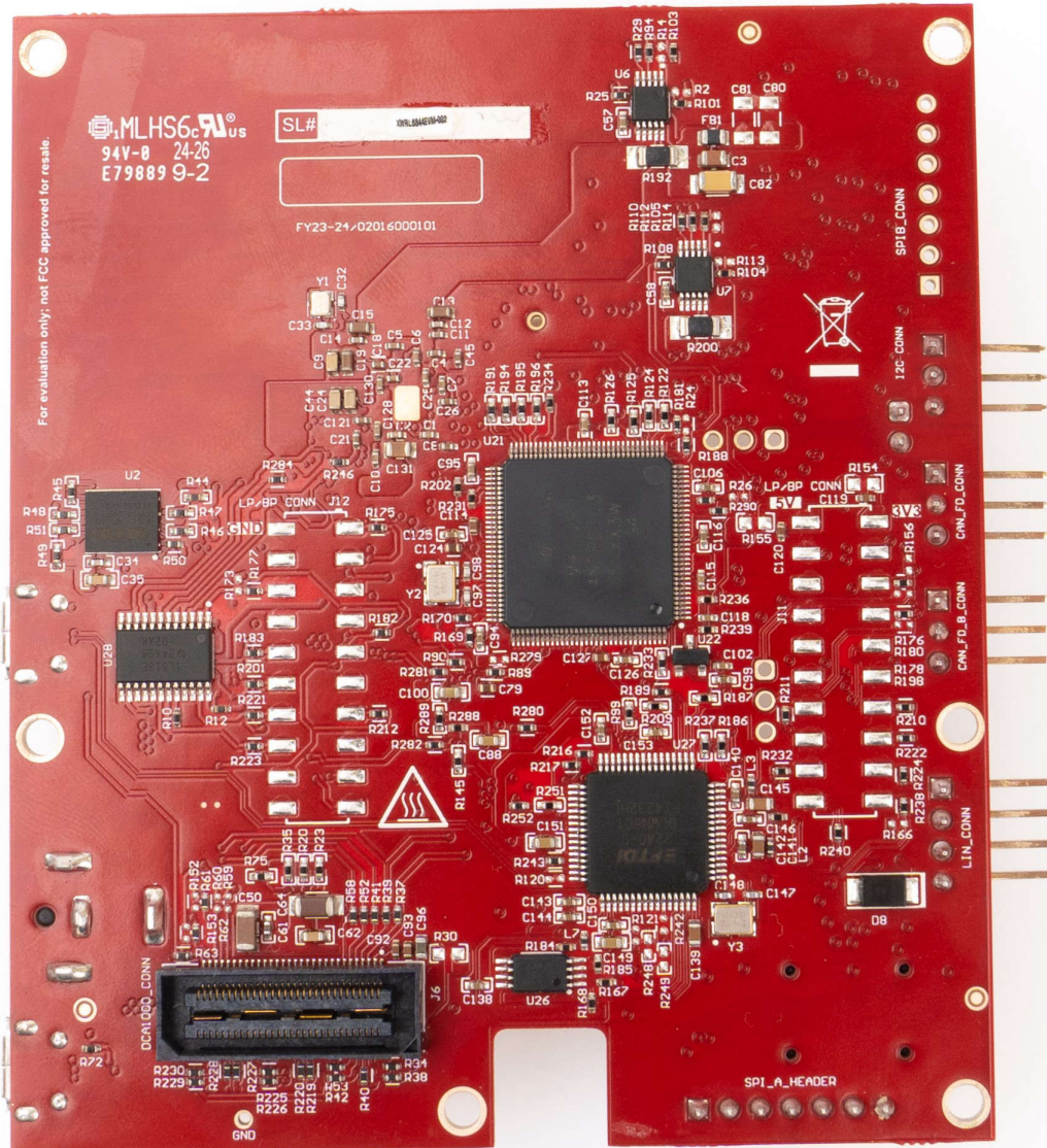
图 3-2. xWRL6844EVM (底视图)
