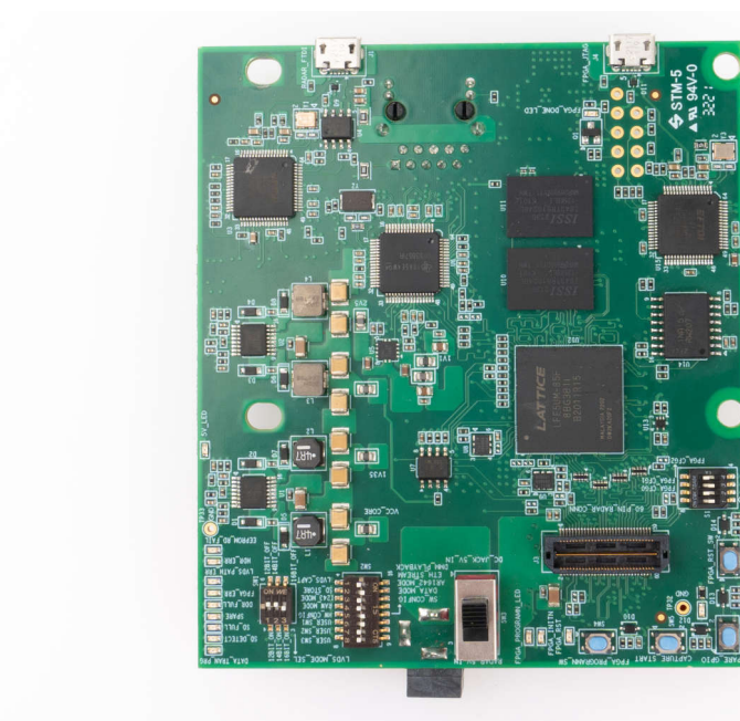
图 3-32. DCA1000 开关设置
