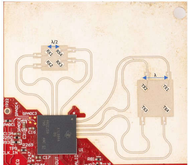
图 3-6. 关于 TX 和 RX 的天线虚拟阵列
