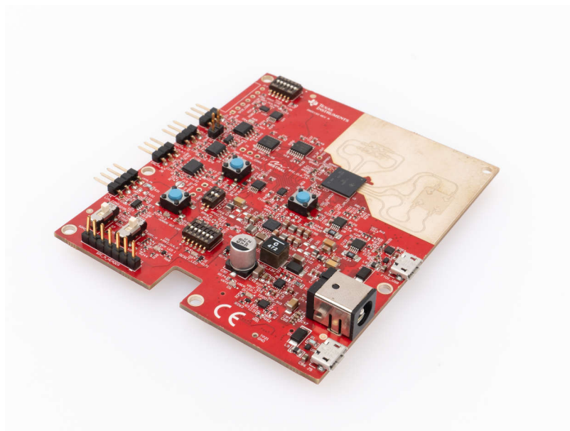
图 1-1. xWRL6844EVM
