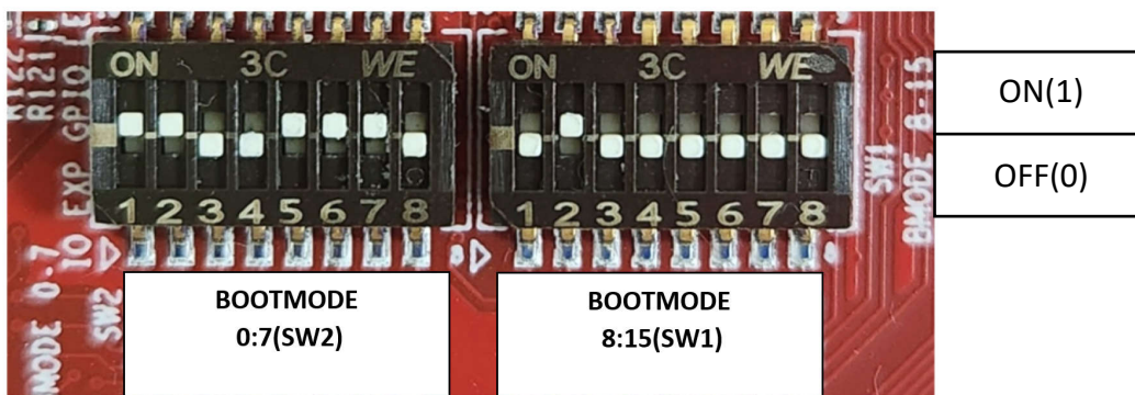
图 2-17. 引导模式开关 SW2 和 SW1 ( OSPI 引导 )
