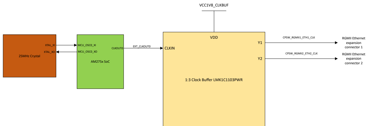
图 2-12. 晶体时钟树
