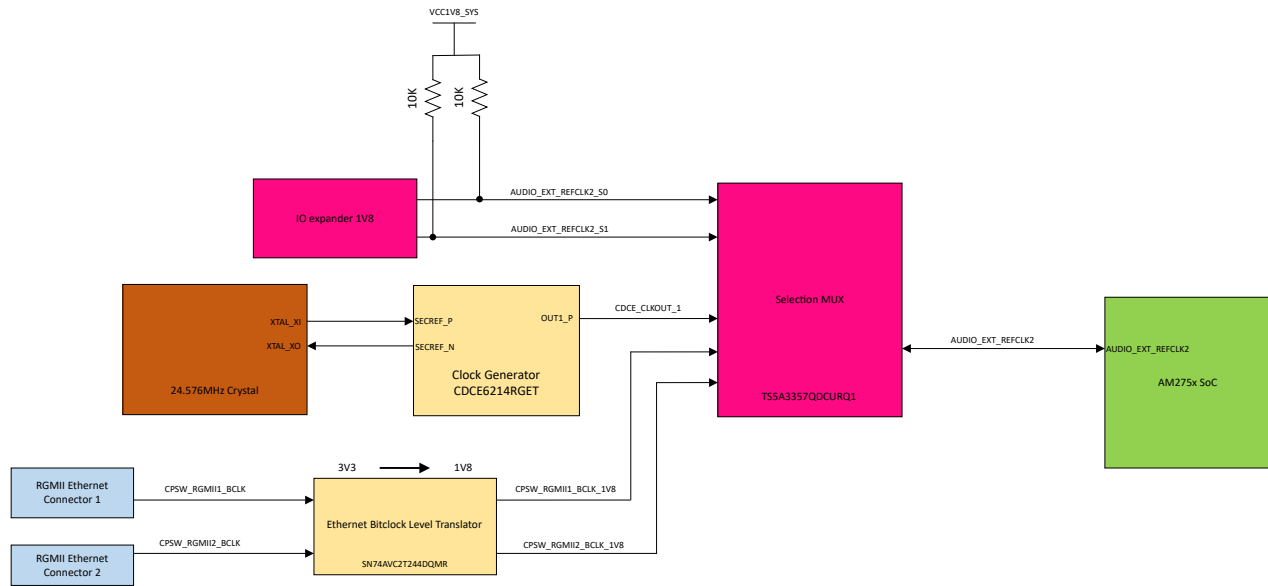
图 2-13. Audio_EXT_REFCLK2 时钟树
