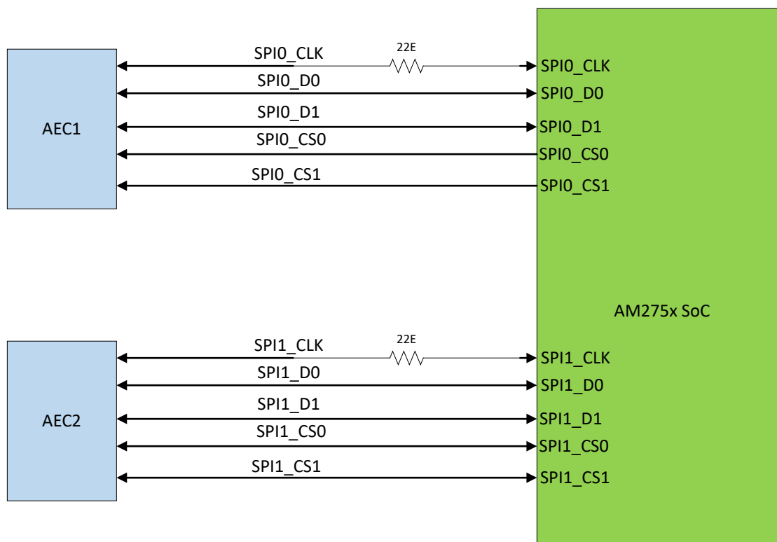
图 2-33. SPI 接口方框图
