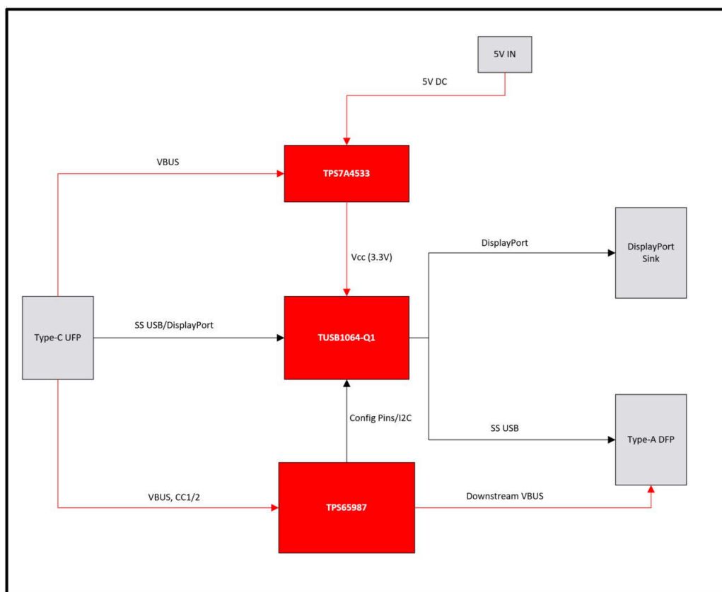
图 1-1. 方框图
