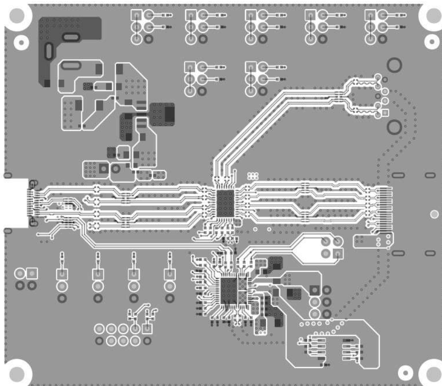
图 4-5. TUSB1064-Q1 EVM PCB 第 1 层 (顶部)
