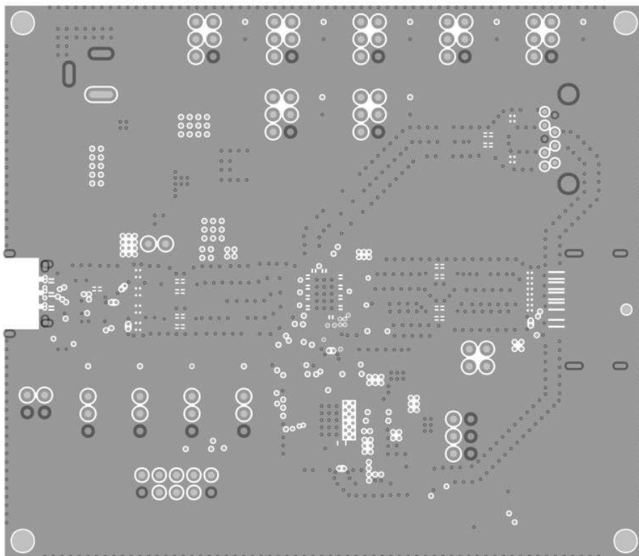
图 4-6. TUSB1064-Q1 EVM PCB 第 2 层 (GND)
