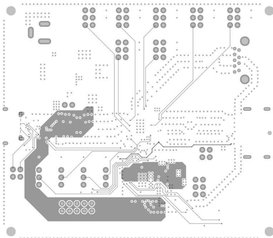
图 4-8. TUSB1064-Q1 EVM PCB 第 4 层 ( 信号 )
