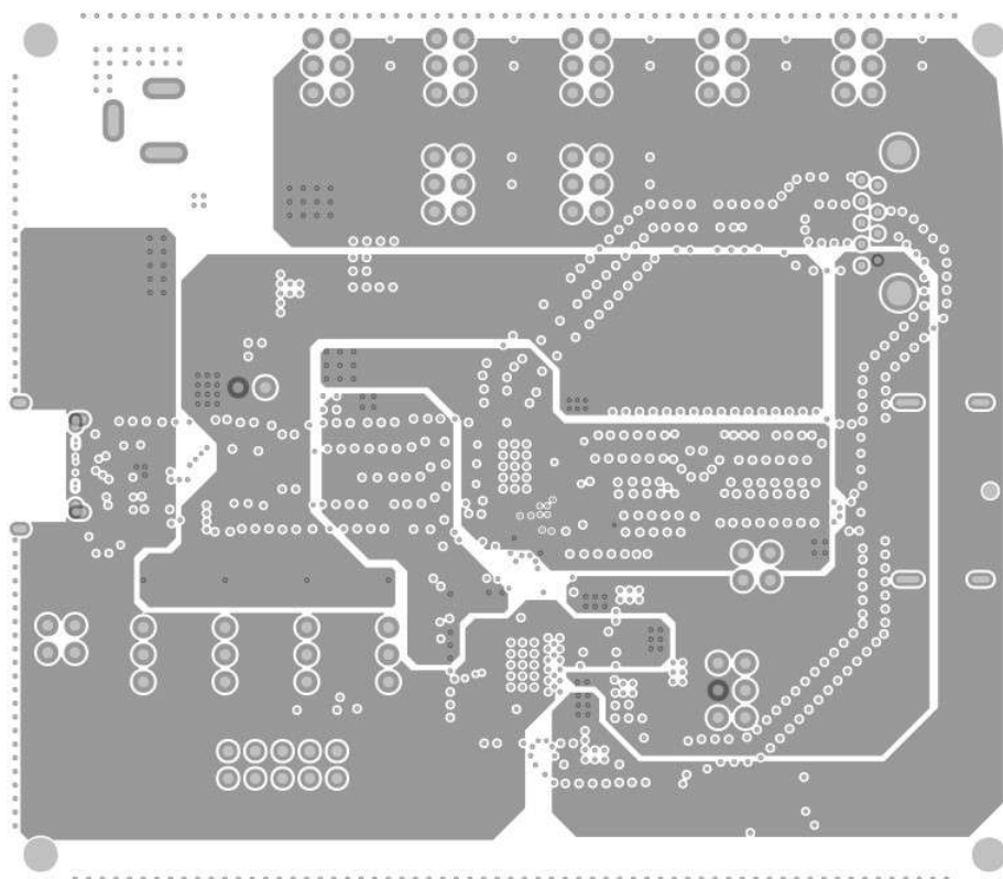
图 4-7. TUSB1064-Q1 EVM PCB 第 3 层 ( 电源 )
