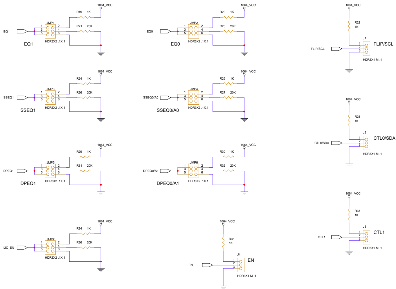
图 4-2. TUSB1064-Q1 EVM 原理图 (第 2 页)
