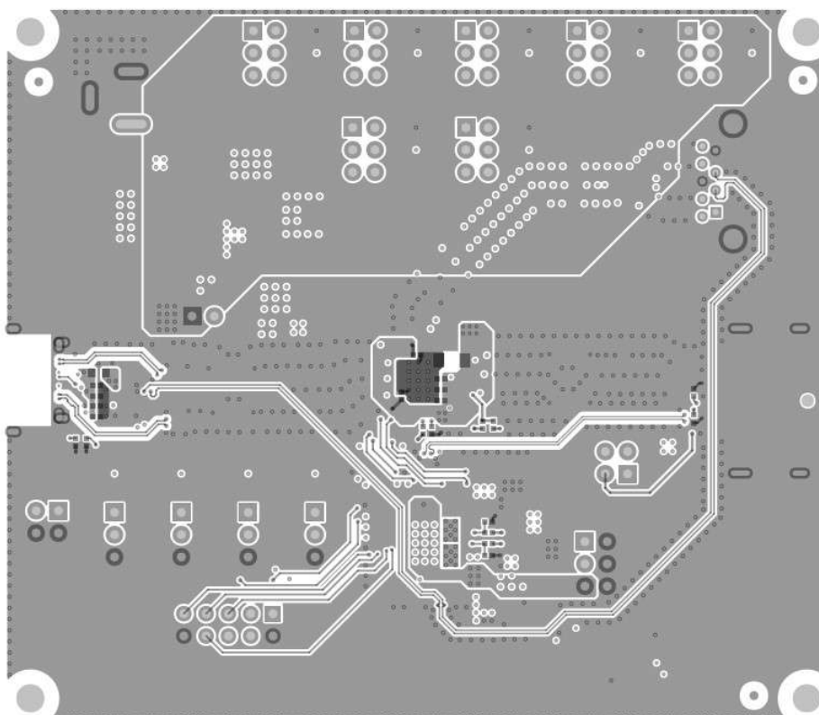
图 4-10. TUSB1064-Q1 EVM PCB 第 6 层 (底部)
