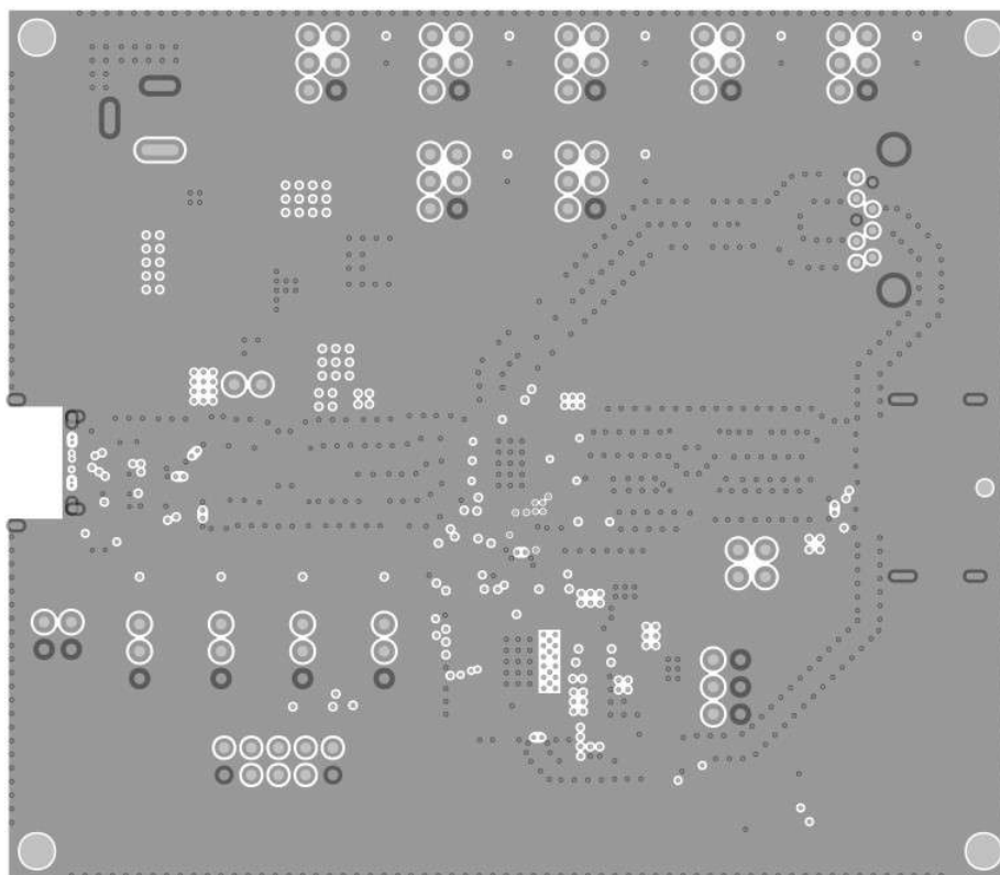
图 4-9. TUSB1064-Q1 EVM PCB 第 5 层 (GND)
