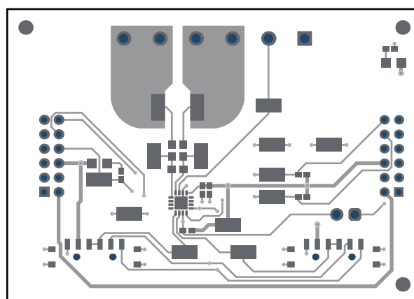
图 4-4. 顶层
