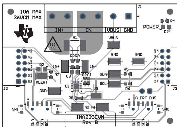
图 4-3. 顶视图
