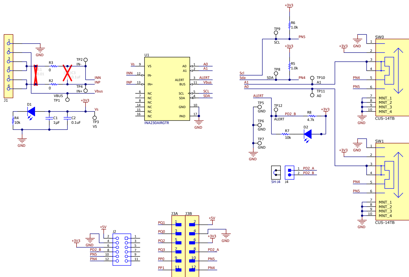
图 4-1. 原理图电路
