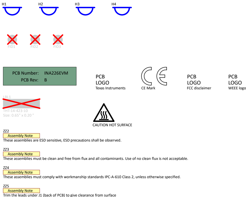
图 4-2. 硬件原理图
