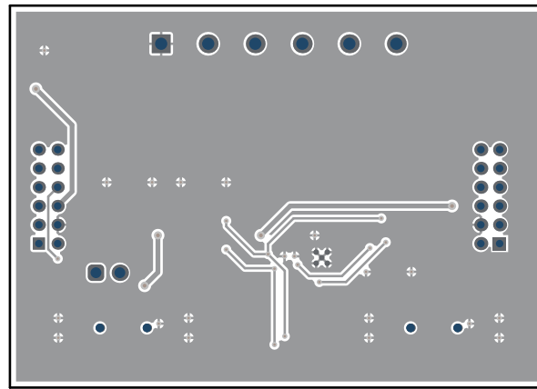
图 4-6. 底层
