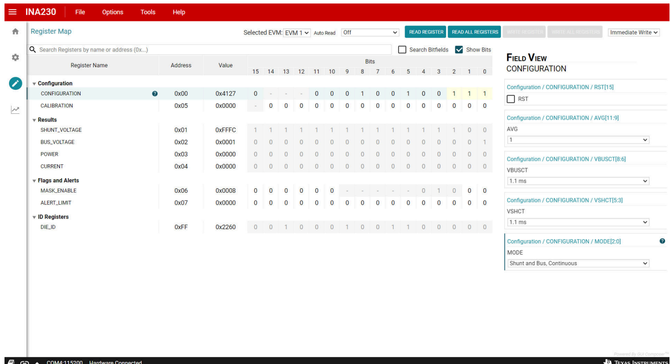
图 3-9. GUI 寄存器选项卡
