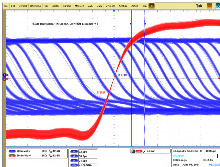
图 4-5. SYSREF 5 代码步长延迟
