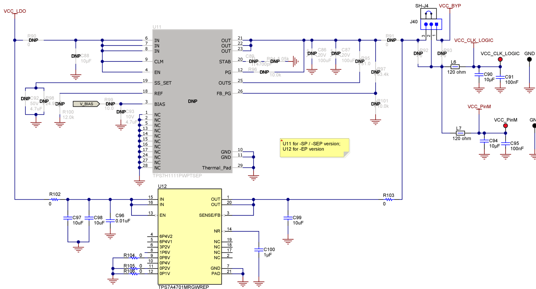
图 5-2. 电源
