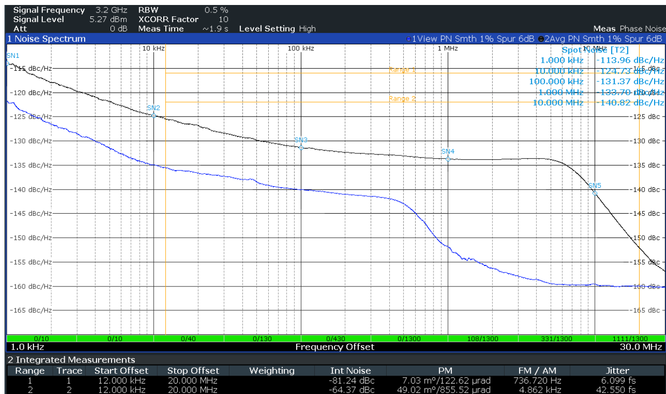
图 4-3. 4 倍频模式信号分析仪图
