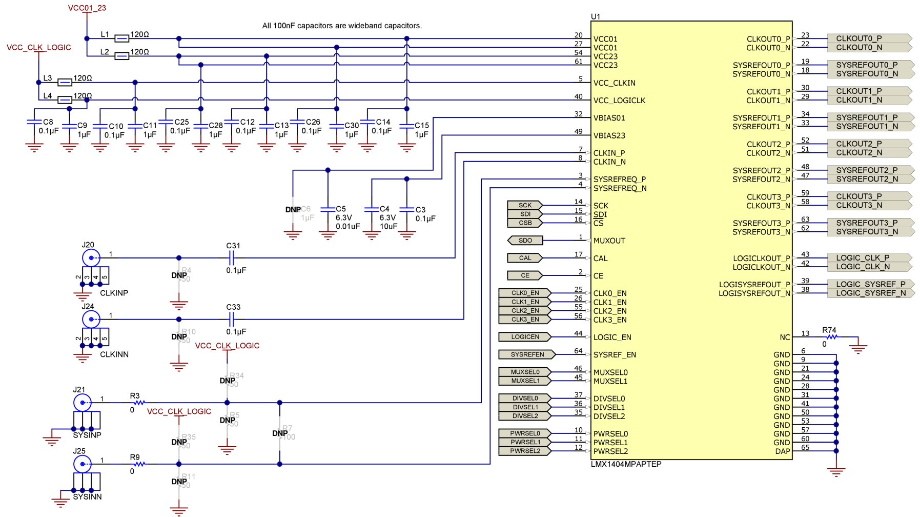
图 5-3. LMX1404-EP
