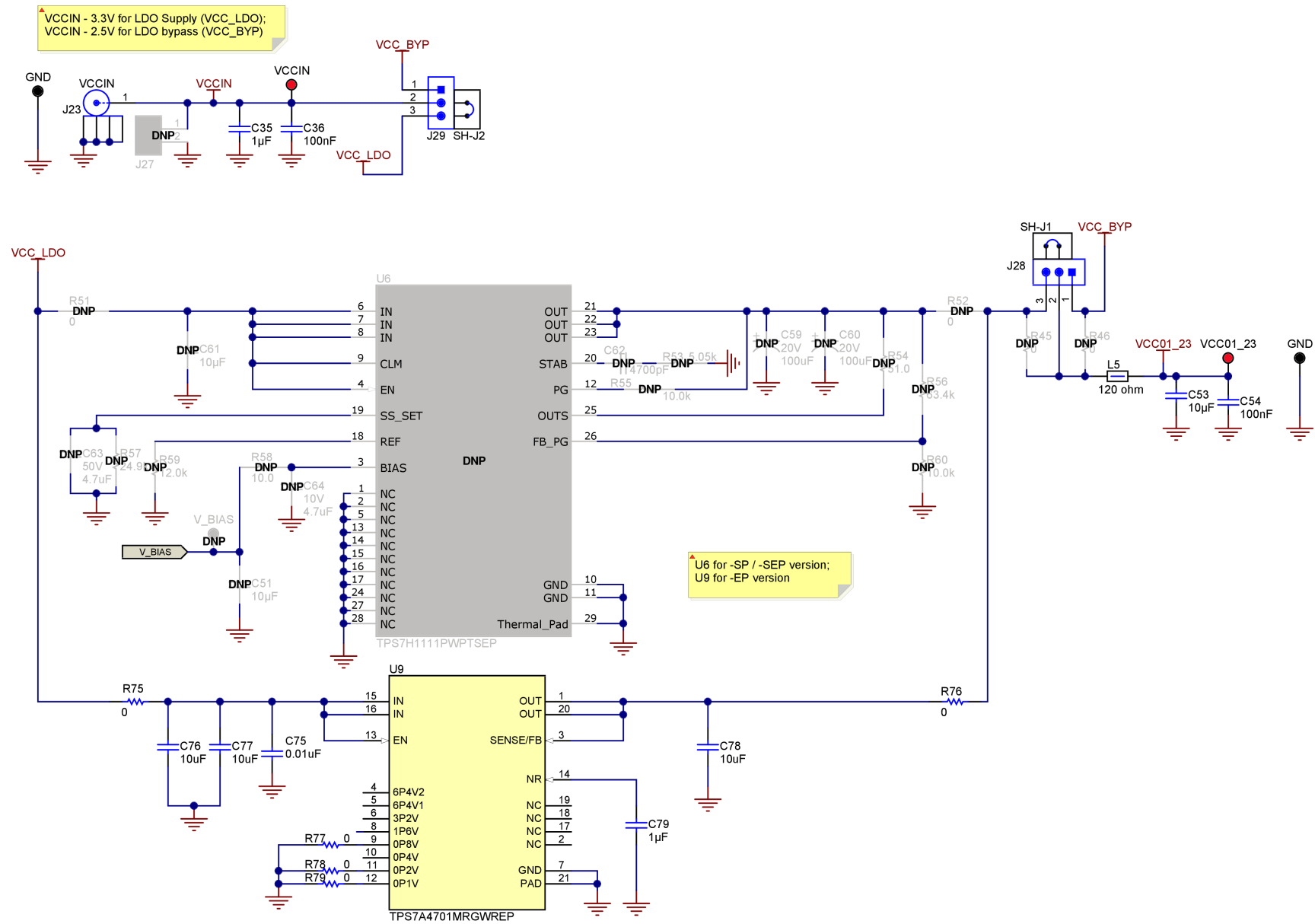
图 5-1. 电源
