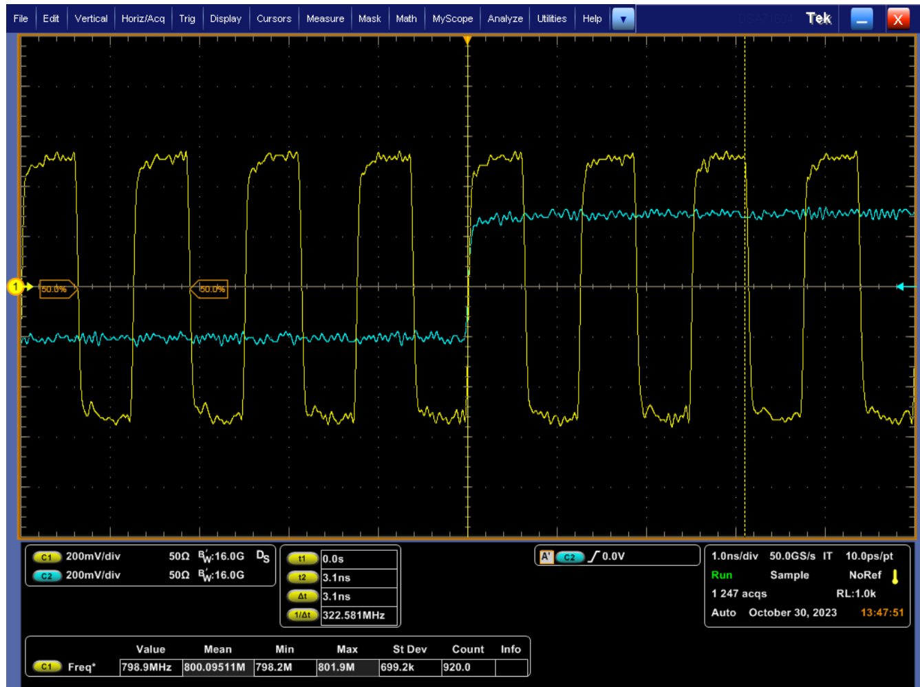
图 4-4. 具有 10MHz SYSREF 的缓冲器模式
