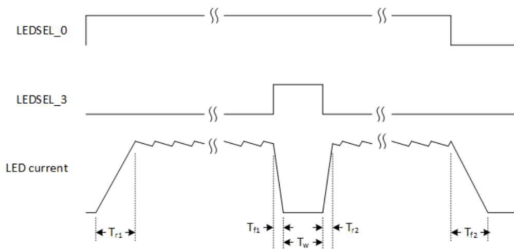
图 2-7. DLP4621-Q1 电子产品 EVM LED 驱动器板时序规格
