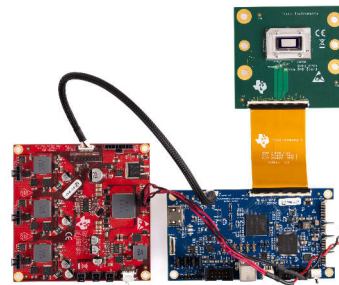
DLP4621Q1EVM
