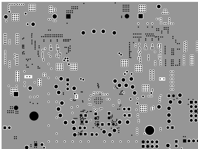
图 3-9. 第 5 层 — GND
