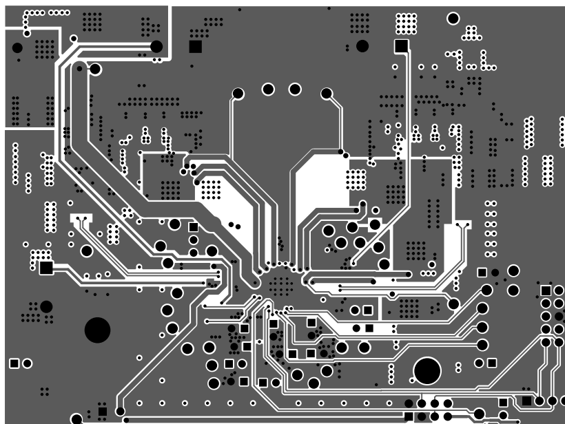
图 3-7. 信号层 1
