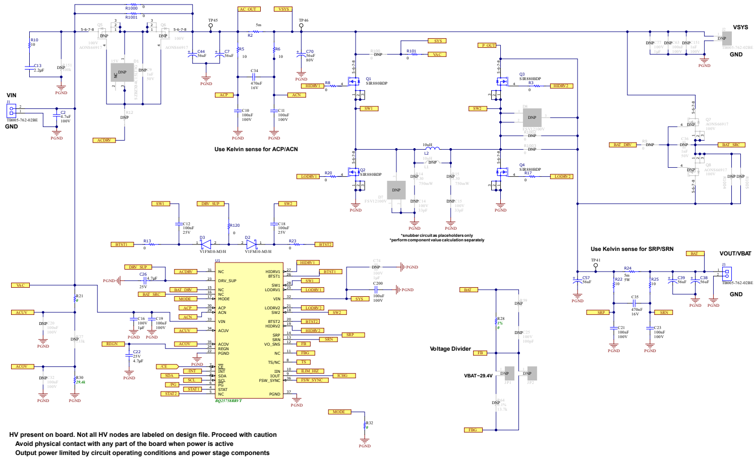
图 3-1. BQ25758 和 BQ25758A EVM 原理图 (第 1 页)
