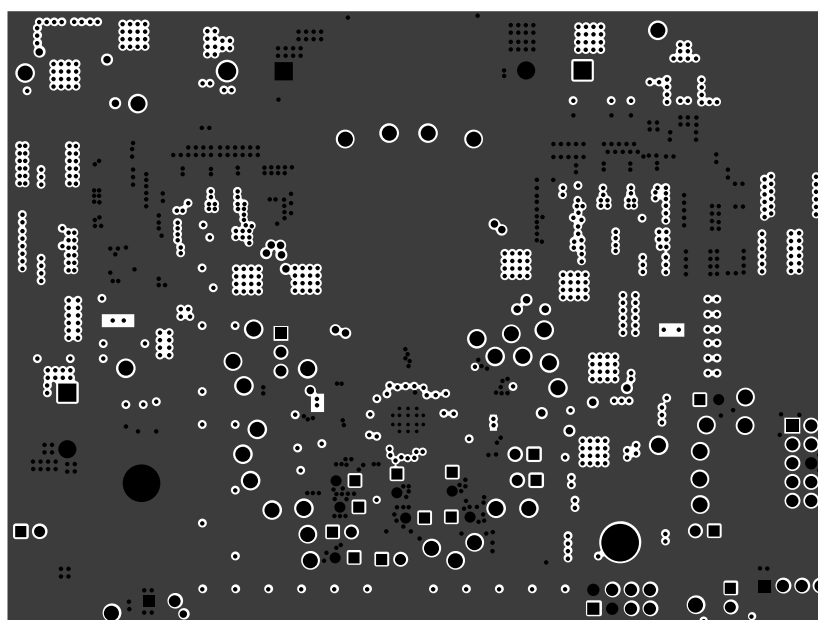
图 3-6. 第 2 层 — GND
