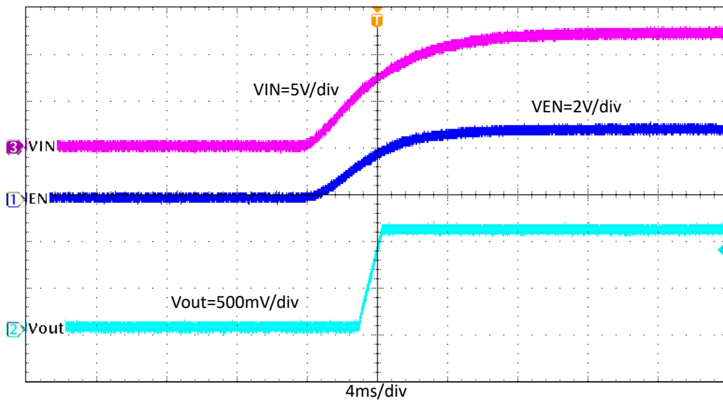
图 7-10. TPS562203EVM 相对于 V_{IN} 的启动
