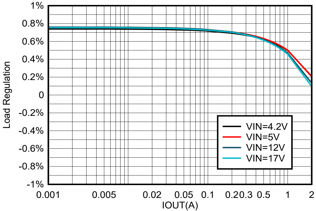
图 7-5. TPS562206EVM 负载调整率
