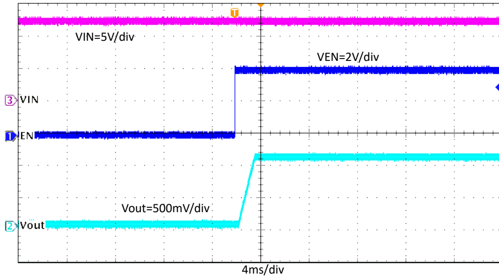
图 7-11. TPS562203EVM 相对于 EN 的启动
