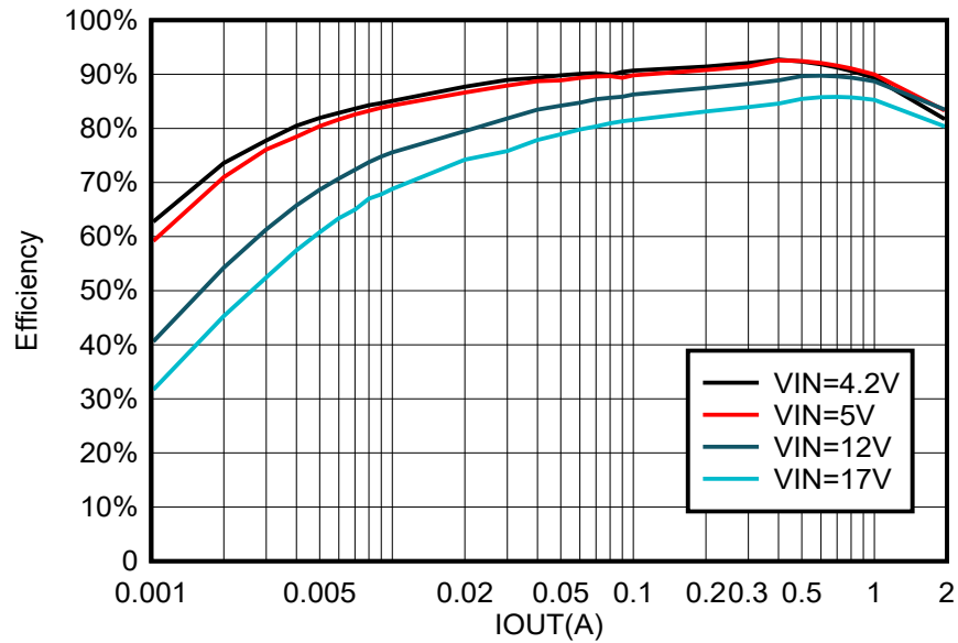
图 7-2. TPS562203EVM 效率
