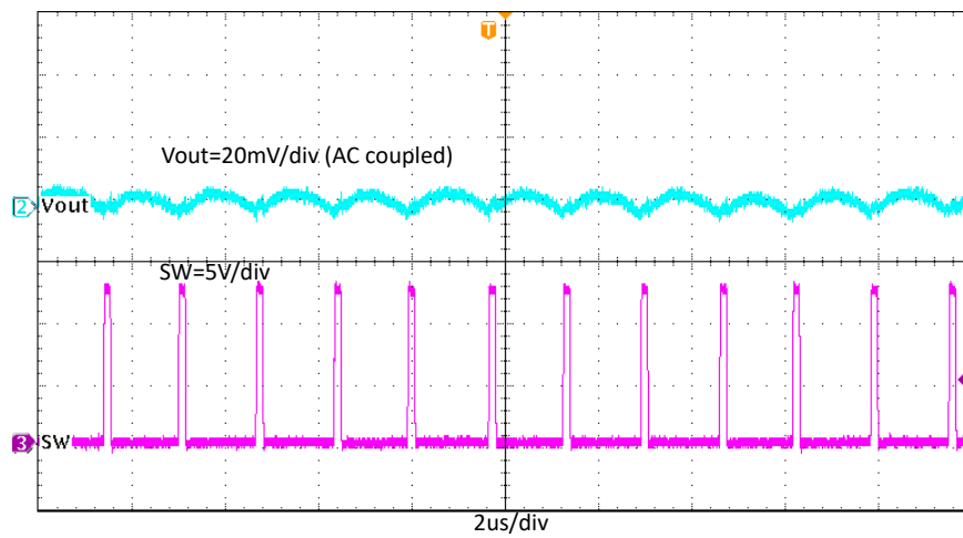
图 7-16. TPS562206EVM 输出电压纹波, I_{OUT} = 0.01A
