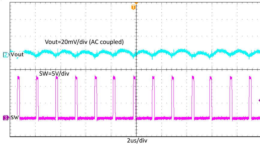
图 7-14. TPS562203EVM 输出电压纹波， I_{OUT} = 2A
