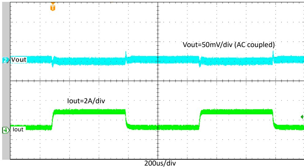
图 7-9. TPS562206EVM 负载瞬态响应，10% 至 90% ( 0.2A 至 1.8A ) 负载阶跃
