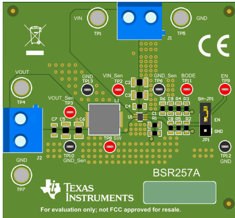
图 7-1. TPS562203EVM 连接器和跳线布置
