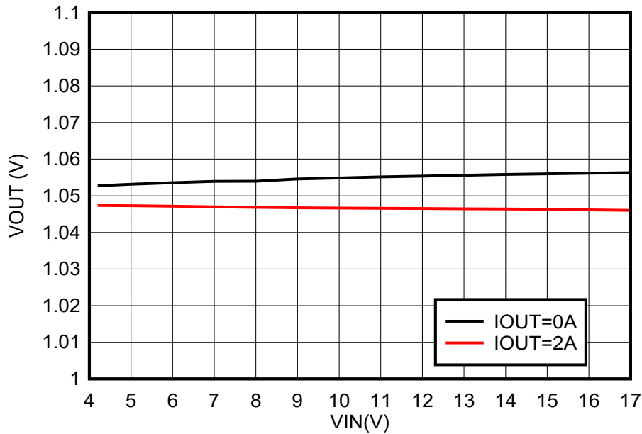
图 7-6. TPS562203EVM 线性调整率
