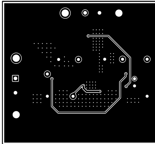
图 8-4. TPS562203EVM 底层
