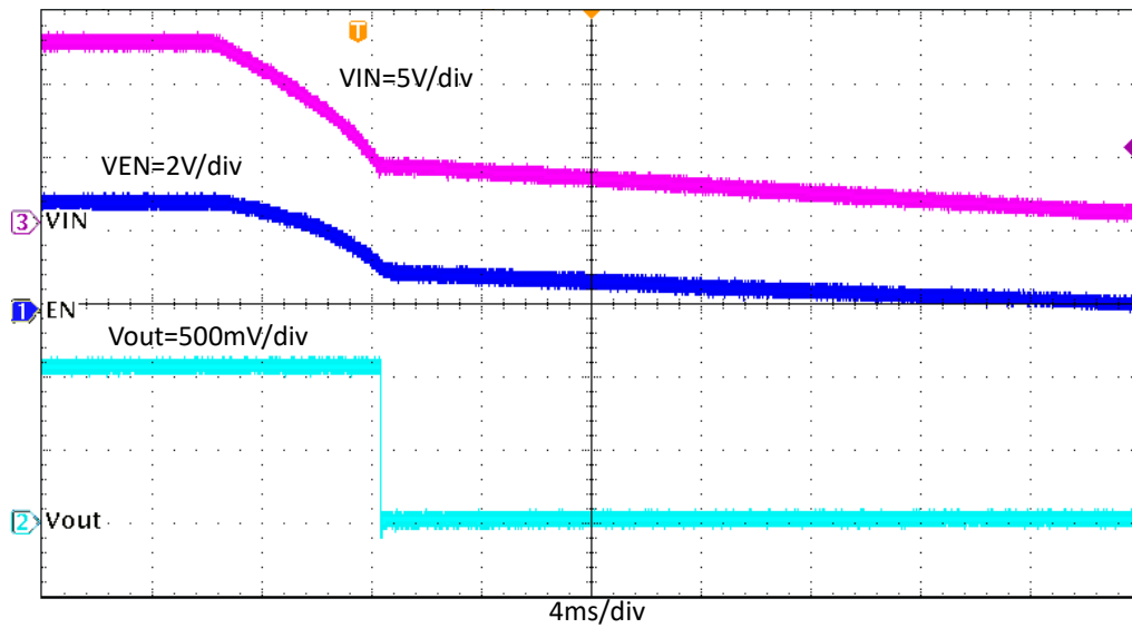
图 7-12. TPS562203EVM 相对于 V_{IN} 的关断
