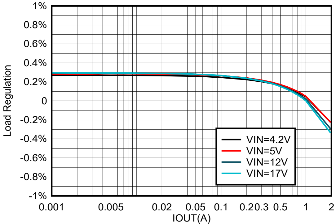
图 7-4. TPS562203EVM 负载调整率
