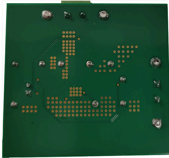
图 8-6. TPS562203EVM 电路板 (底视图)
