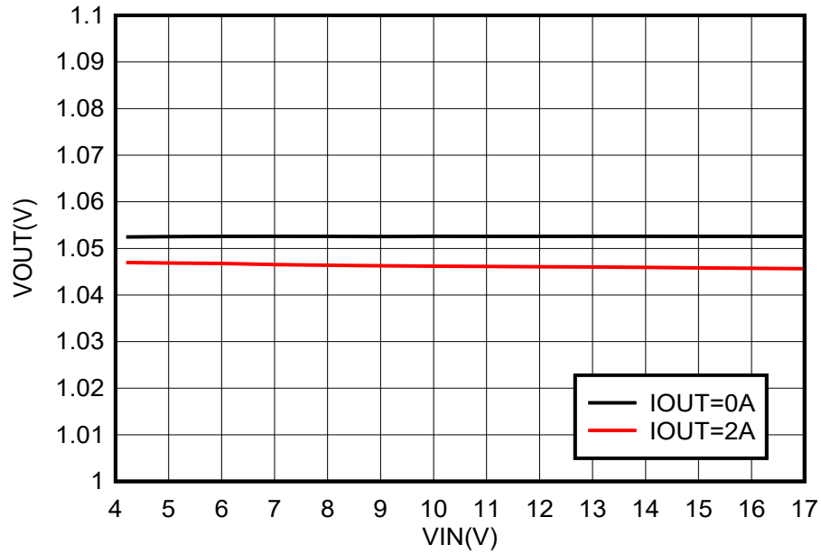
图 7-7. TPS562206EVM 线性调整率
