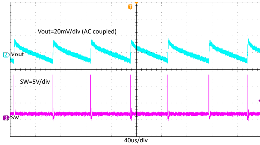
图 7-15. TPS562203EVM 输出电压纹波, I_{OUT} = 0.01A
