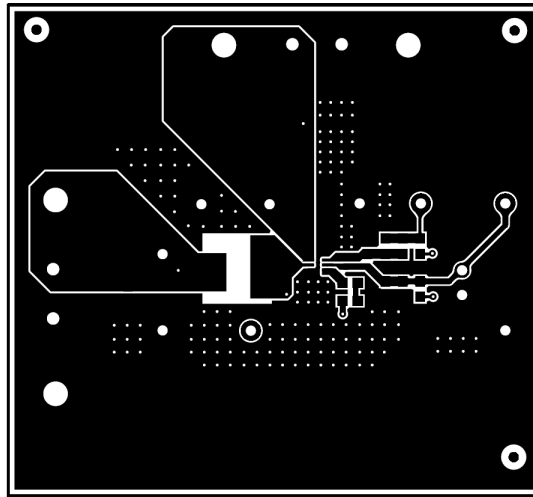
图 8-3. TPS562203EVM 顶层
