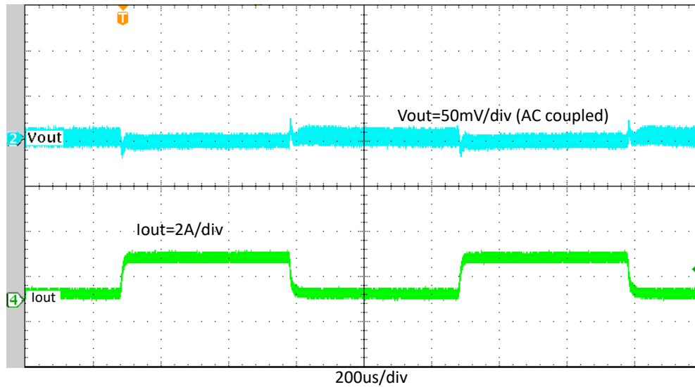
图 7-8. TPS562203EVM 负载瞬态响应，10% 至 90% ( 0.2A 至 1.8A ) 负载阶跃
