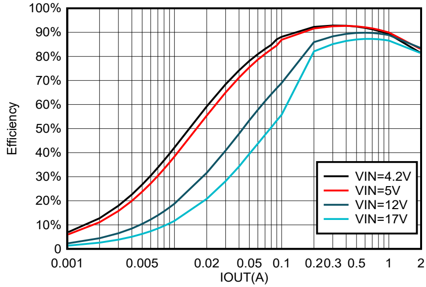
图 7-3. TPS562206EVM 效率
