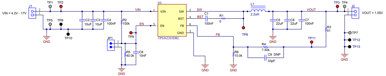
图 8-1. TPS562203EVM 原理图
