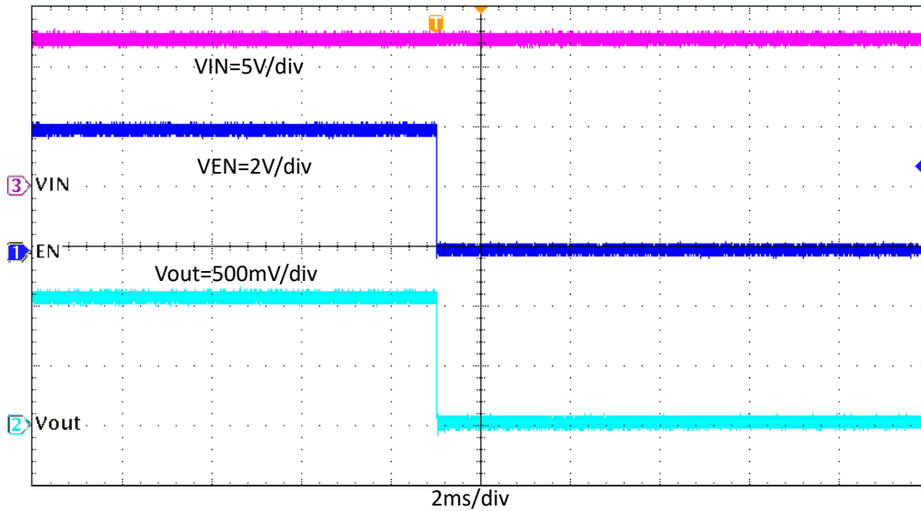
图 7-13. TPS562203EVM 相对于 EN 的关断
