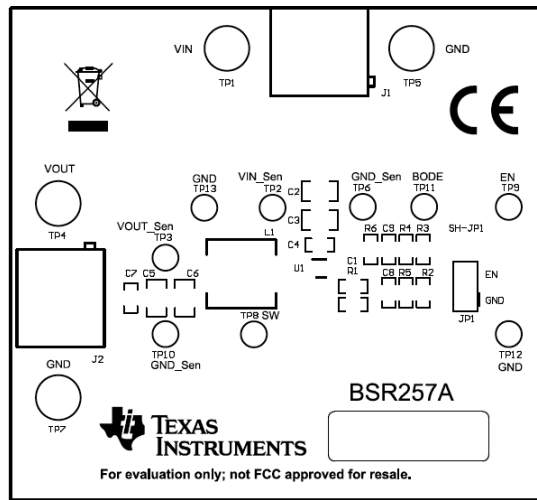
图 8-2. TPS562203EVM 顶层装配图
