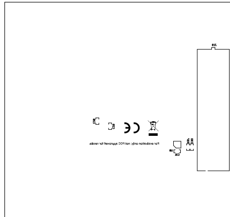
图 4-12. 底层丝印层
