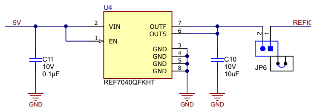
图 2-3. REF7040
