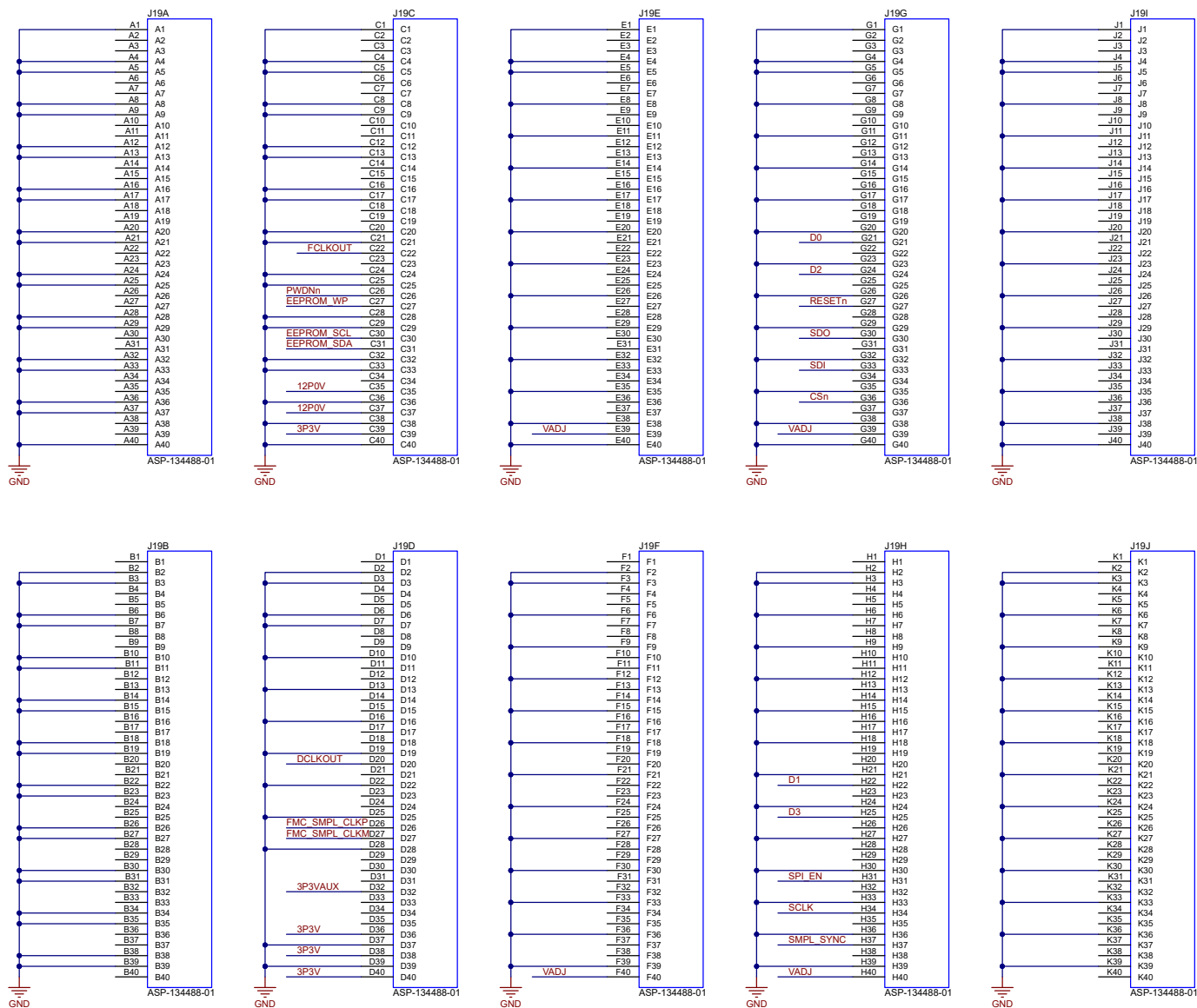
图 4-6. 数字连接器原理图
