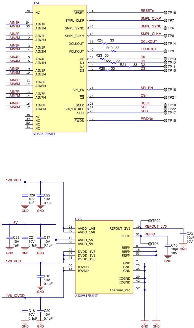
图 2-5. 与 ADS9817 的连接
