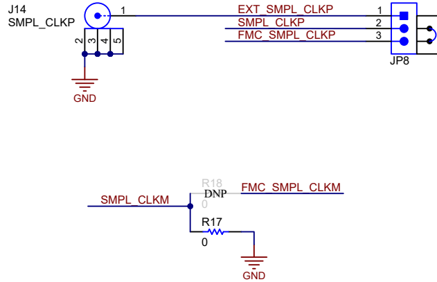
图 2-6. 采样时钟选择
