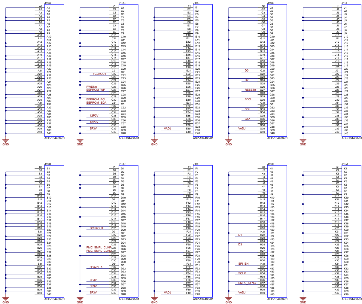
图 2-4. 数字 I/O
