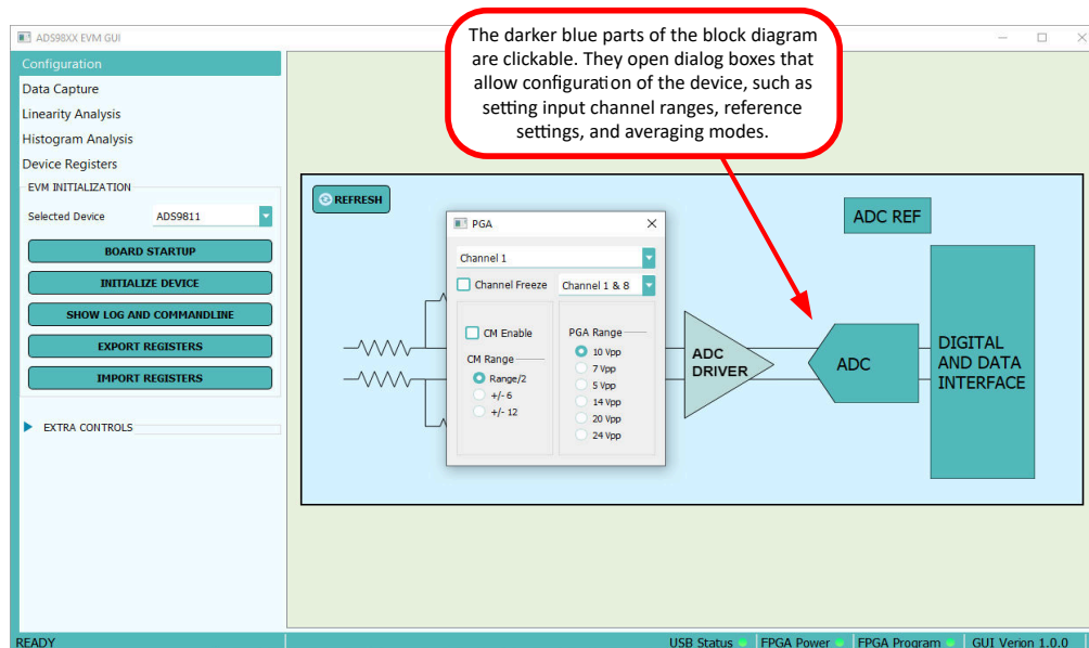
图 3-10. GUI 方框图
