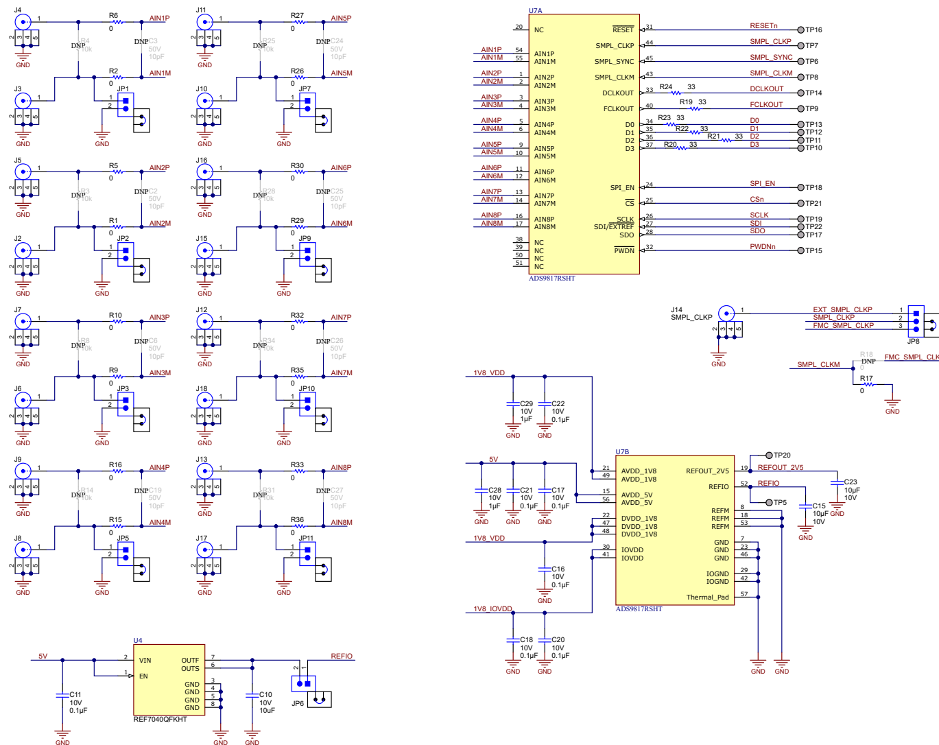
图 4-4. ADS9817 器件连接原理图
