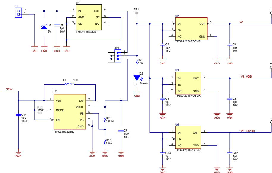
图 2-7. 电源输入和稳压器
