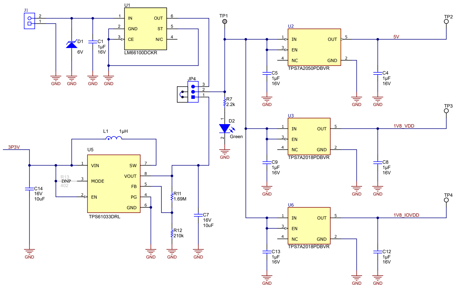
图 4-2. 电源连接和稳压器原理图
