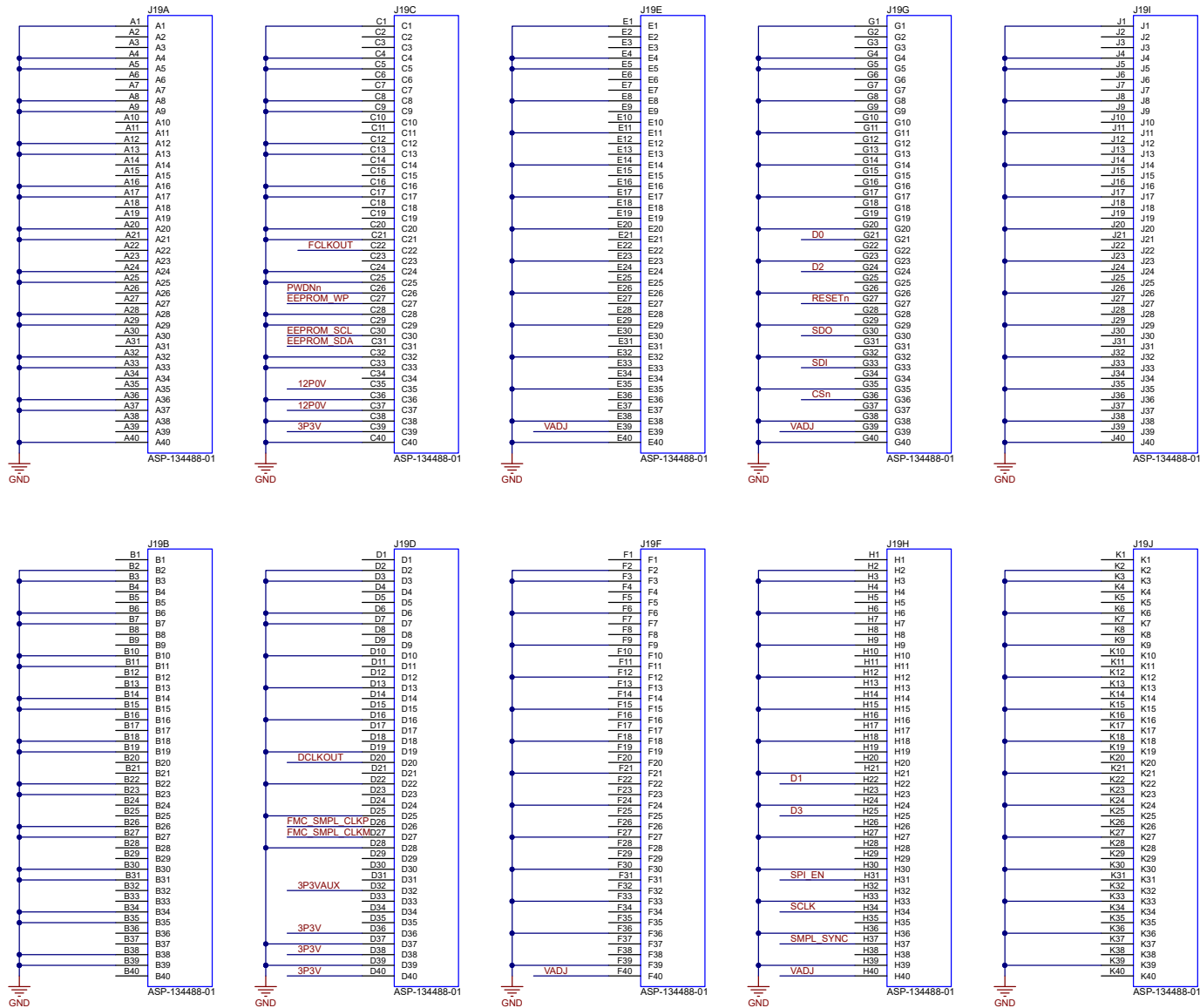
图 4-3. 数字连接器原理图
