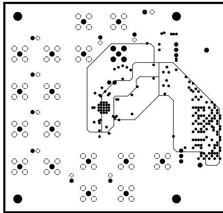
图 4-10. GND2 层
