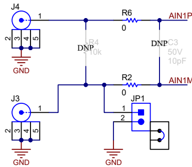
图 2-2. 输入 SMA 连接数字接口
