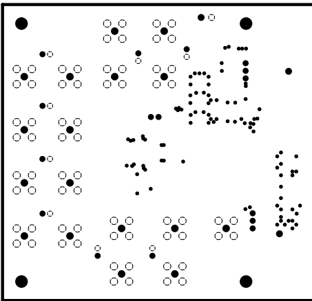
图 4-9. GND1 层
