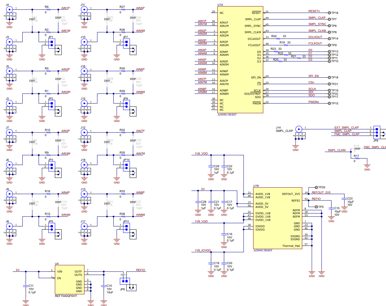
图 4-1. ADS9813 器件连接原理图
