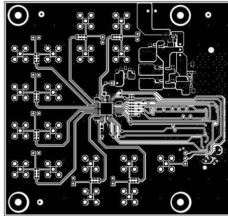
图 4-8. 顶层
