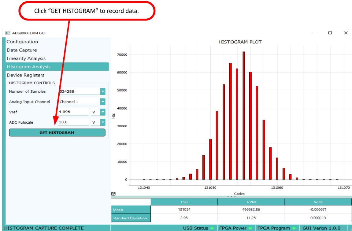
图 3-14. 直方图数据
