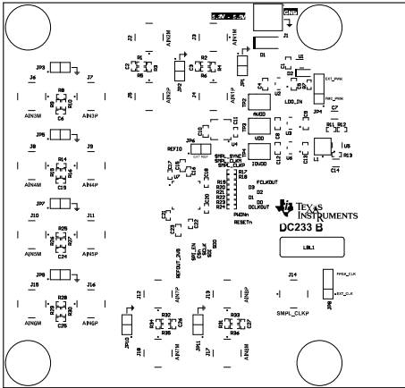
图 4-7. 顶层丝印层
