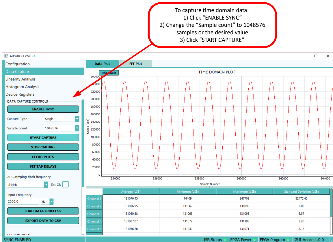
图 3-11. 时域数据
