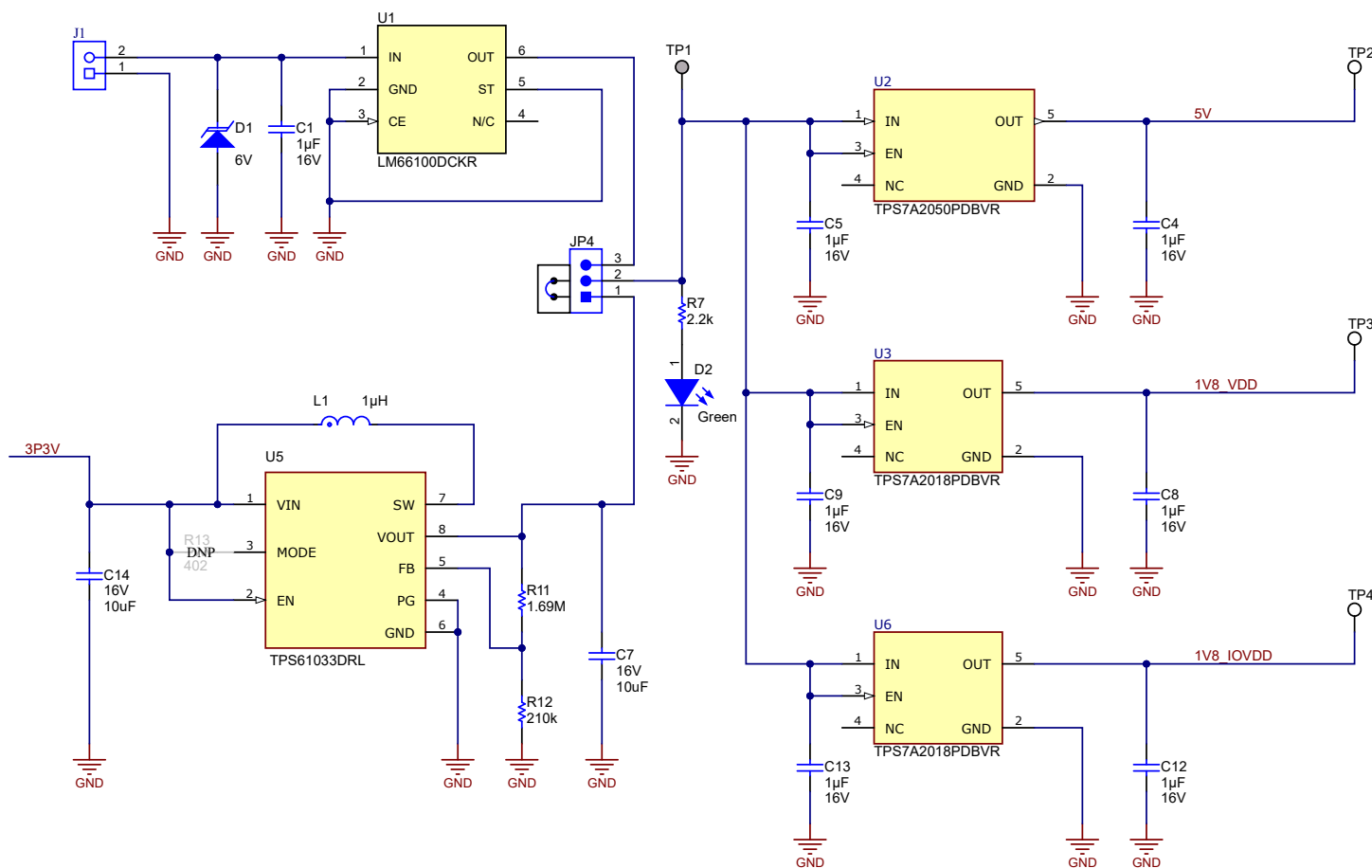
图 4-5. 电源连接和稳压器原理图
