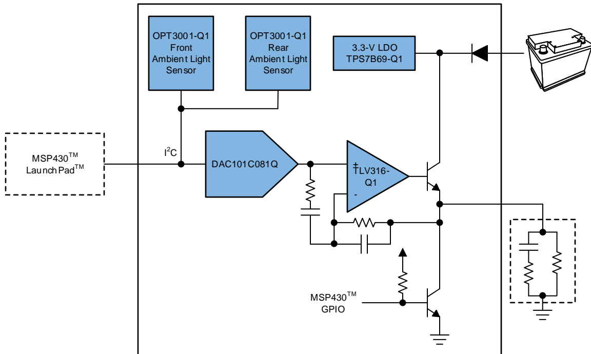
图 1. TIDA-01359 Block Diagram
