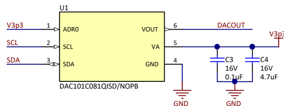
图 7. DAC Schematic
