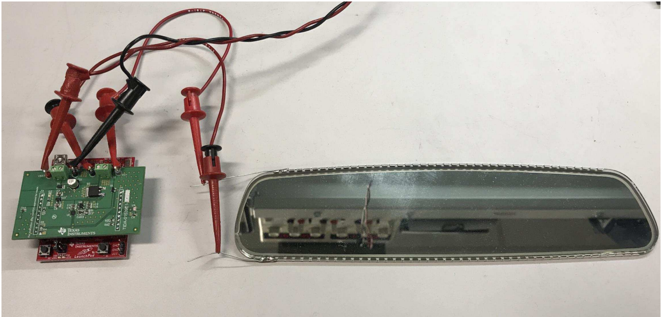
图 14. TIDA-01539 Test Setup
