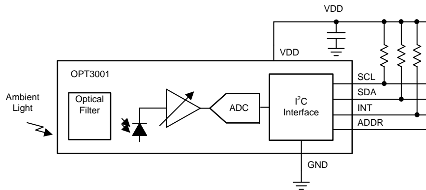
图 2. OPT3001-Q1 Block Diagram
