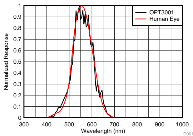
图 3. OPT3001-Q1 Spectral Response
